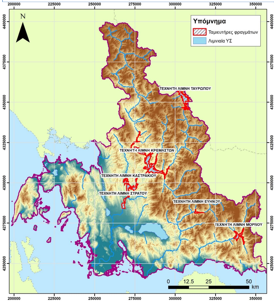
Χάρτης 6-1: Χάρτης φραγμάτων στο EL04
