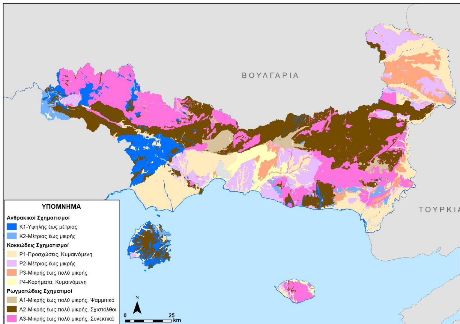
Εικόνα 4-1 Υδρολιθολογικός Χάρτης ΥΔ Θράκης (EL12)
