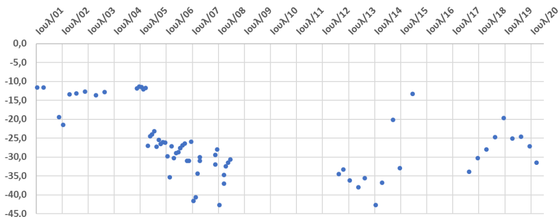
Απόλυτη Στάθμη (m) - EL12051202
