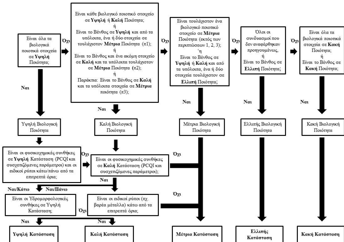
Σχήμα 5.3.1-5: Λογικό διάγραμμα ή δένδρο απόφασης για την συνθετική εκτίμηση της οικολογικής ποιότητας σε μεταβατικά και παράκτια ΥΣ (Borja et al., 2009, τροπ. από Simboura et al, 2016)
