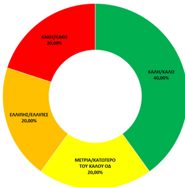
Σχήμα 8.3.1-1: Συνολικός αριθμός (%) λιμναίων ΥΣ ανά κατηγορία οικολογικής κατάστασης – δυναμικού στο ΥΔ Δυτικής Στερεάς Ελλάδας (EL04)
