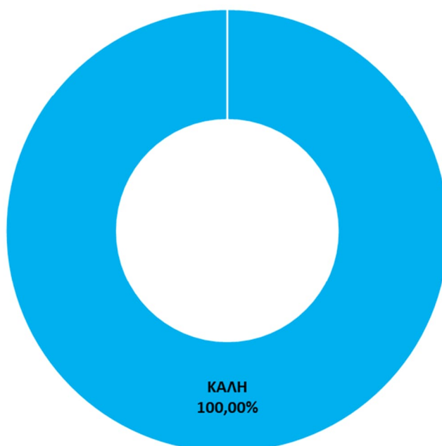
Σχήμα 8.5.2-2: Συνολική επιφάνεια (%) παράκτιων ΥΣ ανά κατηγορία χημικής κατάστασης στο ΥΔ Δυτικής Στερεάς Ελλάδας (EL04)
