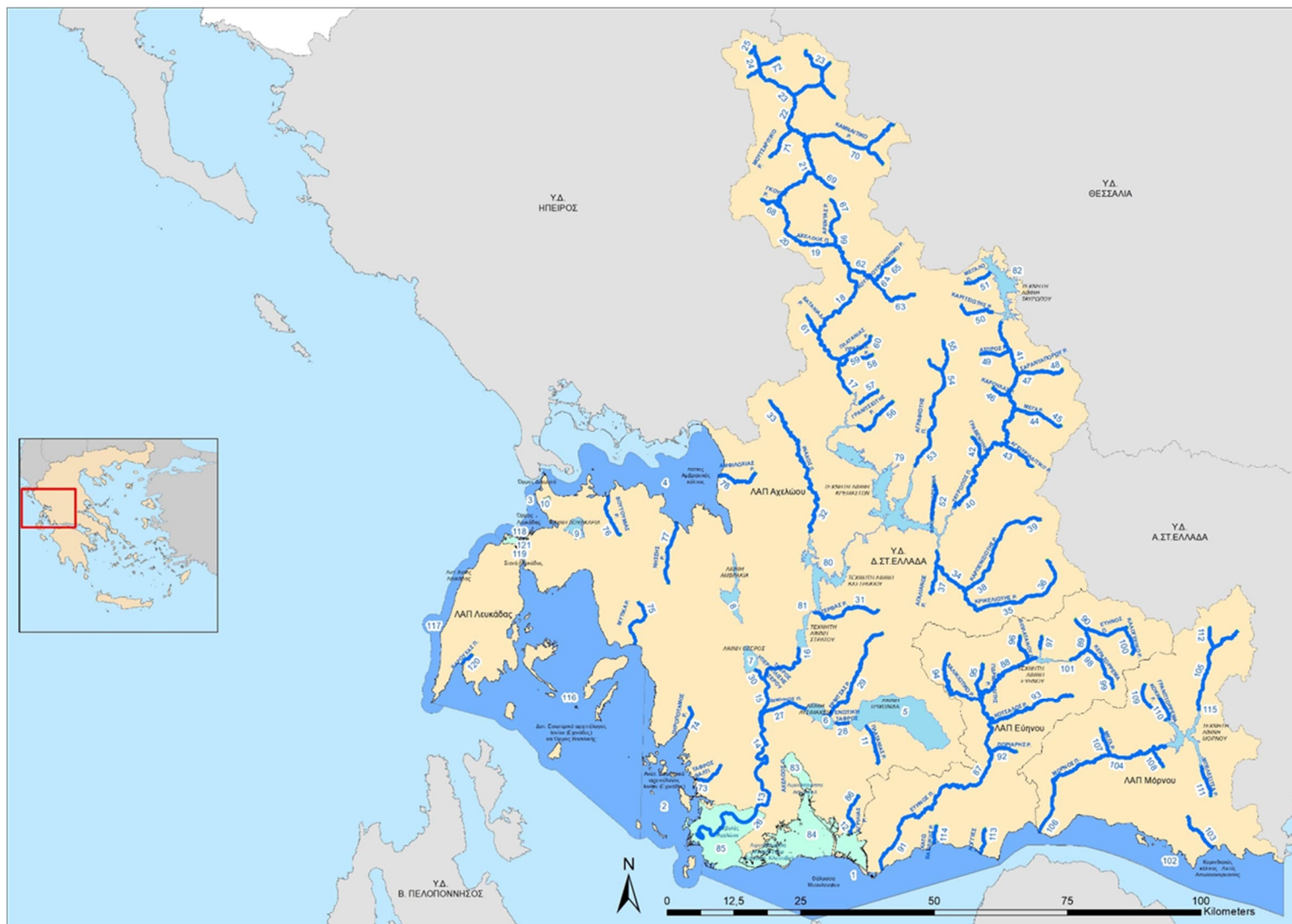
Χάρτης 4-1: Χάρτης επιφανειακών ΥΣ ΥΔ Δυτικής Στερεάς Ελλάδας (EL04)
