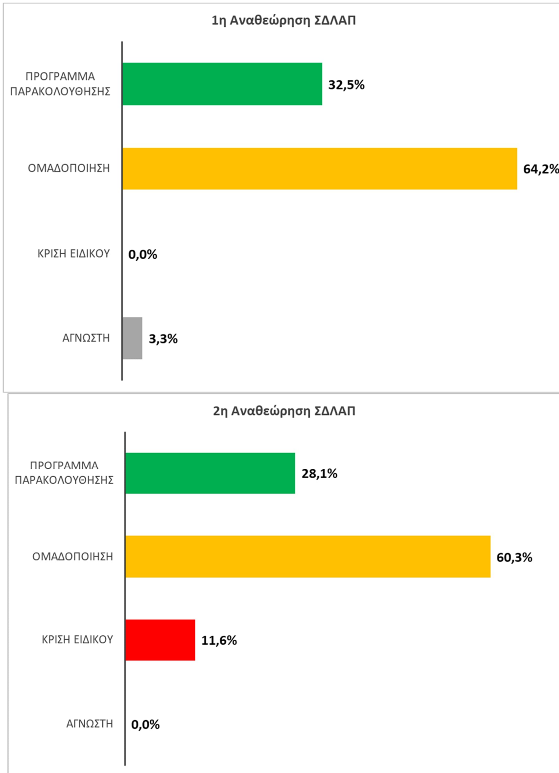
Σχήμα 8.6-4: Μέθοδος και επίπεδο εμπιστοσύνης ταξινόμησης της χημικής κατάστασης των επιφανειακών υδατικών συστημάτων στο ΥΔ Δυτικής Στερεάς Ελλάδας (EL04) σε σύγκριση με την εγκεκριμένη 1 η Αναθεώρηση των ΣΔΛΑΠ
