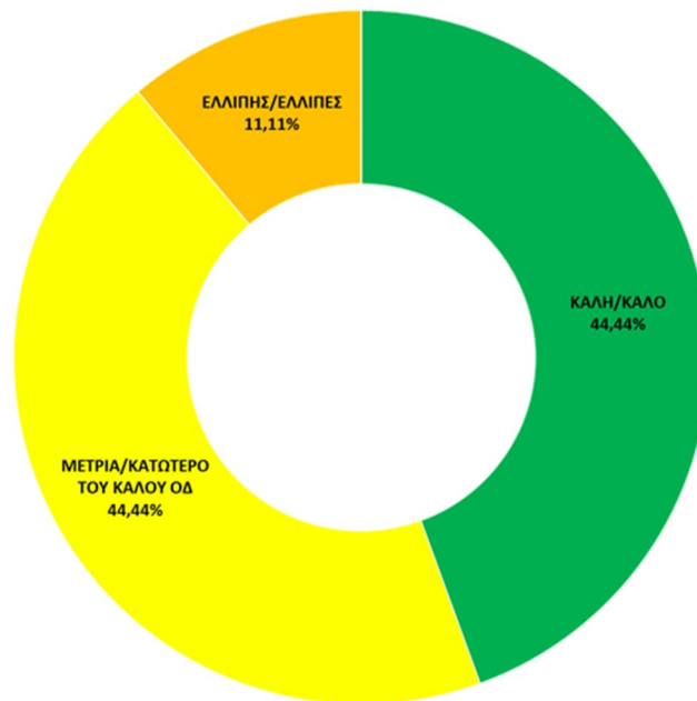
Σχήμα 8.5.1-1: Συνολικός αριθμός (%) παράκτιων ΥΣ ανά κατηγορία οικολογικής κατάστασης – δυναμικού στο ΥΔ Δυτικής Στερεάς Ελλάδας (EL04)
