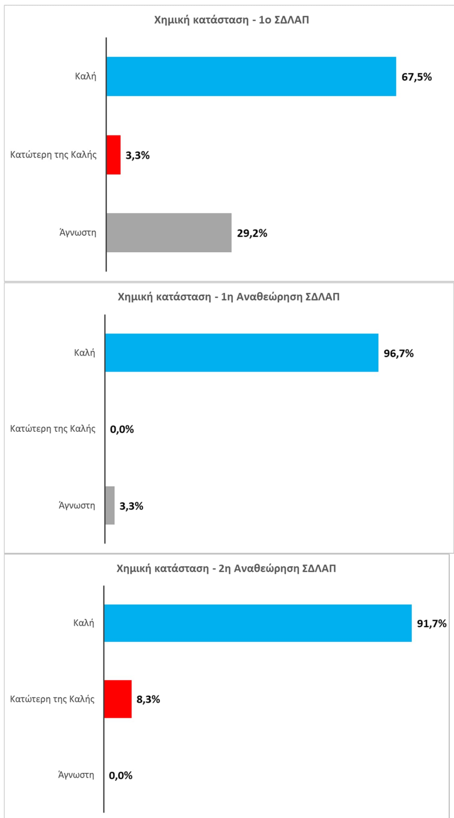
Σχήμα 8.6-3: Αποτελέσματα ταξινόμησης χημικής κατάστασης επιφανειακών υδατικών συστημάτων στο ΥΔ Δυτικής Στερεάς Ελλάδας (EL04) σε σύγκριση με τα προηγούμενα εγκεκριμένα ΣΔΛΑΠ.
