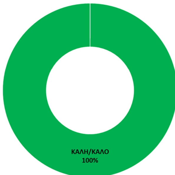
Σχήμα 8.3.2-2: Συνολική επιφάνεια (%) ποτάμιων ΙΤΥΣ λιμναίου χαρακτήρα (ταμιευτήρων) ανά κατηγορία οικολογικής κατάστασης – δυναμικού στο ΥΔ Δυτικής Στερεάς Ελλάδας (EL04).
