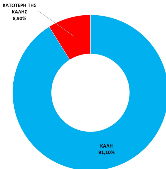
Σχήμα 8.2.2-2: Συνολικό μήκος (%) ποτάμιων υδατικών συστημάτων ανά κατηγορία χημικής κατάστασης στο ΥΔ Δυτ. Στερεάς Ελλάδας (EL04)
