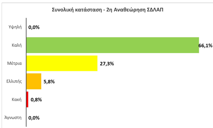
Σχήμα 8.6-5: Αποτελέσματα ταξινόμηση συνολικής κατάστασης επιφανειακών υδατικών συστημάτων στο ΥΔ Δυτικής Στερεάς Ελλάδας (EL04) σε σύγκριση με τα προηγούμενα εγκεκριμένα ΣΔΛΑΠ.
