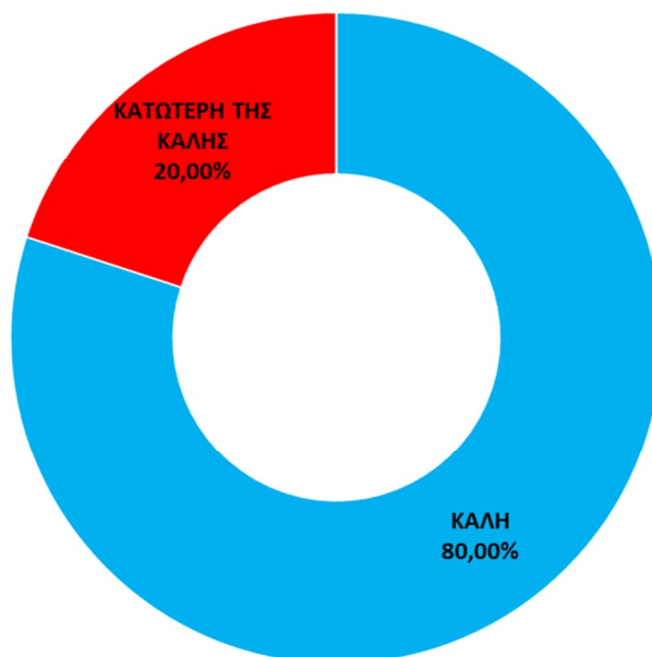
Σχήμα 8.4.2-1: Συνολικός αριθμός (%) μεταβατικών ΥΣ ανά κατηγορία χημικής κατάστασης στο ΥΔ Δυτικής Στερεάς Ελλάδας (EL04)
