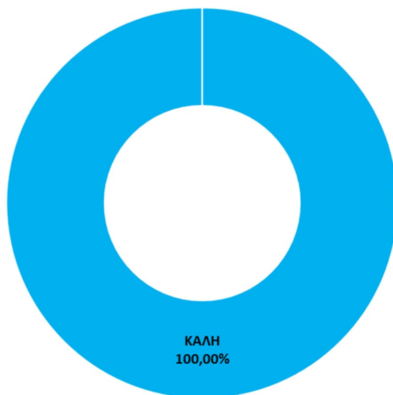
Σχήμα 8.5.2-1: Συνολικός αριθμός (%) παράκτιων ΥΣ ανά κατηγορία χημικής κατάστασης στο ΥΔ Δυτικής Στερεάς Ελλάδας (EL04)
