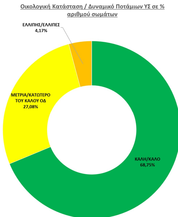
Σχήμα 8.2.1-1: Συνολικός αριθμός (%) ποτάμιων υδατικών συστημάτων ανά κατηγορία οικολογικής κατάστασης – δυναμικού στο ΥΔ Δυτικής Στερεάς Ελλάδας (EL04)
