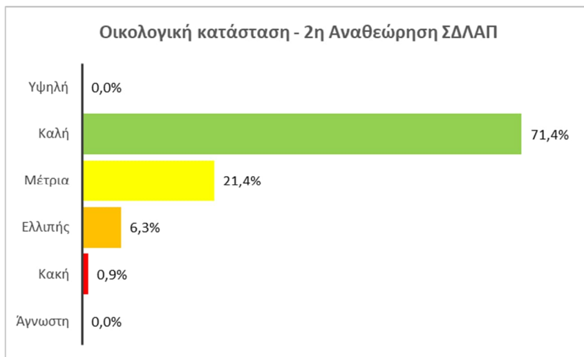
Σχήμα 8.6-1: Αποτελέσματα ταξινόμησης οικολογικής κατάστασης επιφανειακών υδατικών συστημάτων στο ΥΔ Δυτικής Στερεάς Ελλάδας (EL04) σε σύγκριση με τα προηγούμενα εγκεκριμένα ΣΔΛΑΠ (δεν συμπεριλαμβάνονται τα ΙΤΥΣ/ΤΥΣ, εκτός των ταμιευτήρων)
