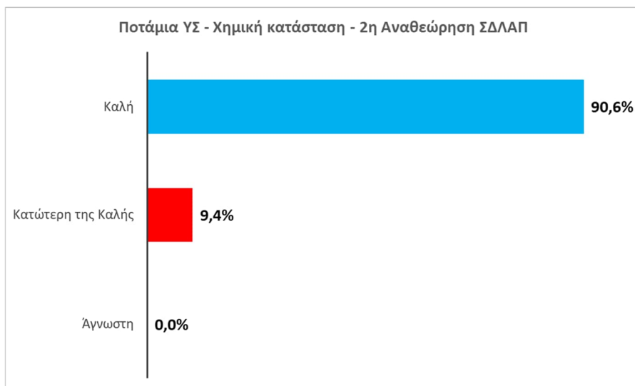
Σχήμα 8.2.2-3: Ταξινόμηση χημικής κατάστασης ποτάμιων υδατικών συστημάτων στο ΥΔ Δυτικής Στερεάς Ελλάδας (EL04) σε σύγκριση με τα προηγούμενα εγκεκριμένα ΣΔΛΑΠ
