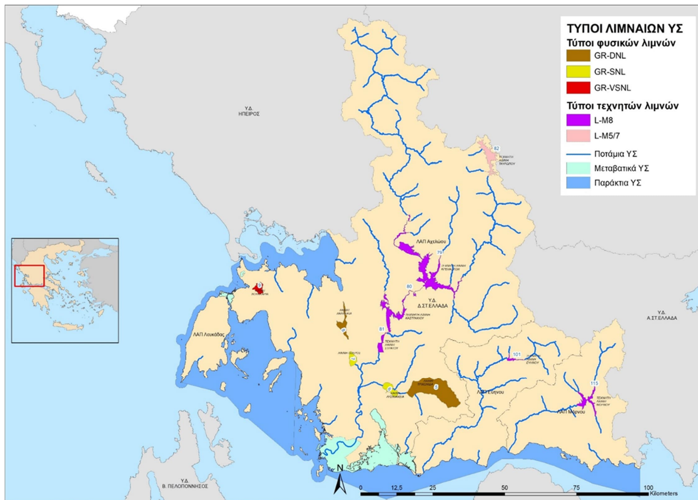
Χάρτης 4-3: Χάρτης τυπολογίας ποτάμινων ΙΤΥΣ λιμναίου χαρακτήρα και λιμναίων ΥΣ ΥΔ Δυτικής Στερεάς Ελλάδας (EL04)
