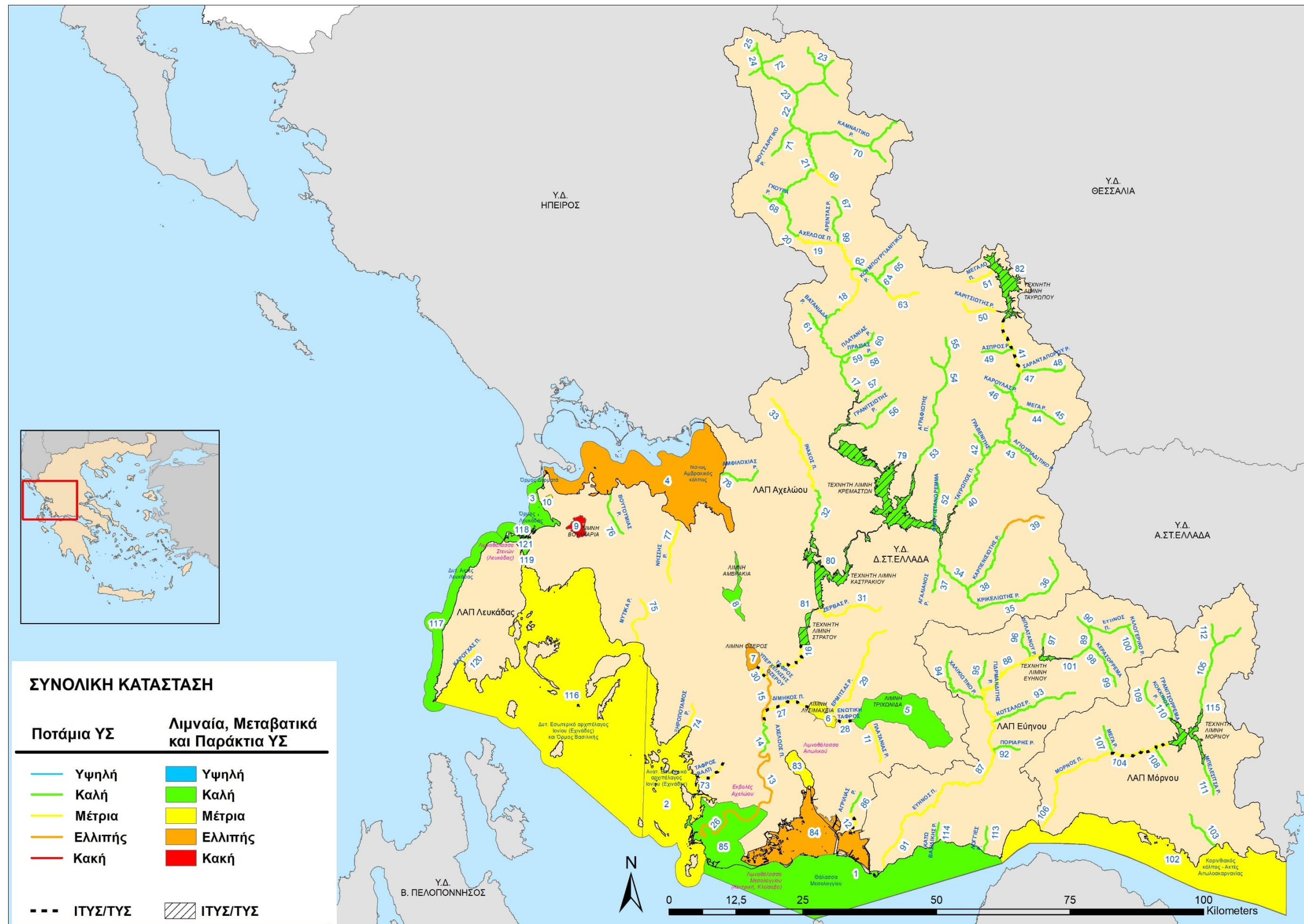
Χάρτης 8-3: Χάρτης ταξινόμησης της συνολικής κατάστασης των υδατικών συστημάτων του Υδατικού Διαμερίσματος Δυτικής Στερεάς Ελλάδας (EL04)
