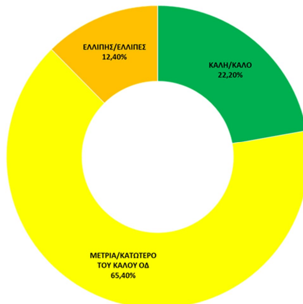
Σχήμα 8.5.1-2: Συνολική επιφάνεια (%) παράκτιων ΥΣ ανά κατηγορία οικολογικής κατάστασης – δυναμικού στο ΥΔ Δυτικής Στερεάς Ελλάδας (EL04)
