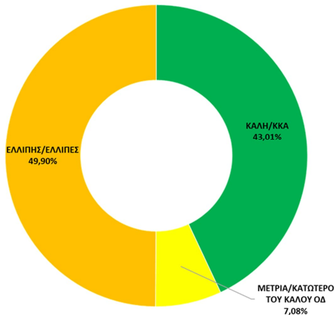
Σχήμα 8.4.1-2: Συνολική επιφάνεια (%) μεταβατικών ΥΣ ανά κατηγορία οικολογικής κατάστασης – δυναμικού στο ΥΔ Δυτικής Στερεάς Ελλάδας (EL04)
