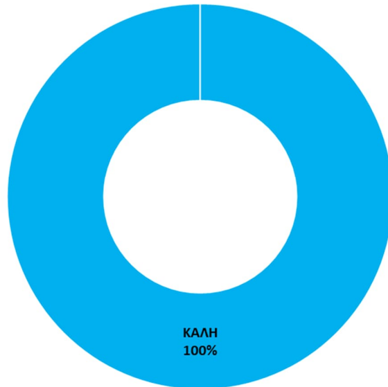
Σχήμα 8.3.1-3: Συνολικός αριθμός (%) λιμναίων ΥΣ ανά κατηγορία χημικής κατάστασης στο ΥΔ Δυτικής Στερεάς Ελλάδας (EL04)
