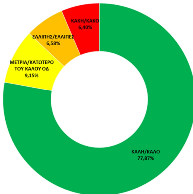
Σχήμα 8.3.1-2: Συνολική επιφάνεια (%) λιμναίων ΥΣ ανά κατηγορία οικολογικής κατάστασης – δυναμικού στο ΥΔ Δυτικής Στερεάς Ελλάδας (EL04)
