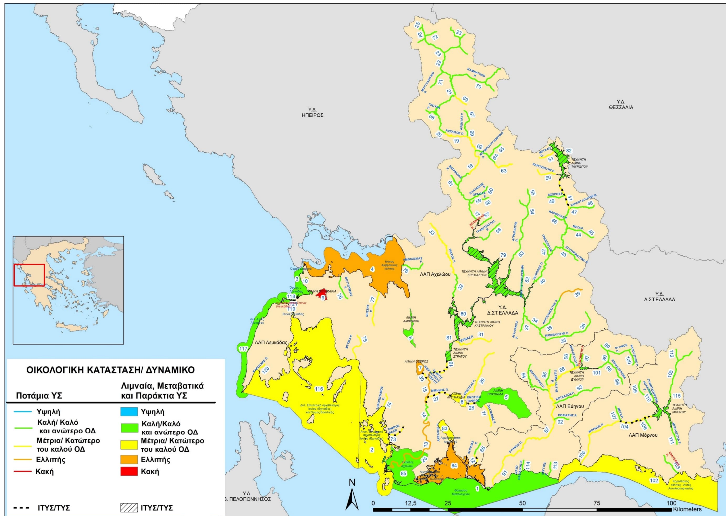
Χάρτης 8-1: Χάρτης ταξινόμησης της οικολογικής κατάστασης των υδατικών συστημάτων του Υδατικού Διαμερίσματος Δυτικής Στερεάς Ελλάδας (EL04)
