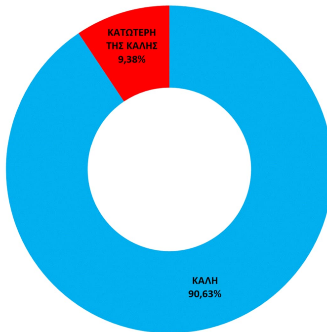
Σχήμα 8.2.2-1: Συνολικός αριθμός (%) ποτάμιων υδατικών συστημάτων ανά κατηγορία χημικής κατάστασης στο ΥΔ Δυτ. Στερεάς Ελλάδας (EL04)
