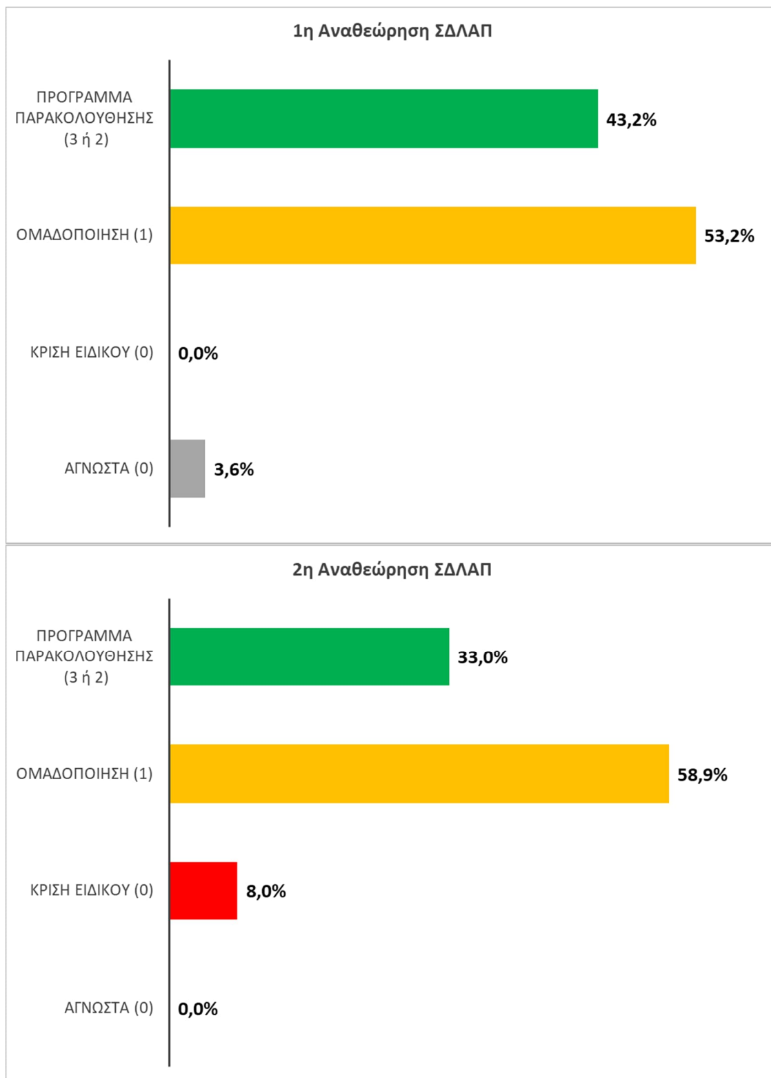
Σχήμα 8.6-2: Μέθοδος και επίπεδο εμπιστοσύνης ταξινόμησης της οικολογικής κατάστασης των επιφανειακών υδατικών συστημάτων στο ΥΔ Δυτικής Στερεάς Ελλάδας (EL04) σε σύγκριση με την εγκεκριμένη 1 η Αναθεώρηση των ΣΔΛΑΠ (δεν συμπεριλαμβάνονται τα ΙΤΥΣ, εκτός των ταμιευτήρων)
