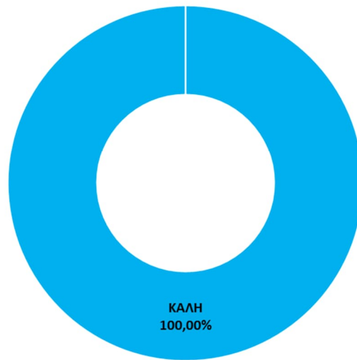
Σχήμα 8.3.2-3: Συνολικός αριθμός (%) ποτάμιων ΙΤΥΣ λιμναίου χαρακτήρα (ταμιευτήρων) ανά κατηγορία χημικής κατάστασης στο ΥΔ Δυτικής Στερεάς Ελλάδας (EL04)
