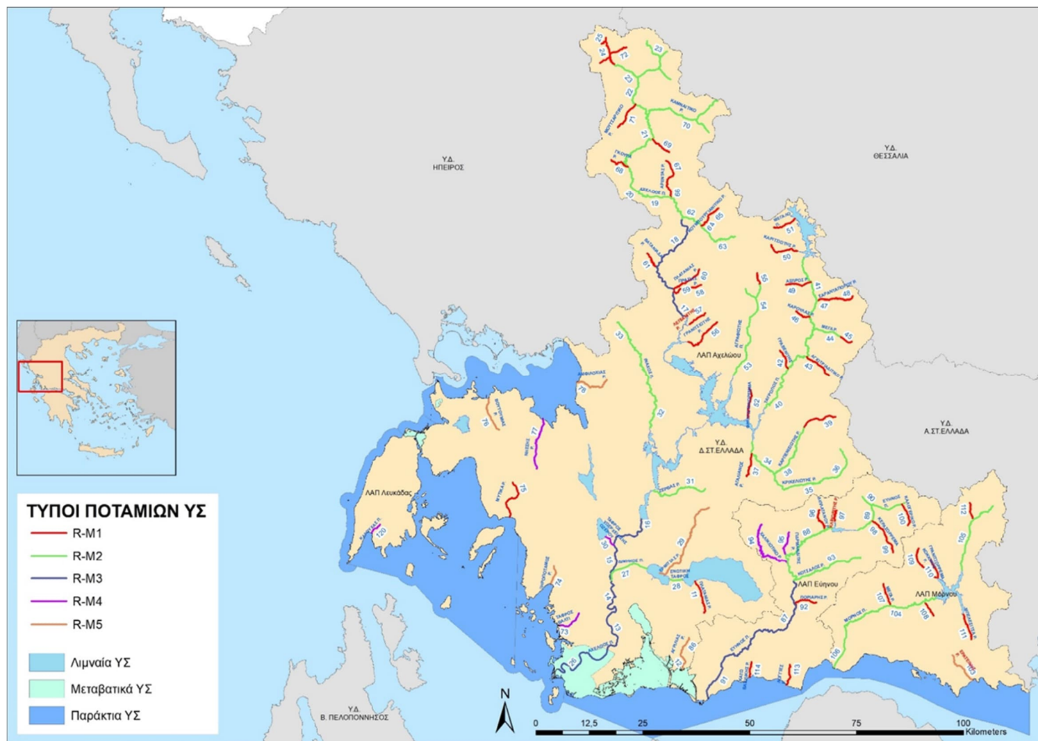
Χάρτης 4-2: Χάρτης τυπολογίας ποτάμιων ΥΣ ΥΔ Δυτικής Στερεάς Ελλάδας (EL04)
