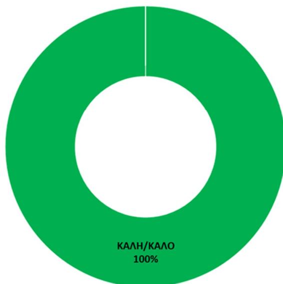
Σχήμα 8.3.2-1: Συνολικός αριθμός (%) ποτάμιων ΙΤΥΣ λιμναίου χαρακτήρα (ταμιευτήρων) ανά κατηγορία οικολογικής κατάστασης – δυναμικού στο ΥΔ Δυτικής Στερεάς Ελλάδας (EL04).
