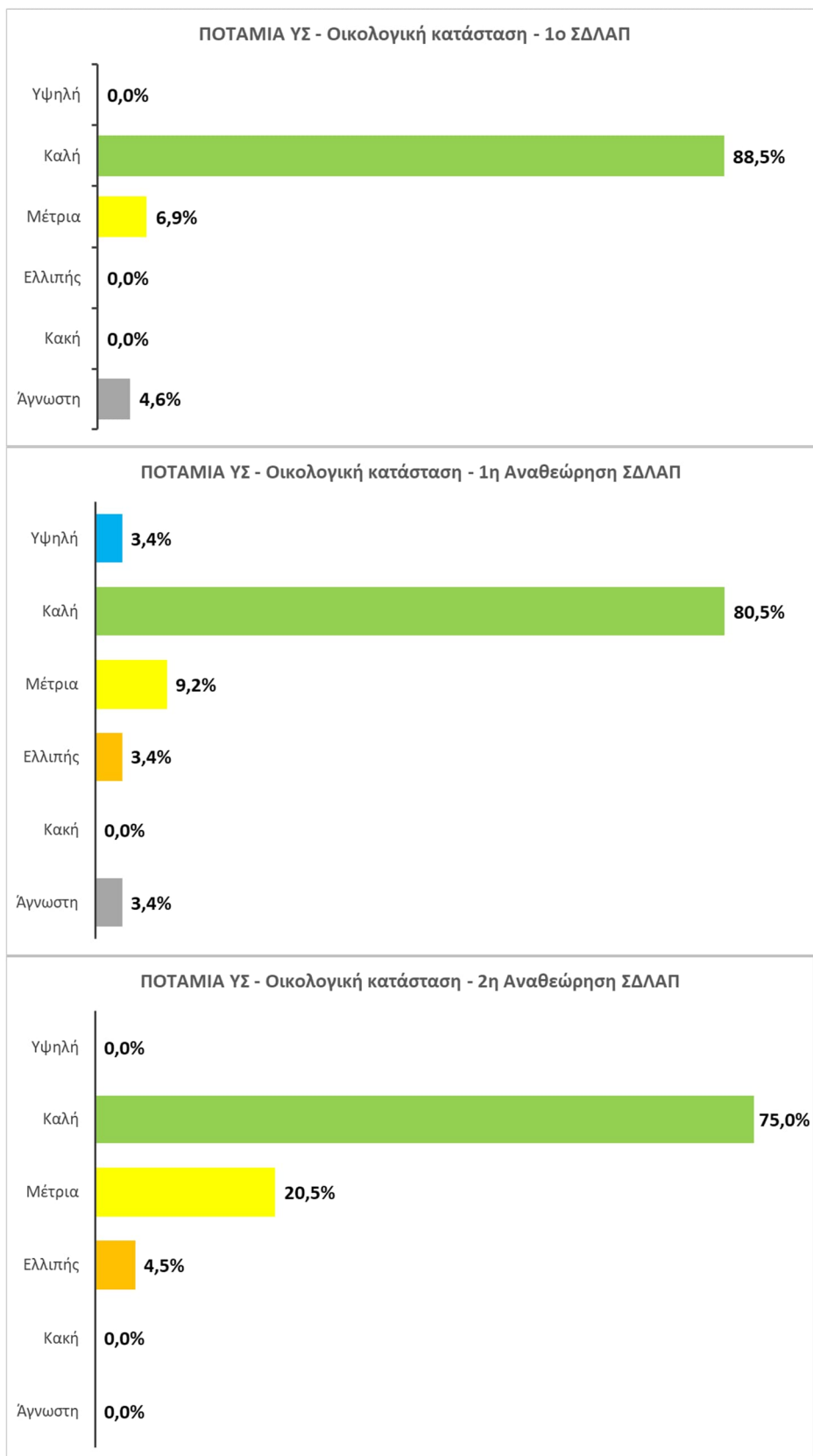
Σχήμα 8.2.1-3: Ταξινόμηση οικολογικής κατάστασης ποτάμιων υδατικών συστημάτων στο ΥΔ Δυτικής Στερεάς Ελλάδας (EL04) σε σύγκριση με τα προηγούμενα εγκεκριμένα ΣΔΛΑΠ (δεν συμπεριλαμβάνονται τα ΙΤΥΣ)
