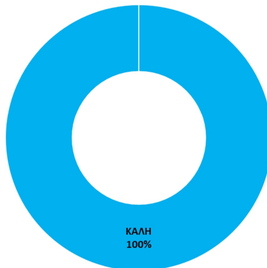
Σχήμα 8.3.2-4: Συνολική επιφάνεια (%) ποτάμιων ΙΤΥΣ λιμναίου χαρακτήρα (ταμιευτήρων) ανά κατηγορία χημικής κατάστασης στο ΥΔ Δυτικής Στερεάς Ελλάδας (EL04)
