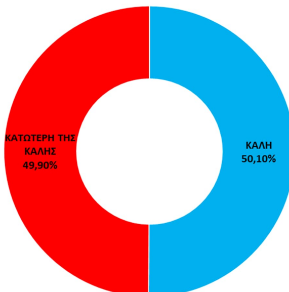
Σχήμα 8.4.2-2: Συνολική επιφάνεια (%) μεταβατικών ΥΣ ανά κατηγορία χημικής κατάστασης στο ΥΔ Δυτικής Στερεάς Ελλάδας (EL04)
