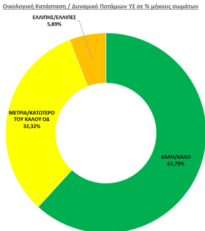
Σχήμα 8.2.1-2: Συνολικό μήκος (%) ποτάμιων υδατικών συστημάτων ανά κατηγορία οικολογικής κατάστασης – δυναμικού στο ΥΔ Δυτικής Στερεάς Ελλάδας (EL04)
