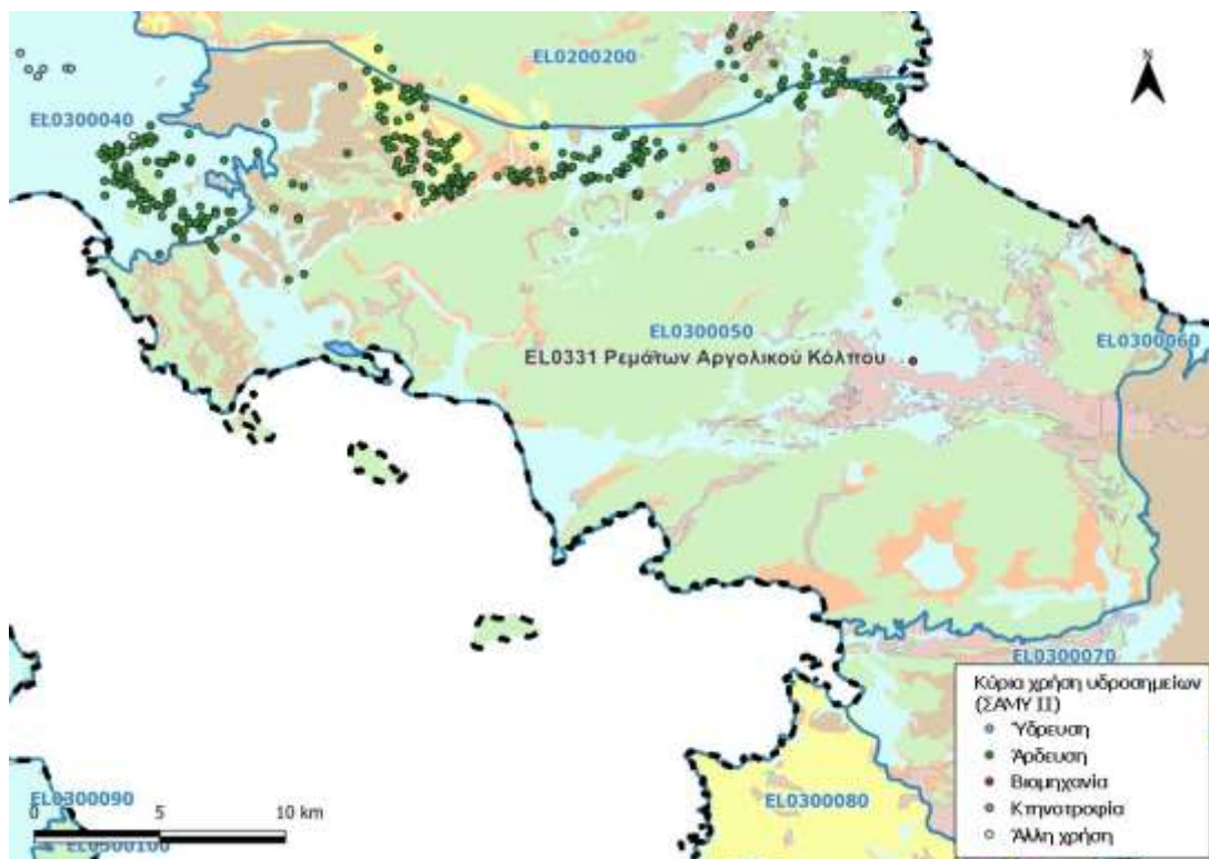
Εικόνα 7-23. Χάρτης χωρικής κατανομής υδροσημείων καταγραφής ΣΑΜΥ ΙΙ (ΕΑΓΜΕ)
