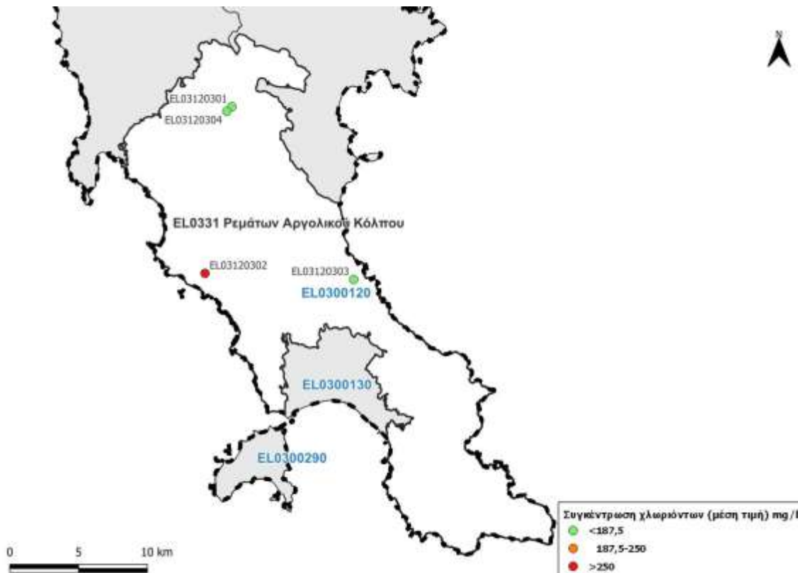
Εικόνα 7-72. Χάρτης συγκέντρωσης χλωριόντων του υπόγειου υδατικού συστήματος Νοτιοανατολικής Λακωνίας (ΕΛ0300120)
