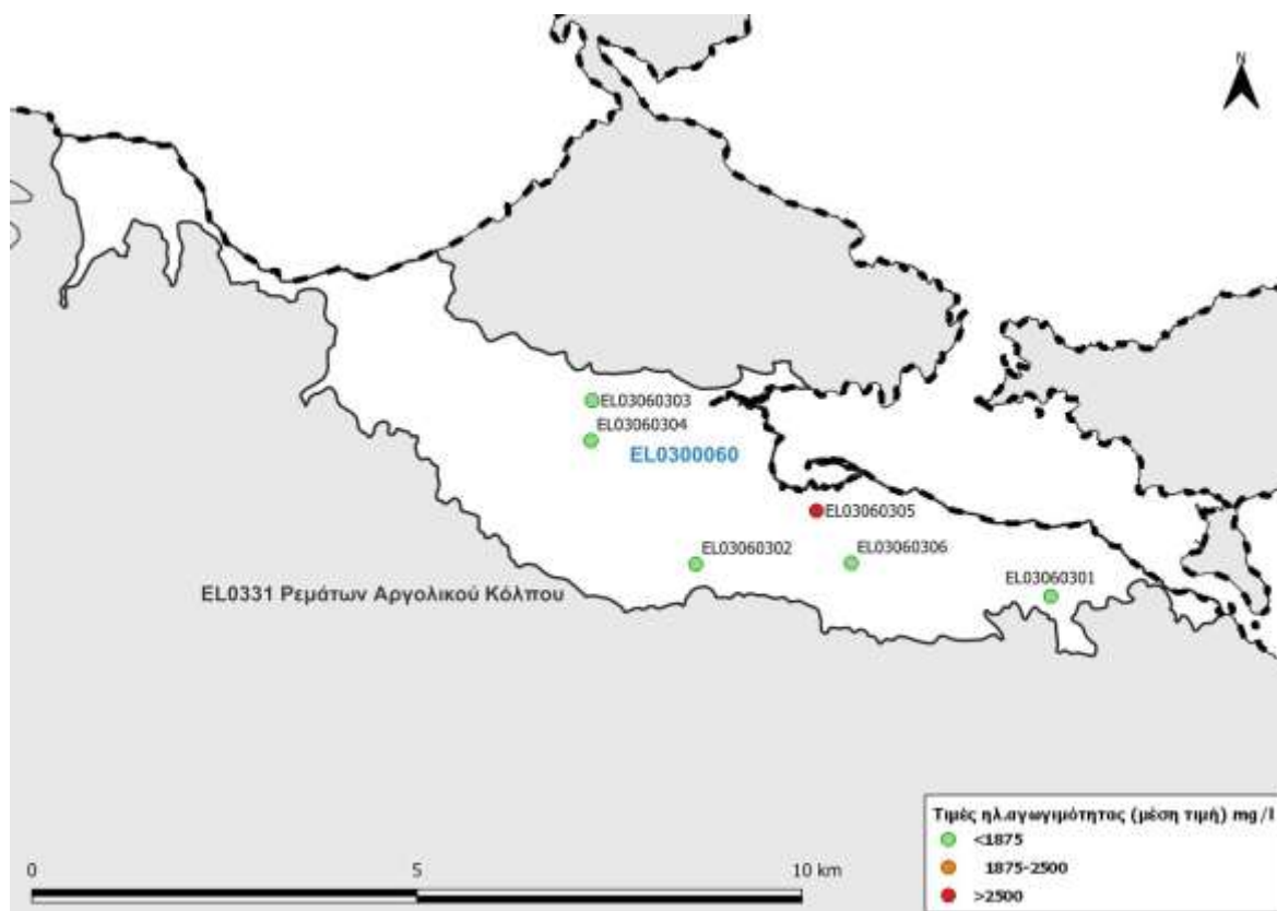
Εικόνα 7-27. Χάρτης τιμών ηλεκτρικής αγωγιμότητας του υπόγειου υδατικού συστήματος Τροιζηνίας (EL0300060)
