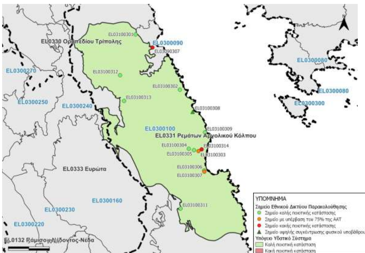
Εικόνα 7-60. Χάρτης χημικής κατάστασης υπόγειου υδατικού συστήματος Πάρνωνα (ΕΛ0300100)
