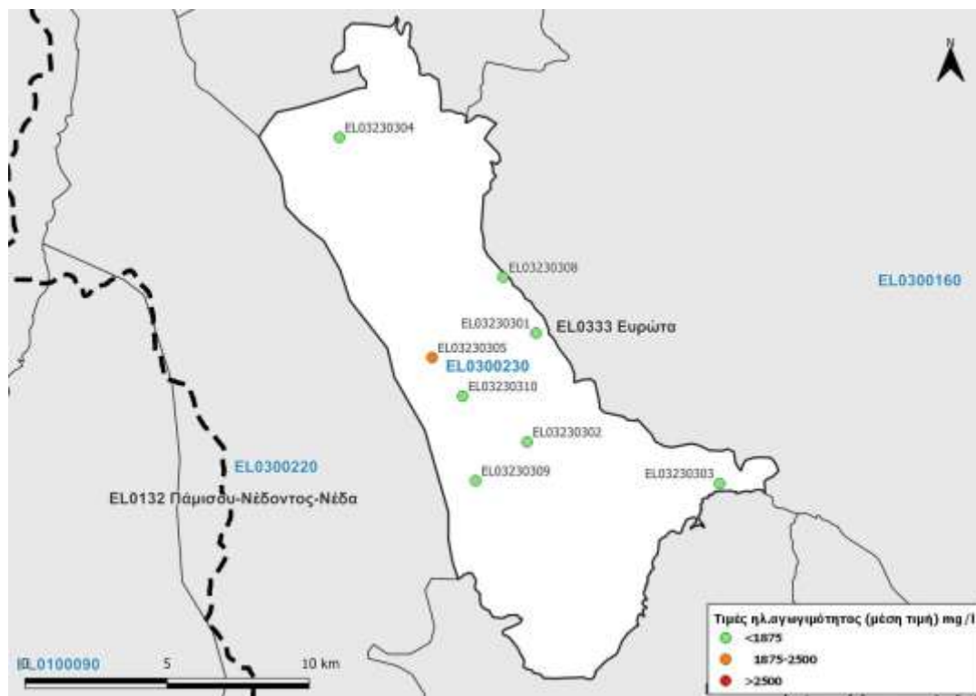
Εικόνα 8-37. Χάρτης τιμών ηλεκτρικής αγωγιμότητας του υπόγειου υδατικού συστήματος Ευρώτα (EL0300230)
