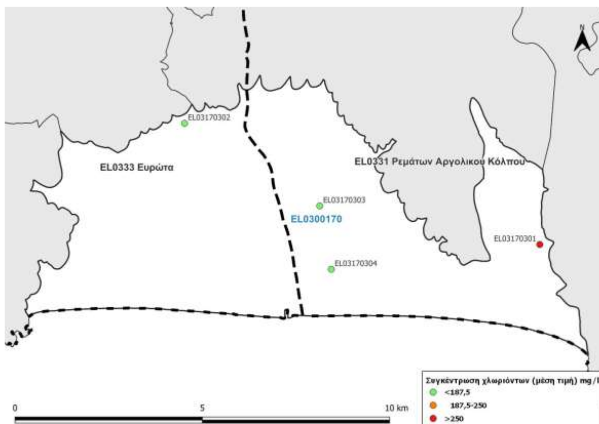
Εικόνα 8-8. Χάρτης συγκέντρωσης χλωριόντων του υπόγειου υδατικού συστήματος Έλους - Βασιλοποτάμου (ΕΛ0300170)
