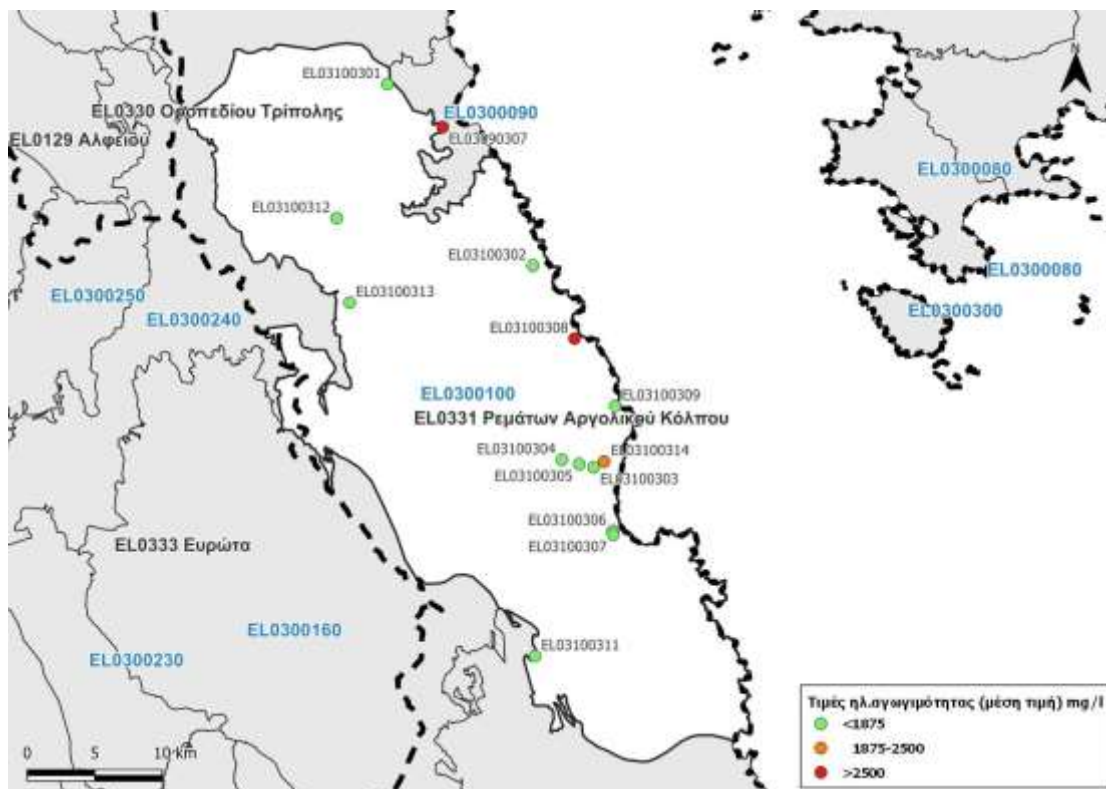
Εικόνα 7-56. Χάρτης τιμών ηλεκτρικής αγωγιμότητας του υπόγειου υδατικού συστήματος Πάρνωνα (EL0300100)
