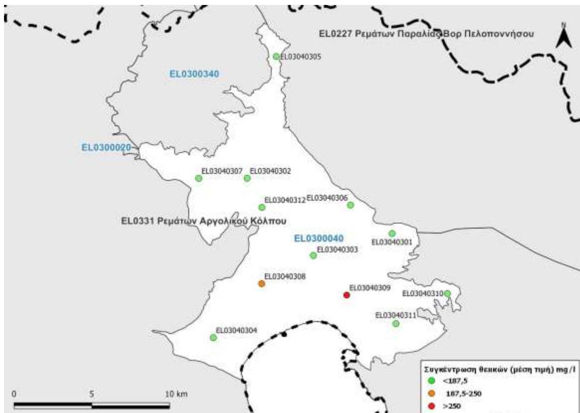
Εικόνα 7-12. Χάρτης συγκέντρωσης θεικών του υπόγειου υδατικού συστήματος Αργολικού Πεδίου (EL0300040)
