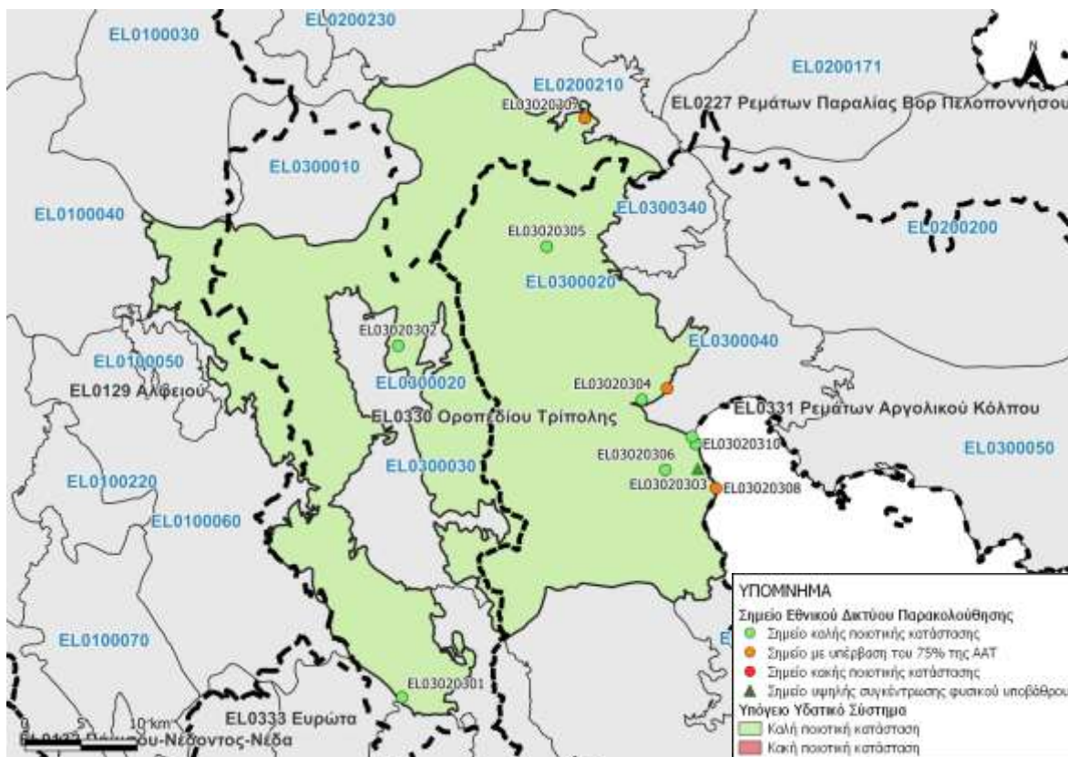
Εικόνα 7-4. Χάρτης χημικής κατάστασης υπόγειου υδατικού συστήματος Αν. Αρκαδίας-Δυτ. Αργολίδας (ΕΛ0300020)
