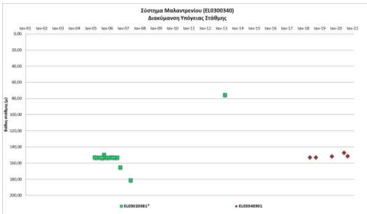
Σχήμα 7-22. Διάγραμμα διακύμανσης στάθμης γεωτρήσεων υπόγειου υδατικού συστήματος Νεογενών Μαλαντρενίου (EL0300340)
