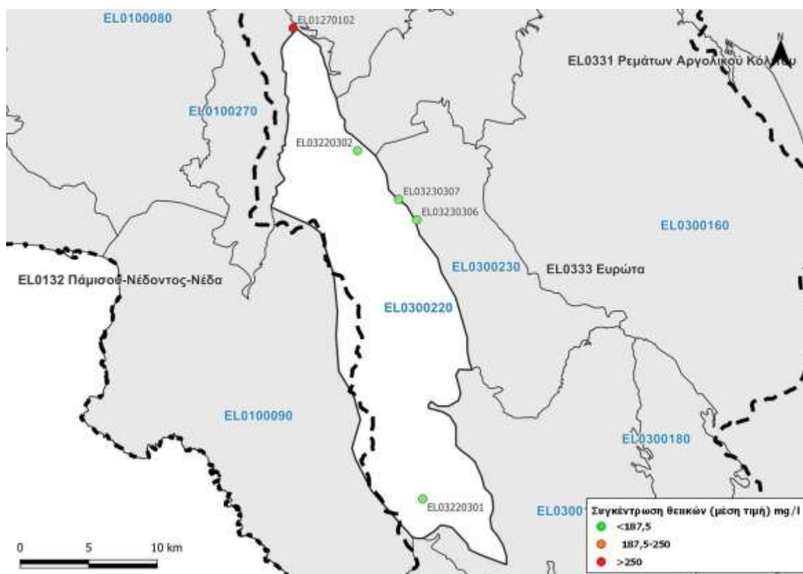
Εικόνα 8-32. Χάρτης συγκέντρωσης θεικών του υπόγειου υδατικού συστήματος Αν. Ταυγέτου – Αγ.Μαρίνας (ΕΛ0300220)
