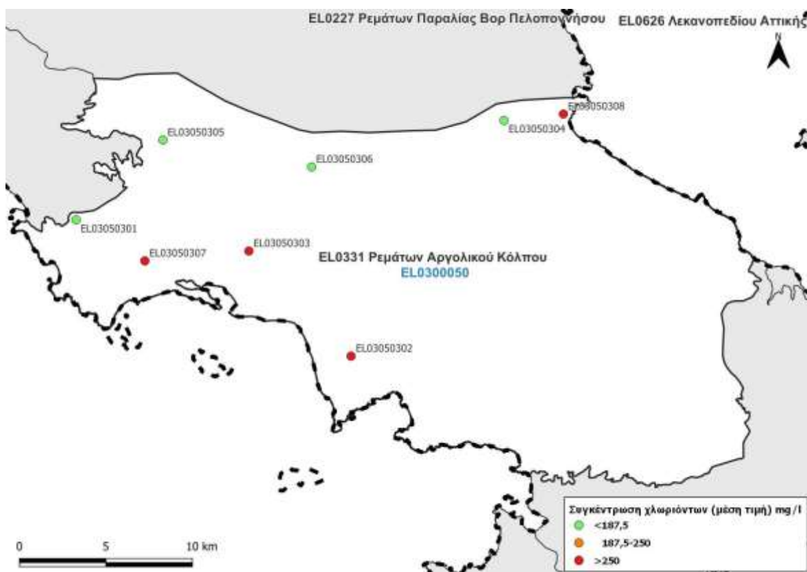
Εικόνα 7-20. Χάρτης συγκέντρωσης χλωριόντων του υπόγειου υδατικού συστήματος Μαυροβουνίου - Διδύμων (ΕΛ0300050)
