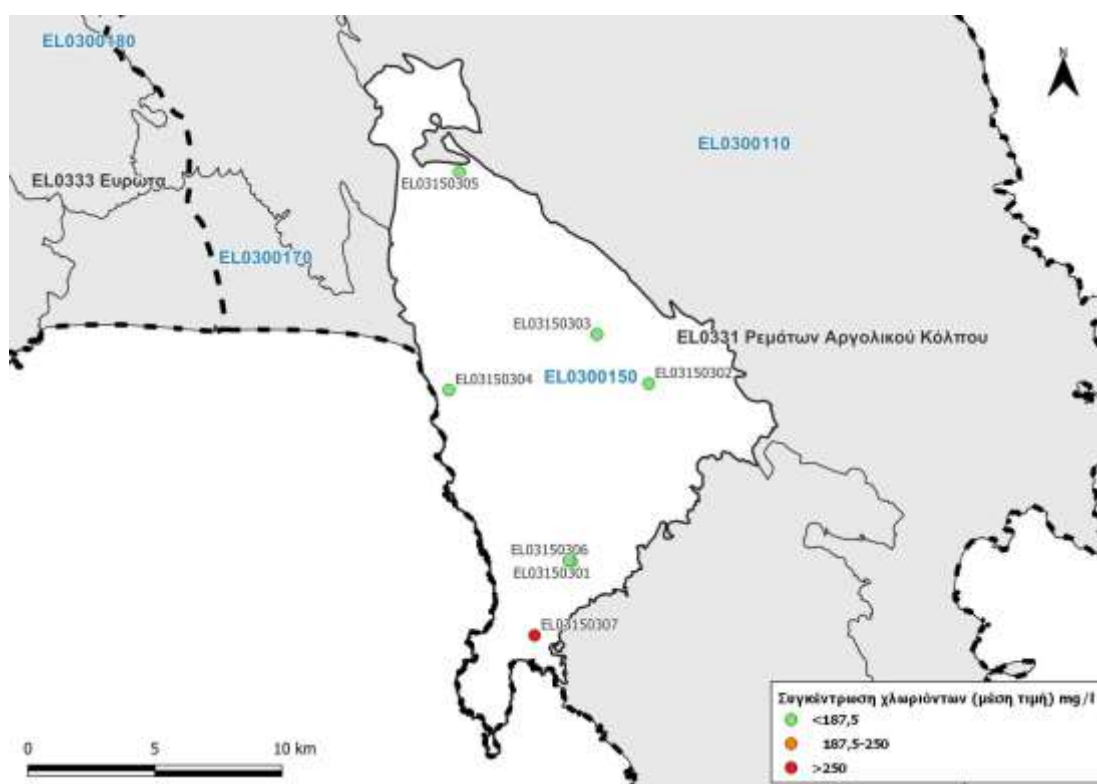
Εικόνα 7-89. Χάρτης συγκέντρωσης χλωριόντων του υπόγειου υδατικού συστήματος Ασωπού - Γλυκόβρυσης (EL0300150)
