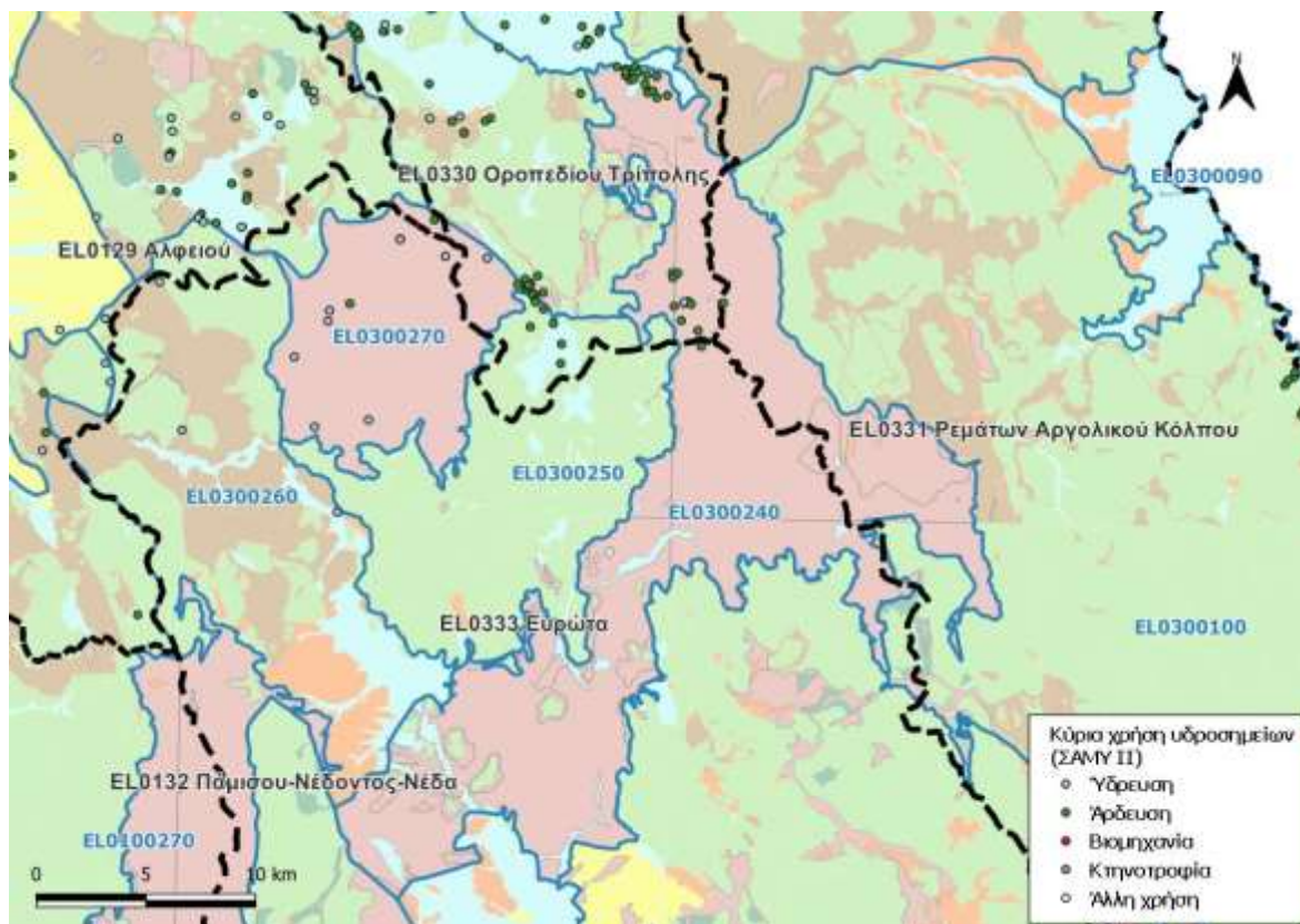
Εικόνα 8-44. Χάρτης χωρικής κατανομής υδροσημείων καταγραφής ΣΑΜΥ II (ΕΑΓΜΕ)
