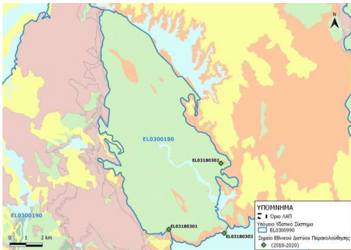
Εικόνα 8-12. Σημεία παρακολούθησης υπόγειου υδατικού συστήματος Σκάλας (EL0300180)
