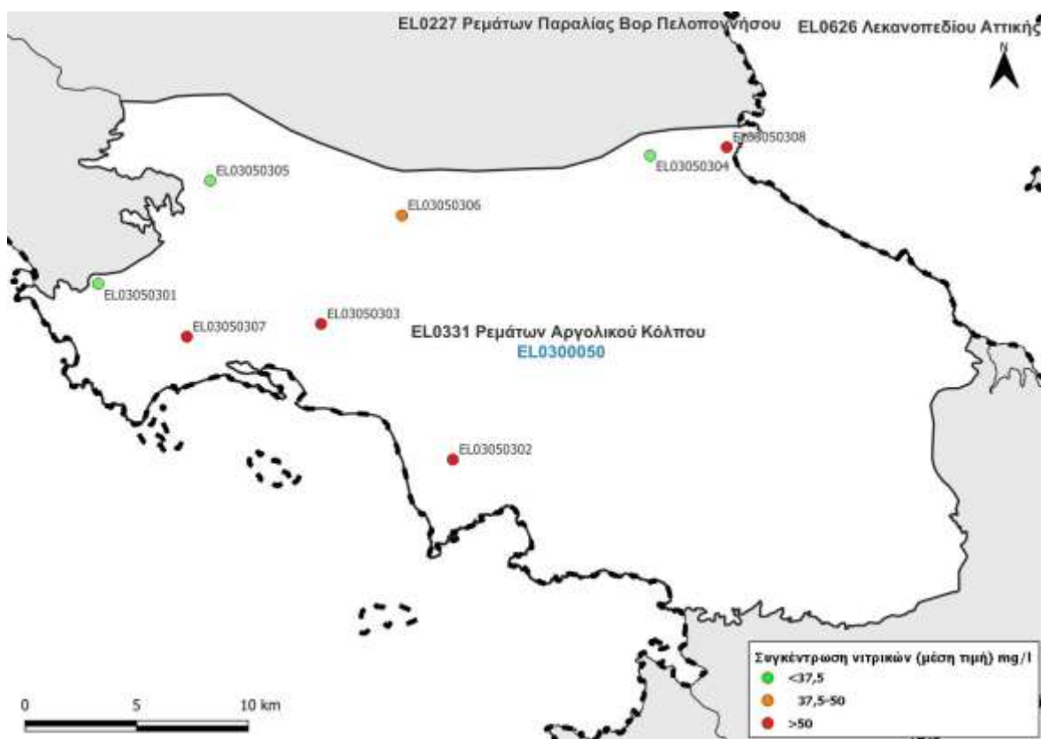
Εικόνα 7-19. Χάρτης συγκέντρωσης νιτρικών του υπόγειου υδατικού συστήματος Μαυροβουνίου - Διδύμων (ΕΛ0300050)
