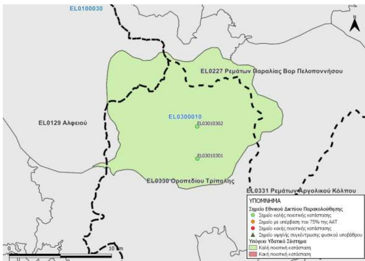
Εικόνα 6-2. Χάρτης χημικής κατάστασης υπόγειου υδατικού συστήματος Κανδήλας (EL0300010)
