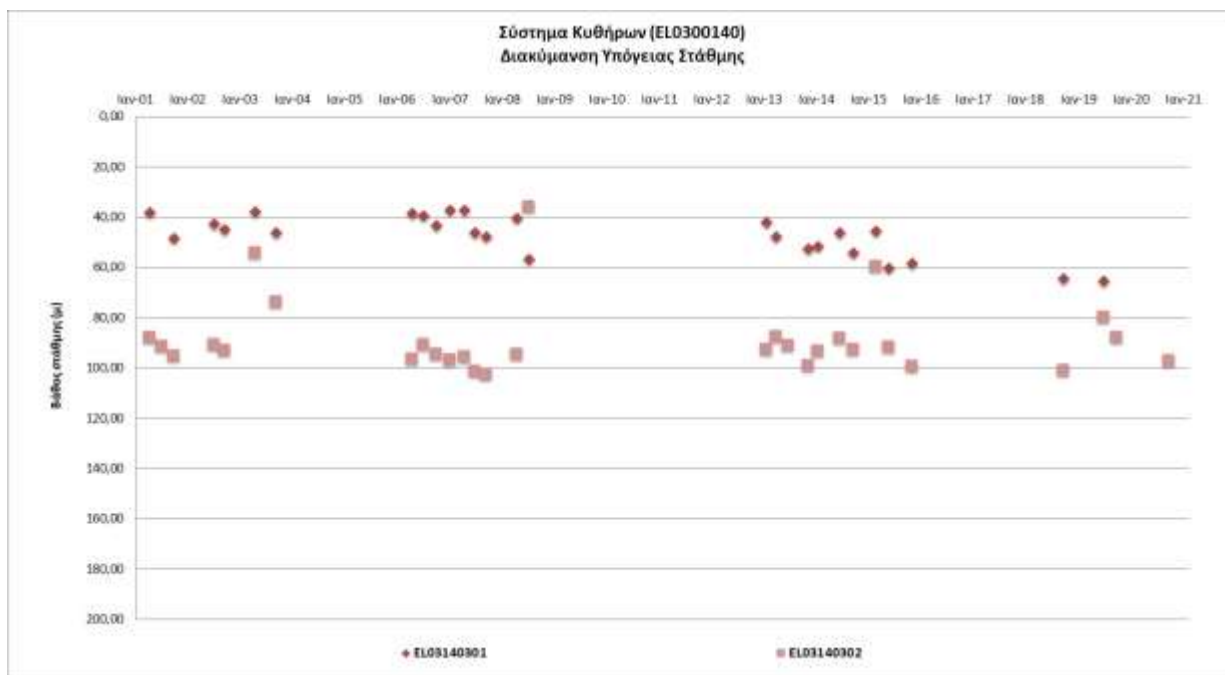
Σχήμα 7-20. Διάγραμμα διακύμανσης στάθμης γεωτρήσεων υπόγειου υδατικού συστήματος Κυθήρων (EL0300140)
