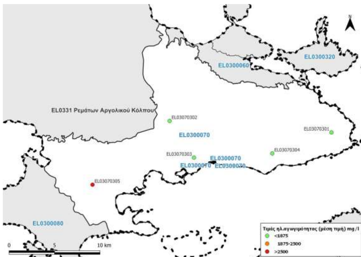
Εικόνα 7-34. Χάρτης τιμών ηλεκτρικής αγωγιμότητας του υπόγειου υδατικού συστήματος Ερμιόνης (ΕΛ0300070060)
