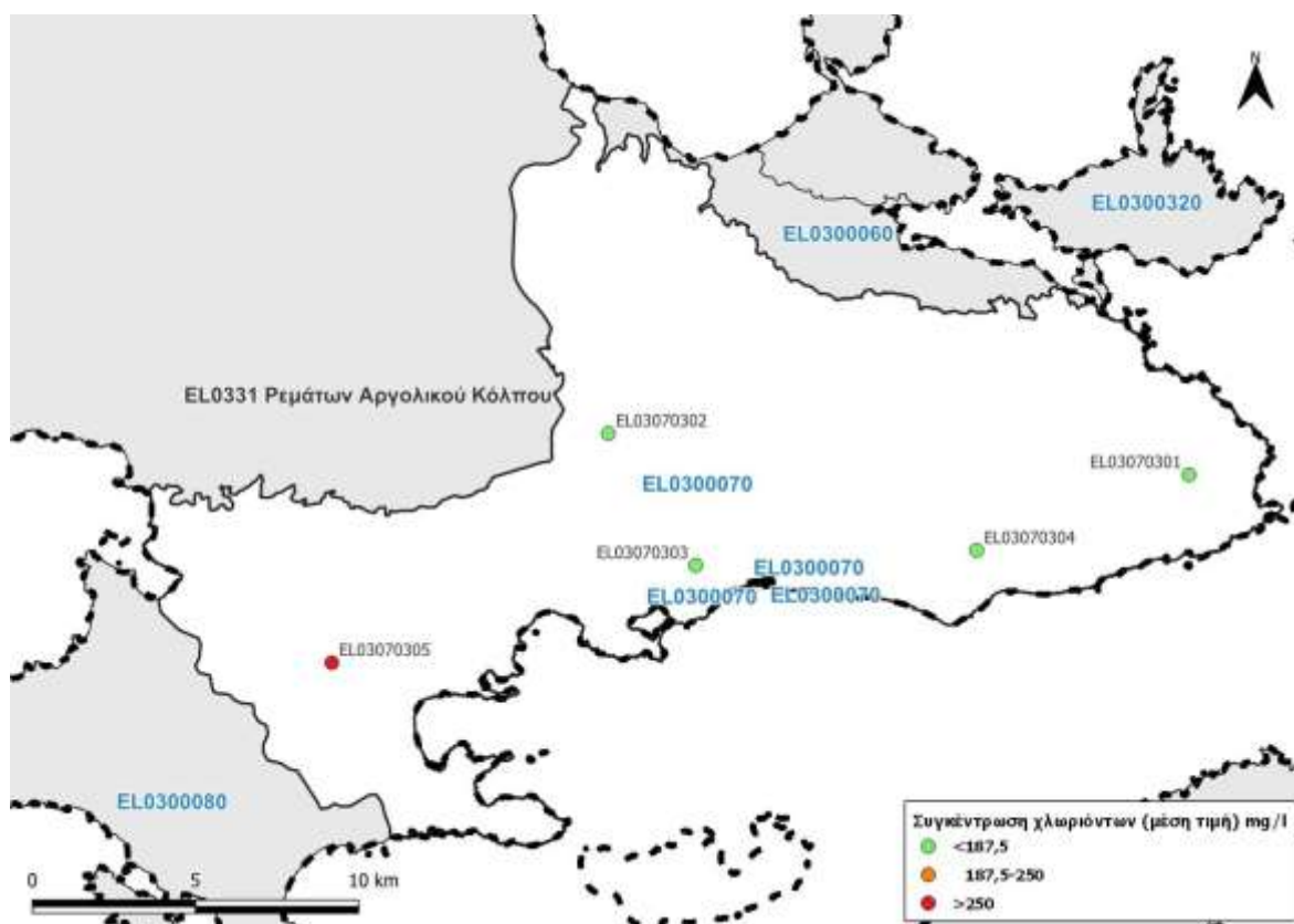
Εικόνα 7-36. Χάρτης συγκέντρωσης χλωριόντων του υπόγειου υδατικού συστήματος Ερμιόνης (EL0300070)
