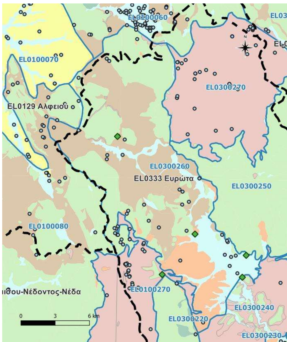
Εικόνα 8-55. Χάρτης Εθνικού Μητρώου Σημείων Υδροληψίας και σημείων εθνικού δικτύου παρακολούθησης
