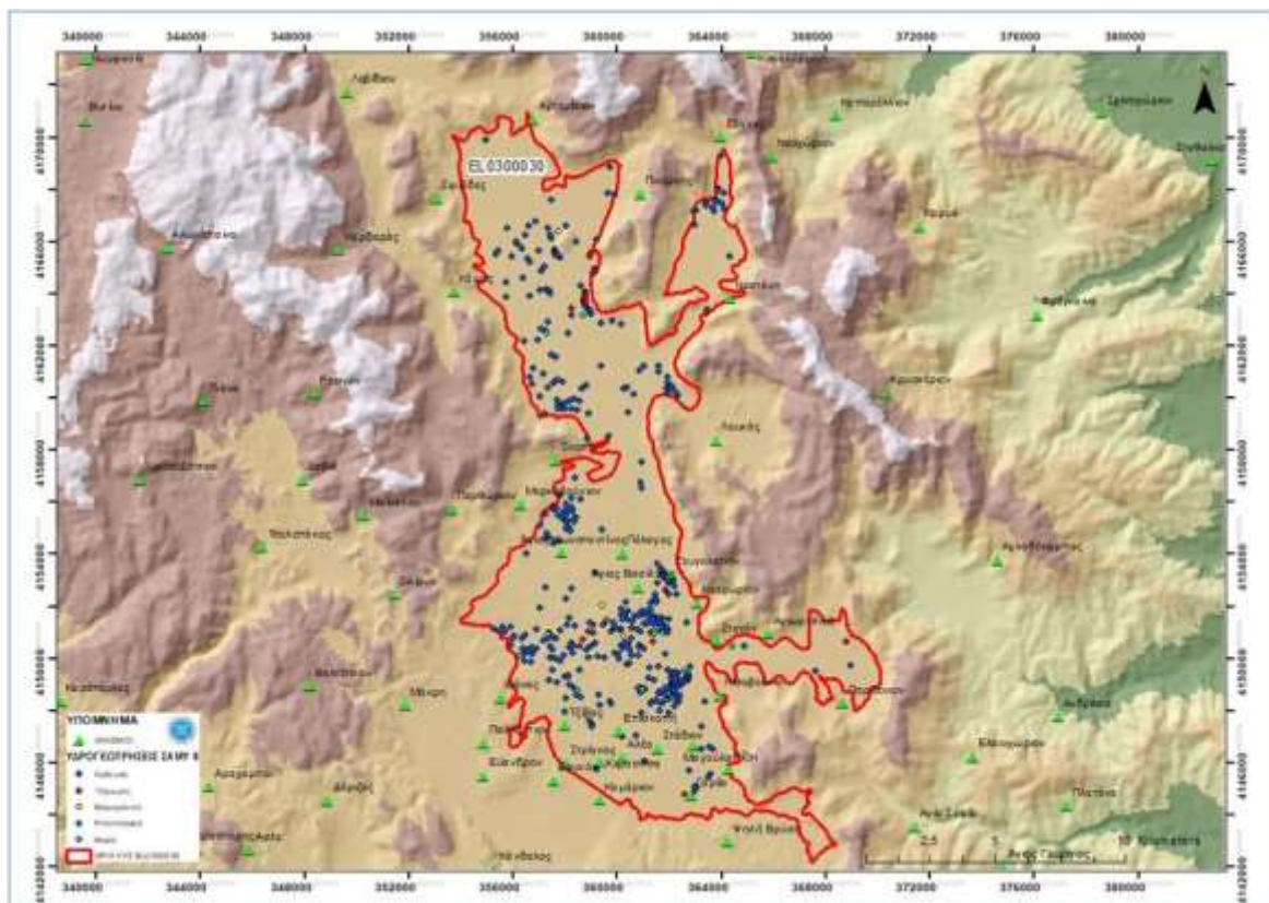
Εικόνα 6-10. Χάρτης χωρικής κατανομής των απογεγραμμένων υδρογεωτρήσεων του ΥΥΣ ΕΛ0300030 κλίμακας 1:50.000 σε προσαρμογή. Στο υπόμνημα διακρίνονται οι γεωτρήσεις άρδευσης, ύδρευσης, βιομηχανικής χρήσης, κτηνοτροφικής, καμία και άλλη χρήση (ΣΑΜΥ II – ΕΑΓΜΕ 2021)
