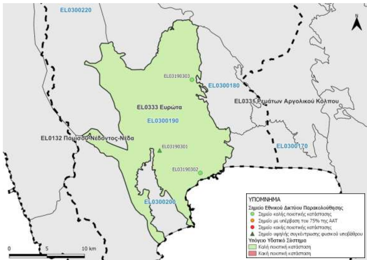
Εικόνα 8-19. Χάρτης χημικής κατάστασης υπόγειου υδατικού συστήματος Κροκεών – Γυθείου (ΕΛ0300190)
