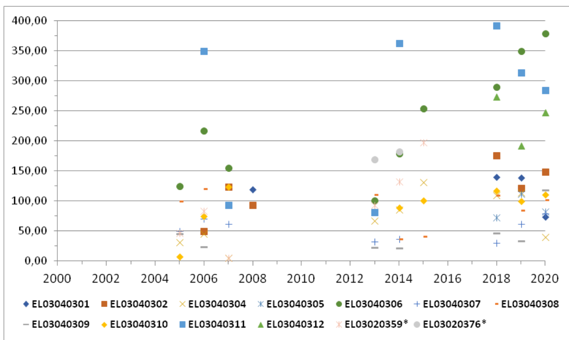
Σχήμα 7-4. Διάγραμμα διαμέσων τιμών συγκέντρωσης νιτρικών ( \text{NO}_3 ) των σημείων παρατήρησης του υπόγειου υδατικού συστήματος Αργολικού Πεδίου (EL0300040) με υπερβάσεις των τιμών ΑΑΤ ή/και του 75% αυτών ανά έτος παρατήρησης
