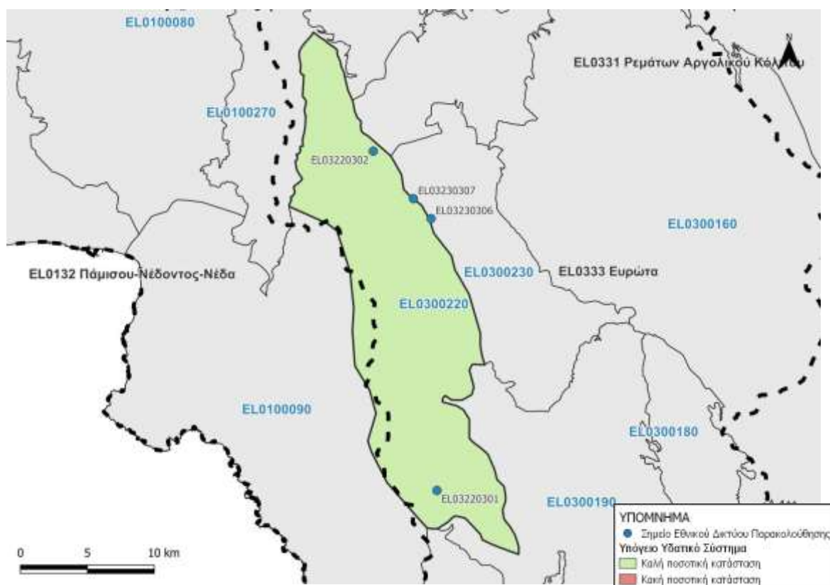
Εικόνα 8-35. Χάρτης ποσοτικής κατάστασης υπόγειου υδατικού συστήματος Αν. Ταυγέτου – Αγ.Μαρίνας (EL0300220)
