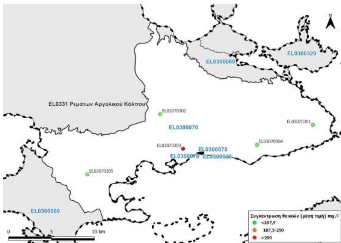
Εικόνα 7-35. Χάρτης συγκέντρωσης θεικών του υπόγειου υδατικού συστήματος Ερμιόνης (ΕΛ0300070)
