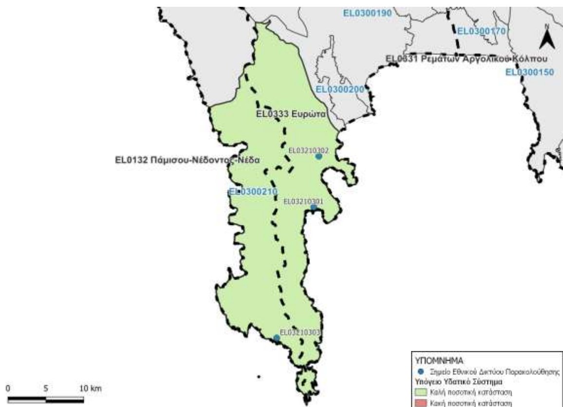
Εικόνα 8-30. Χάρτης ποσοτικής κατάστασης υπόγειου υδατικού συστήματος Σκουταρίου (EL0300210)
