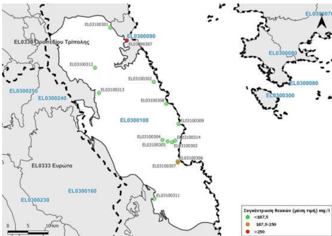
Εικόνα 7-59. Χάρτης συγκέντρωσης θεικών του υπόγειου υδατικού συστήματος Πάρωνα (ΕΛ0300100)
