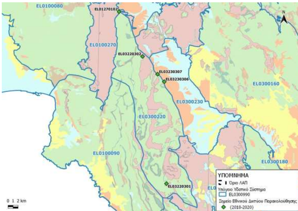
Εικόνα 8-31. Σημεία παρακολούθησης υπόγειου υδατικού συστήματος Αν. Ταυγέτου – Αγ.Μαρίνας (EL0300220)
