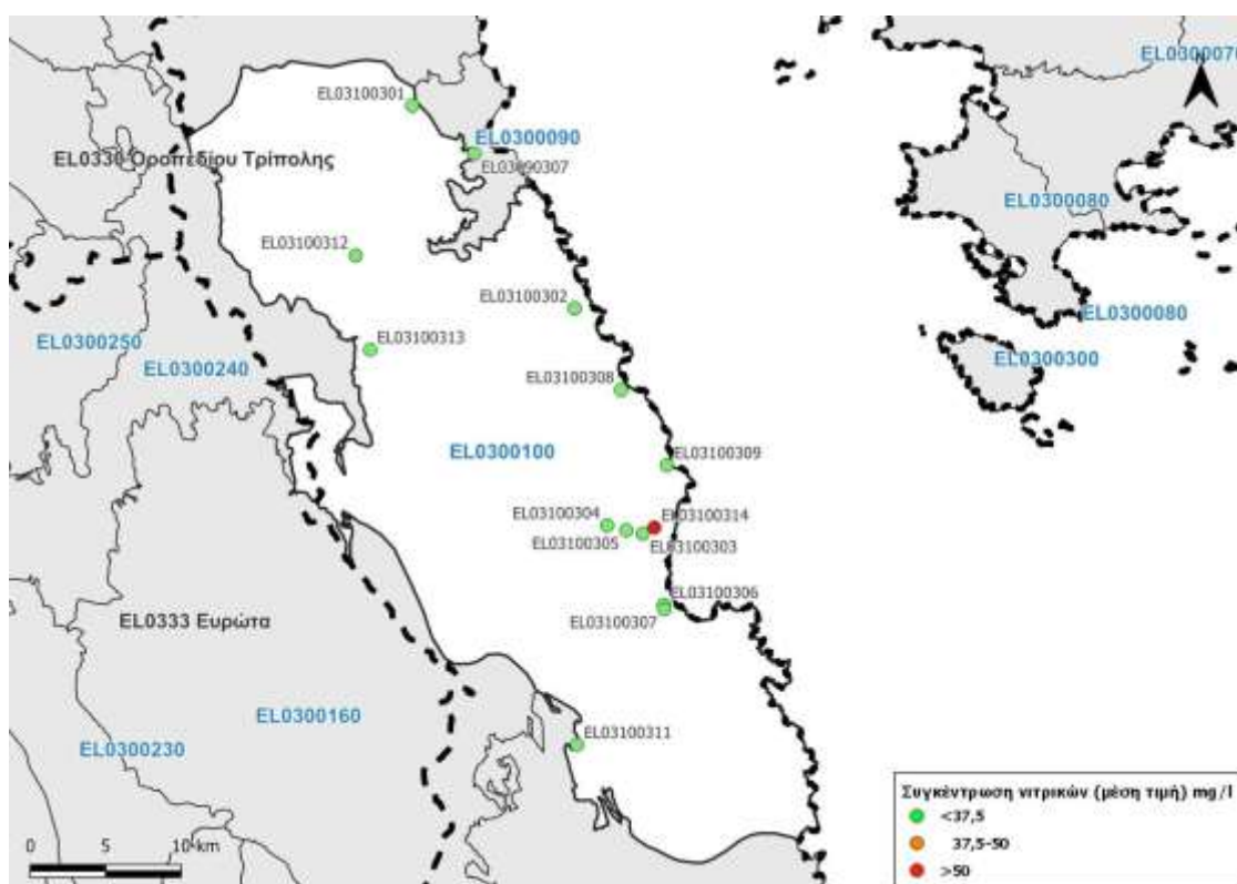
Εικόνα 7-57. Χάρτης συγκέντρωσης νιτρικών του υπόγειου υδατικού συστήματος Πάρνωνα (EL0300100)
