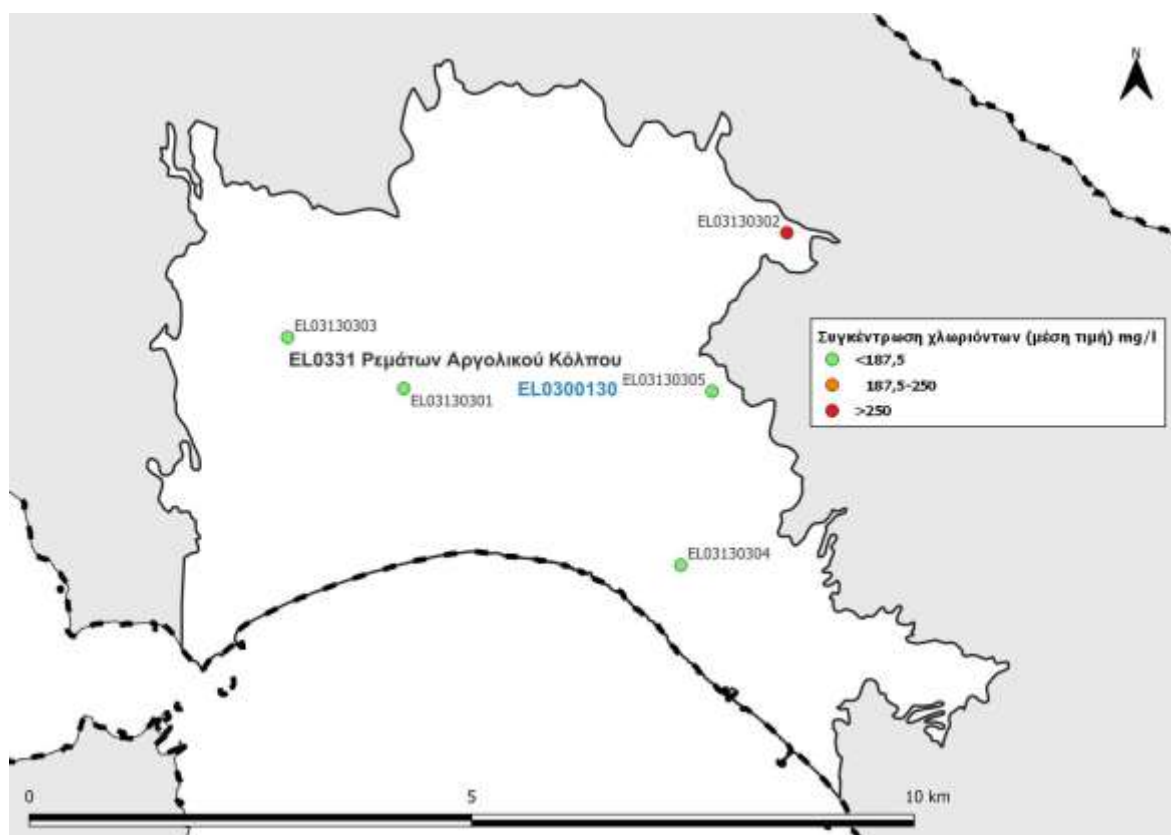
Εικόνα 7-78. Χάρτης συγκέντρωσης χλωριόντων του υπόγειου υδατικού συστήματος Νεάπολης (EL0300130)
