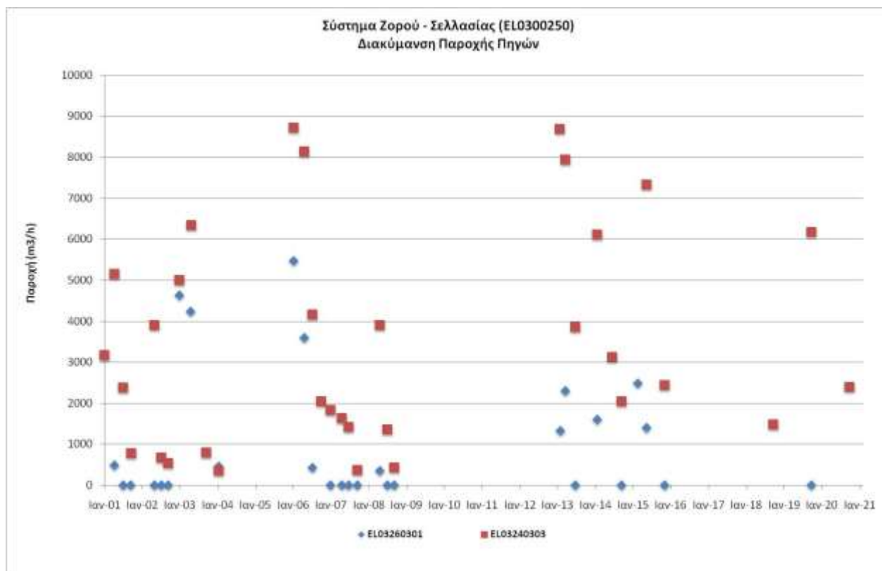
Σχήμα 8-11. Διάγραμμα διακύμανσης παροχής πηγών υπόγειου υδατικού συστήματος Ζορού - Σελλασίας (ΕΛ0300250)
