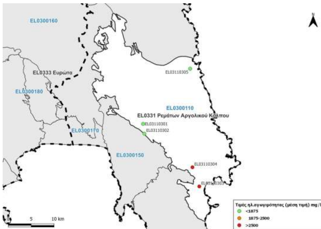
Εικόνα 7-65. Χάρτης τιμών ηλεκτρικής αγωγιμότητας του υπόγειου υδατικού συστήματος Ζάρακα – Μονεμβασιάς (EL0300110)
