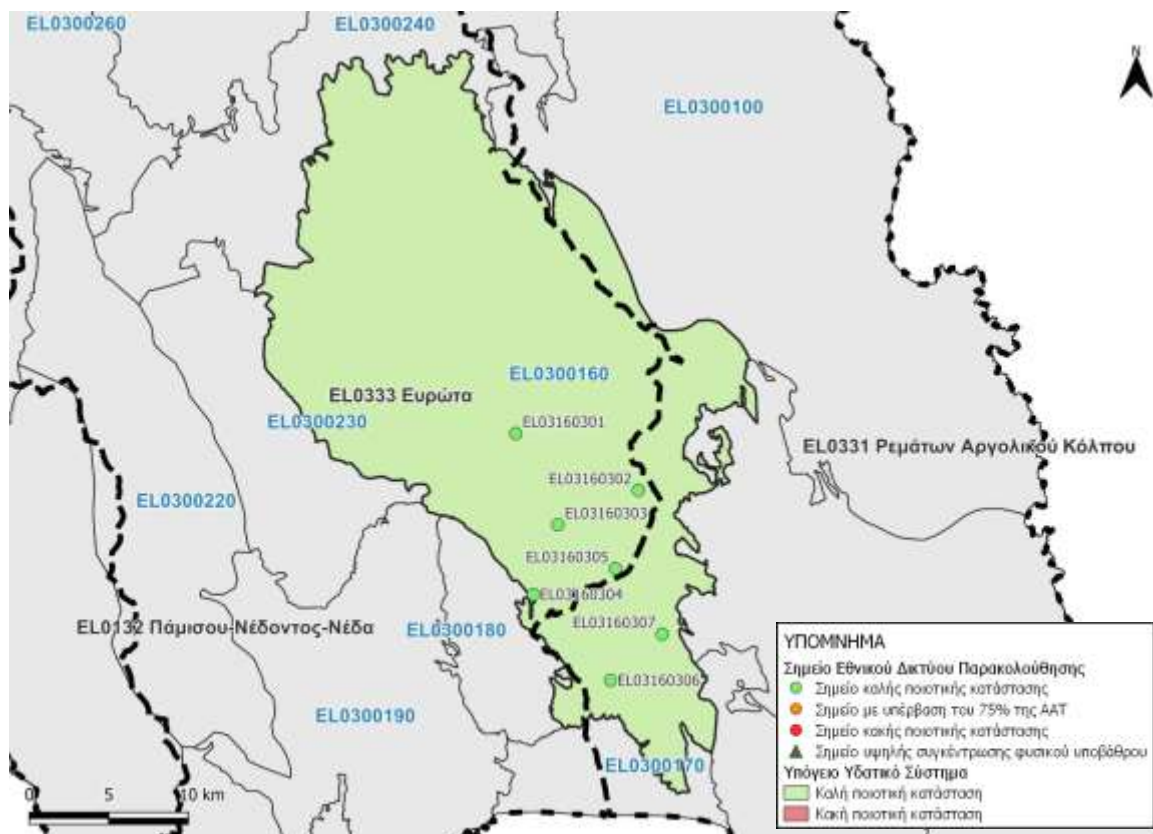
Εικόνα 8-2. Χάρτης χημικής κατάστασης υπόγειου υδατικού συστήματος Γερακίου - Γκοριτσάς (EL0300160)
