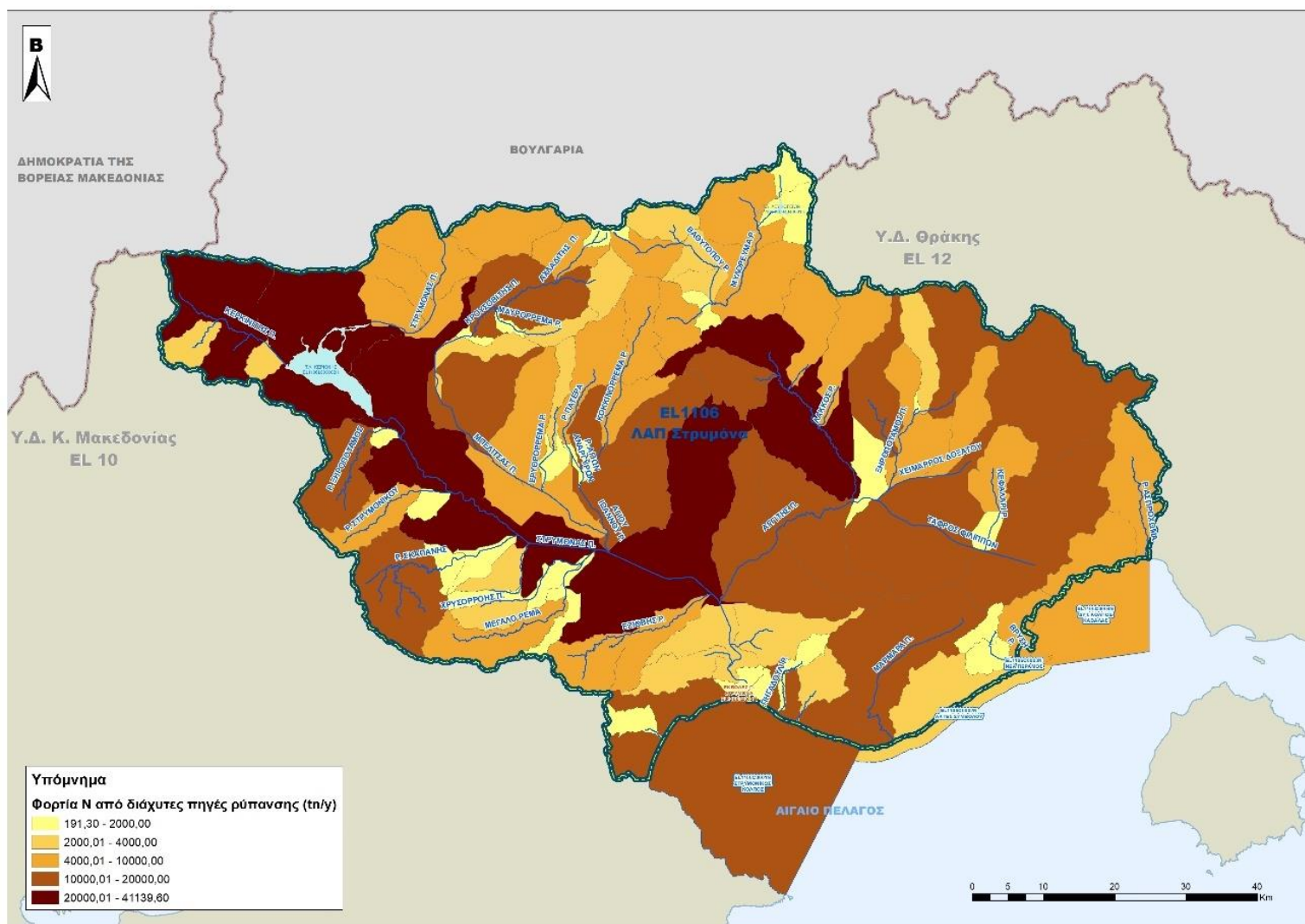
Χάρτης 5-6: Ετήσια φορτία N (tn/year) που απορρέουν στο ΥΔ Ανατολικής Μακεδονίας (EL11) από διάχυτες πηγές ρύπανσης
