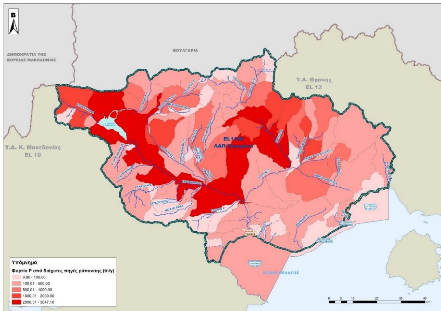
Χάρτης 5-7: Ετήσια φορτία P (tn/year) που απορρέουν στο ΥΔ Ανατολικής Μακεδονίας (EL11) από διάχυτες πηγές ρύπανσης
