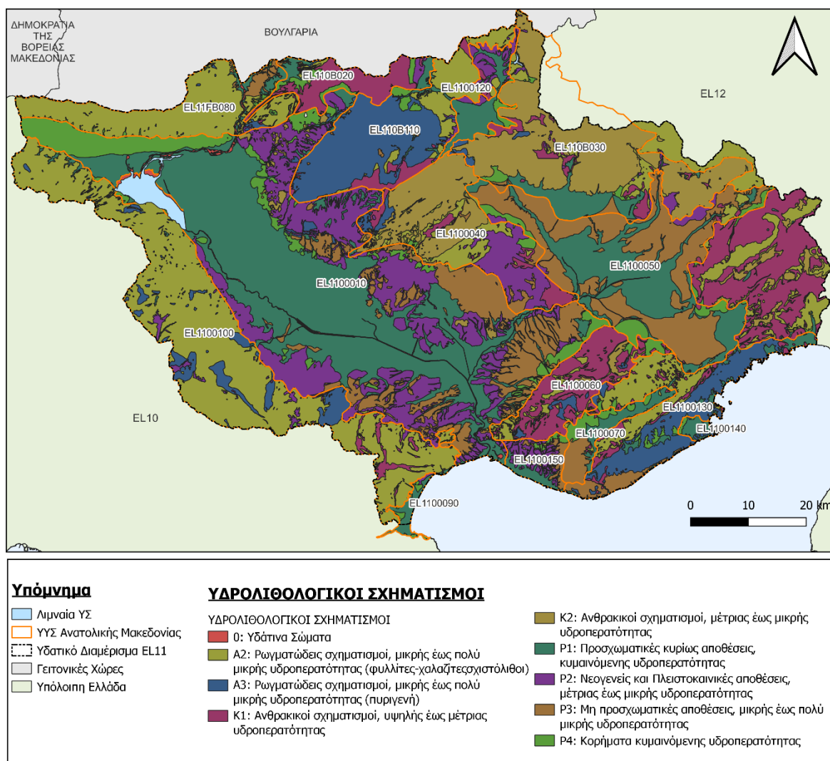
Χάρτης 3-3: Υδρολιθολογικός Χάρτης Υδατικού Διαμερίσματος Ανατολικής Μακεδονίας
