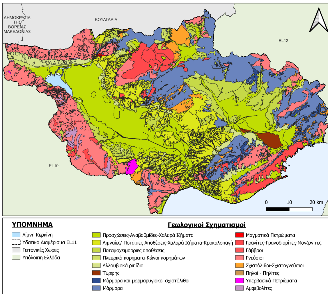
Χάρτης 3-2: Γεωλογικός Χάρτης Υδατικού Διαμερίσματος Ανατολικής Μακεδονίας (EL11) [ΓΓΜΕ, Κλίμακα 1:500.000]
