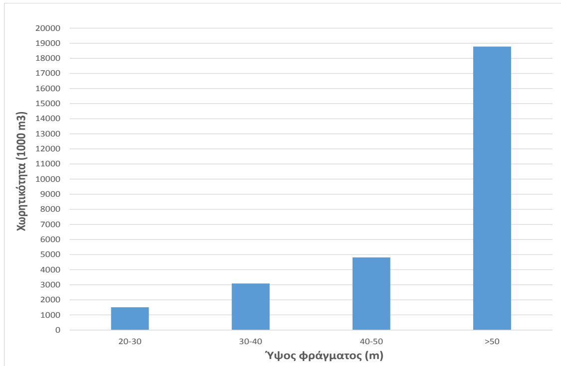
Διάγραμμα 3.2. Σχέση ύψους φράγματος και μέσης χωρητικότητας ταμιευτήρα για 47 μελετηθέντα και κατασκευασθέντα έργα εσωποτάμιας ταμίευσης κυρίως σε νησιωτικές περιοχές (ΥΠΑΑΤ, 2006)
