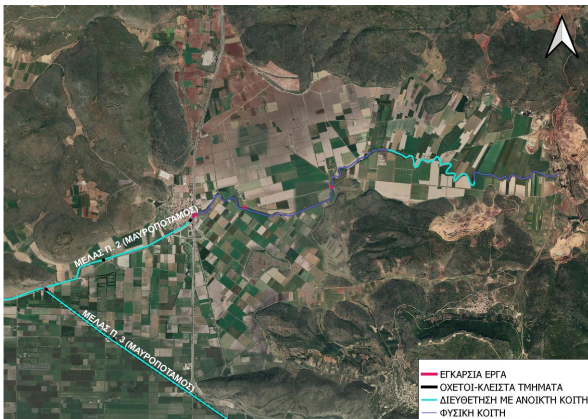
Εικόνα 3-8: Απεικόνιση Κριτηρίων Αξιολόγησης Υδρομορφολογικών Αλλοιώσεων στον Μέλα Π. 2
