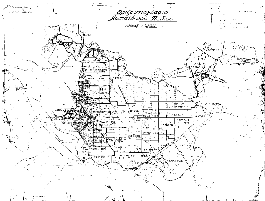
Εικόνα 3-6: Έργα Αποστράγγισης / Άρδευσης Κωπαϊδας
