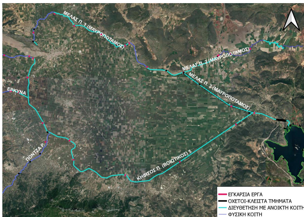
Εικόνα 3-7: Απεικόνιση Κριτηρίων Αξιολόγησης Υδρομορφολογικών Αλλοιώσεων στον Κηφισό Π. (Βοιωτικός) 5
