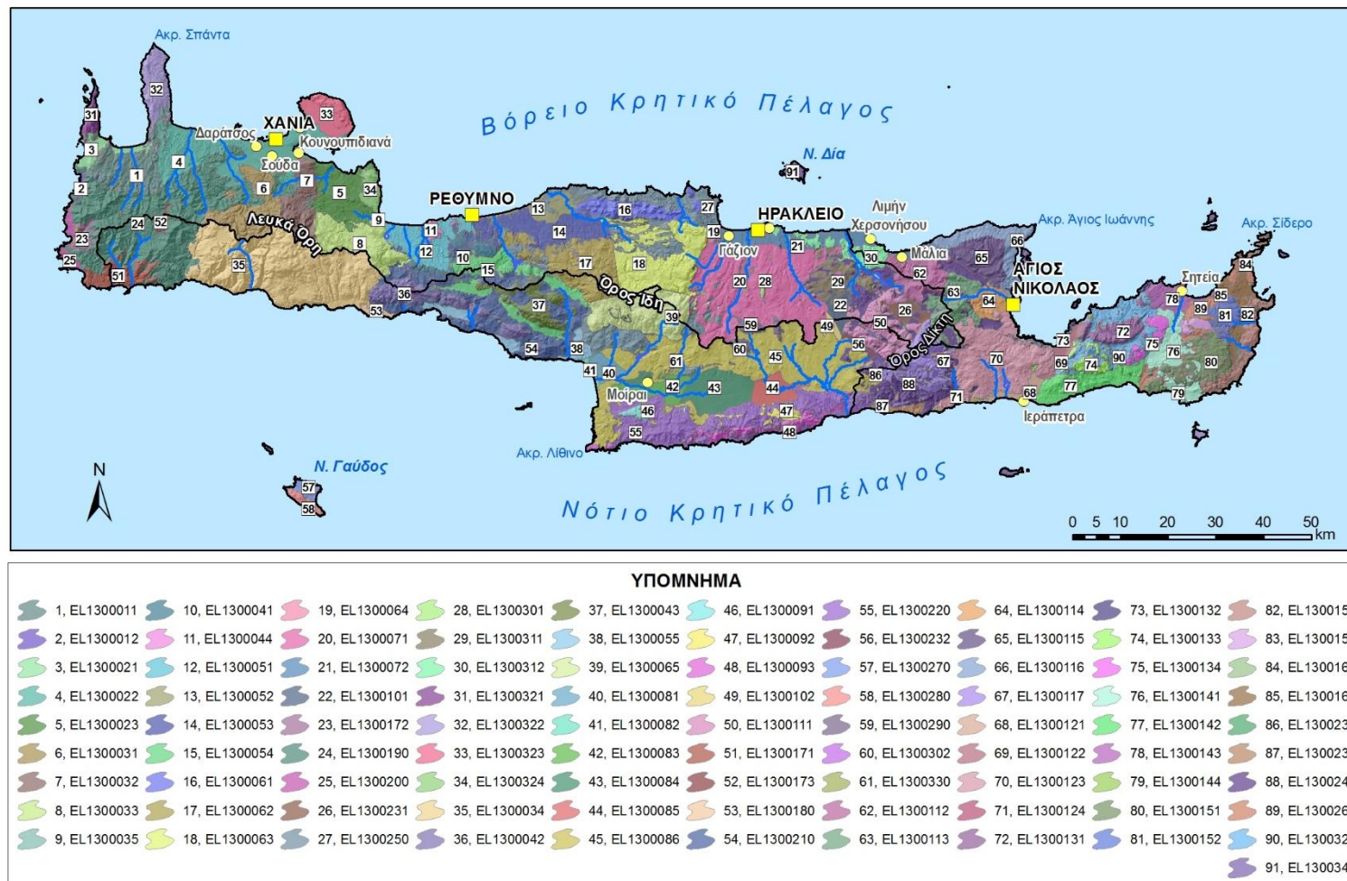
Εικόνα 2-4 Υπόγεια Υδατικά Συστήματα του ΥΔ Κρήτης
