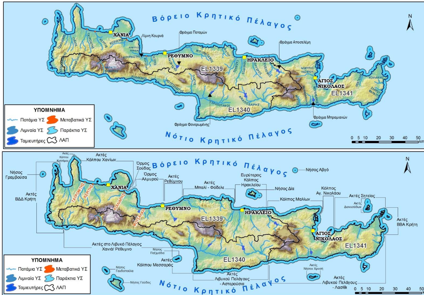
Εικόνα 2-3 Λεκάνες Απορροής Ποταμών και επιφανειακά Υδατικά Συστήματα ΥΔ Κρήτης
