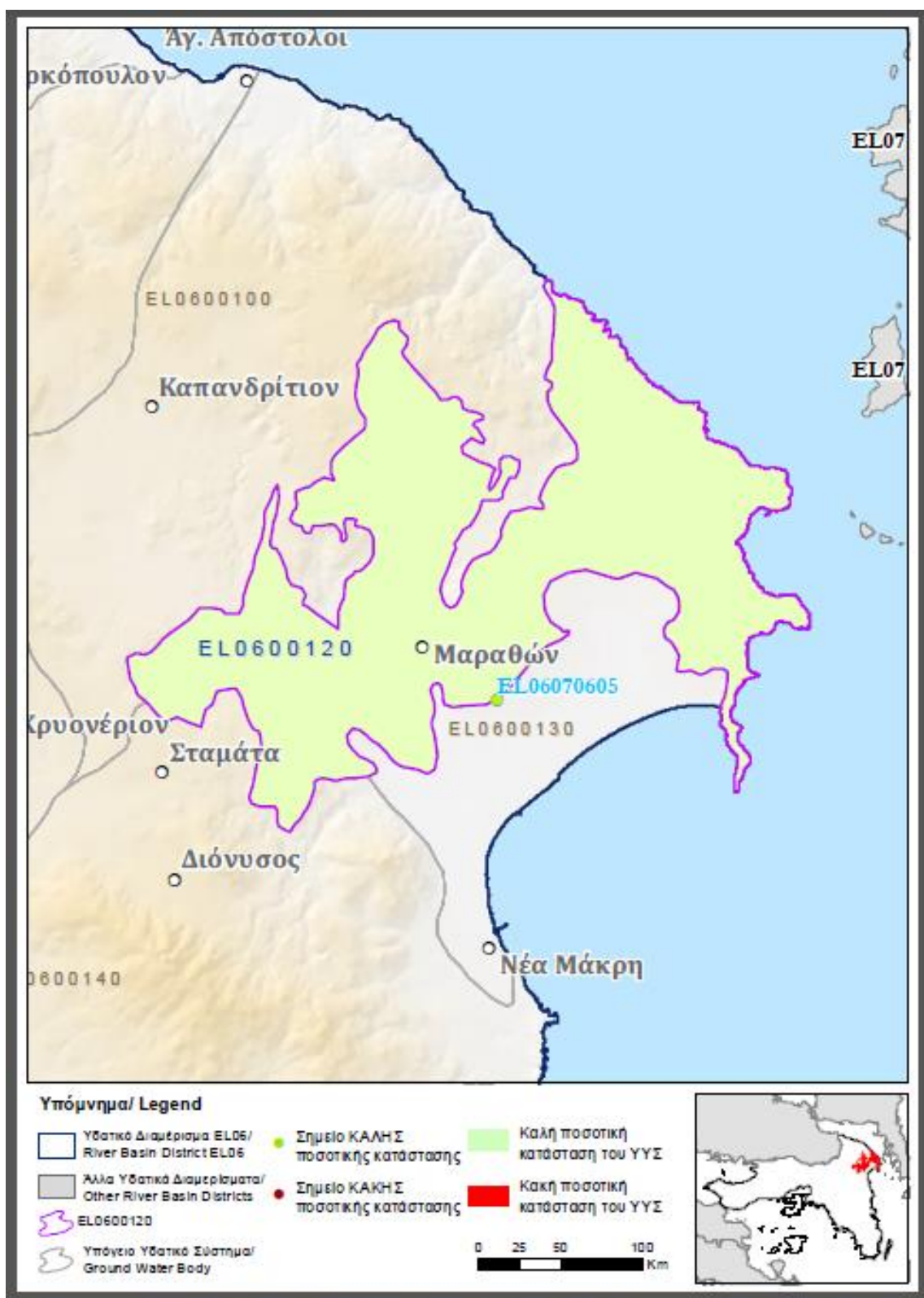
Εικόνα 6-12 Χάρτης ποσοτικής κατάστασης ΥΥΣ ΕΛ0600120
