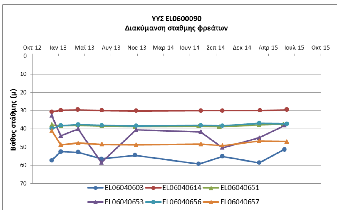
Σχήμα 6-7 Διάγραμμα διακύμανσης στάθμης υδροσημείων ΥΥΣ ΕΛ0600090
