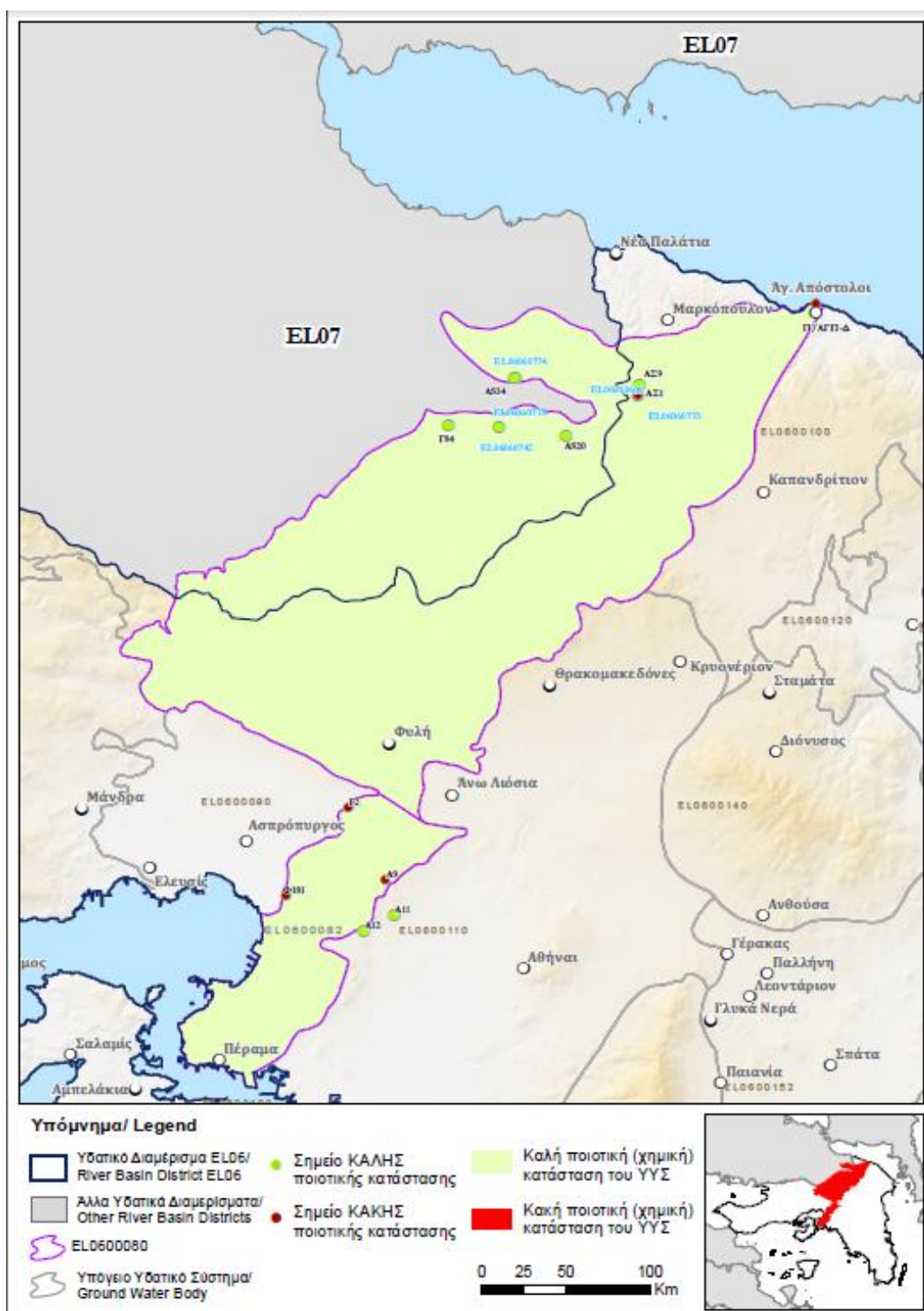
Εικόνα 5-28 Χάρτης ποιοτικής (χημικής) κατάστασης ΥΥΣ ΕΛ0600080
