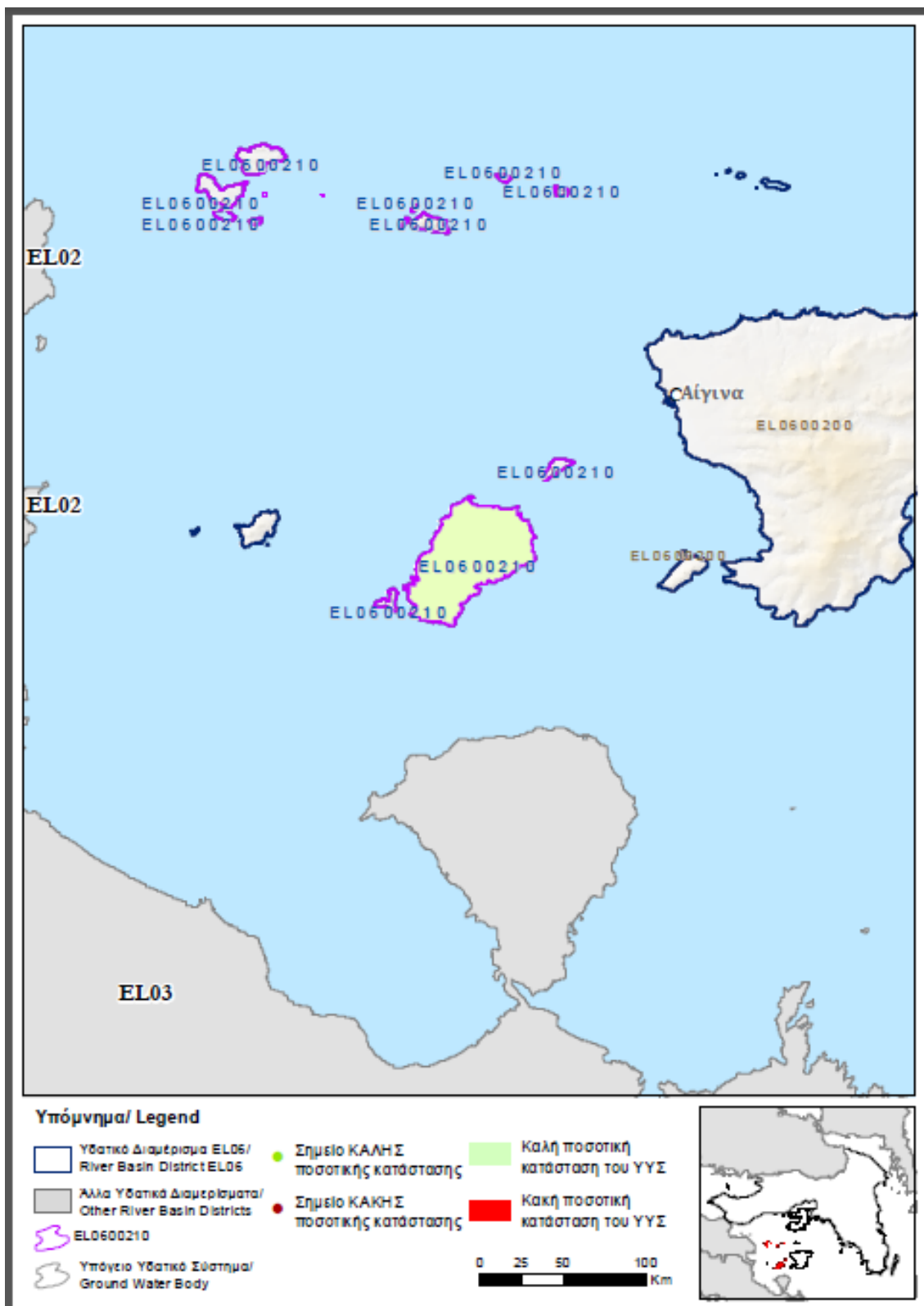
Εικόνα 6-21 Χάρτης ποσοτικής κατάστασης νέου ΥΥΣ EL0600210
