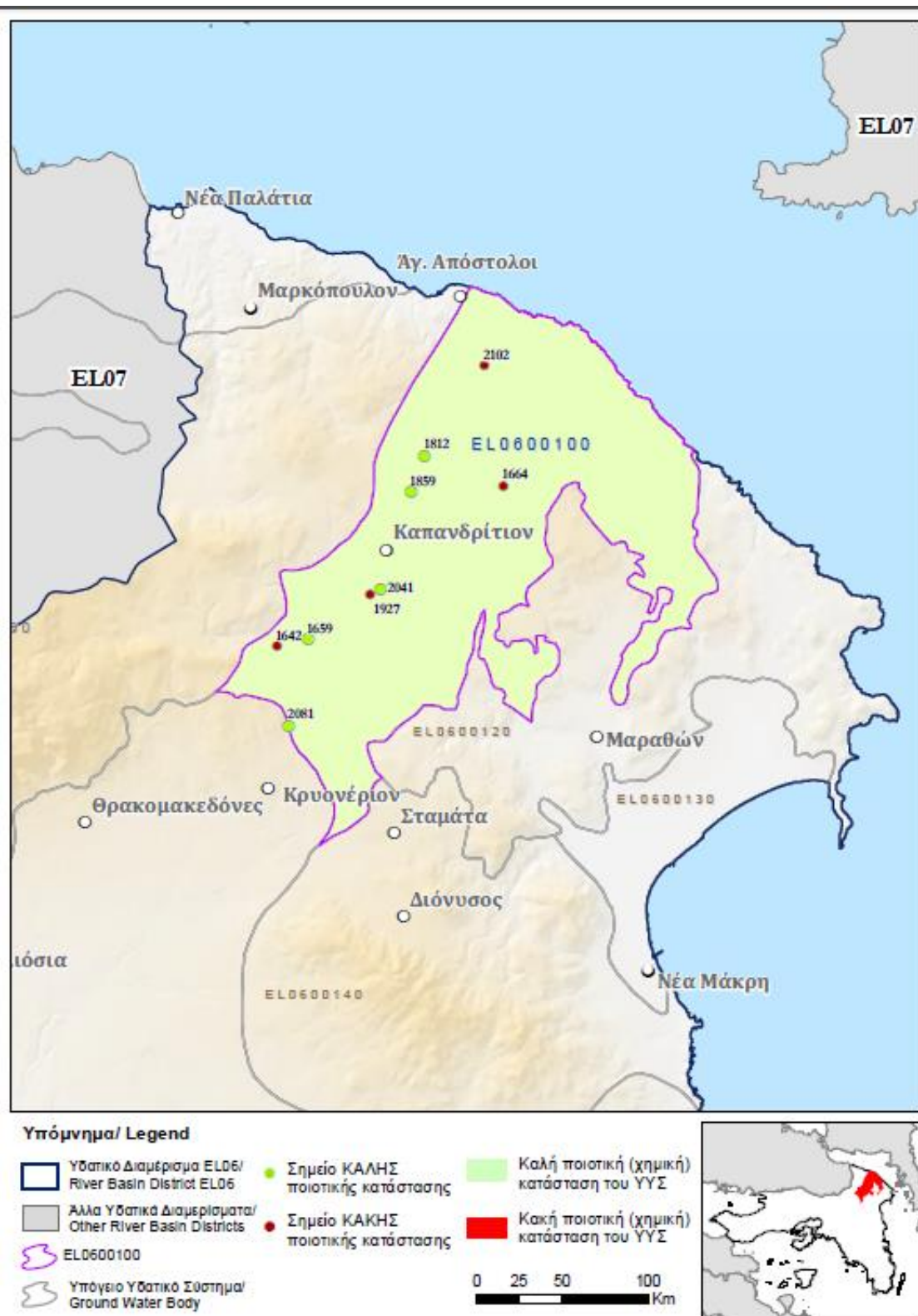
Εικόνα 5-34 Χάρτης ποιοτικής (χημικής) κατάστασης ΥΥΣ EL0600100
