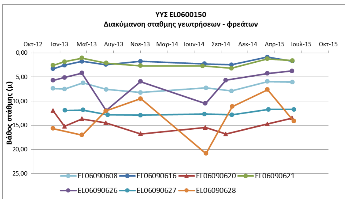
Σχήμα 6-11 Διάγραμμα διακύμανσης στάθμης γεωτρήσεων ΥΥΣ ΕΛ0600150
