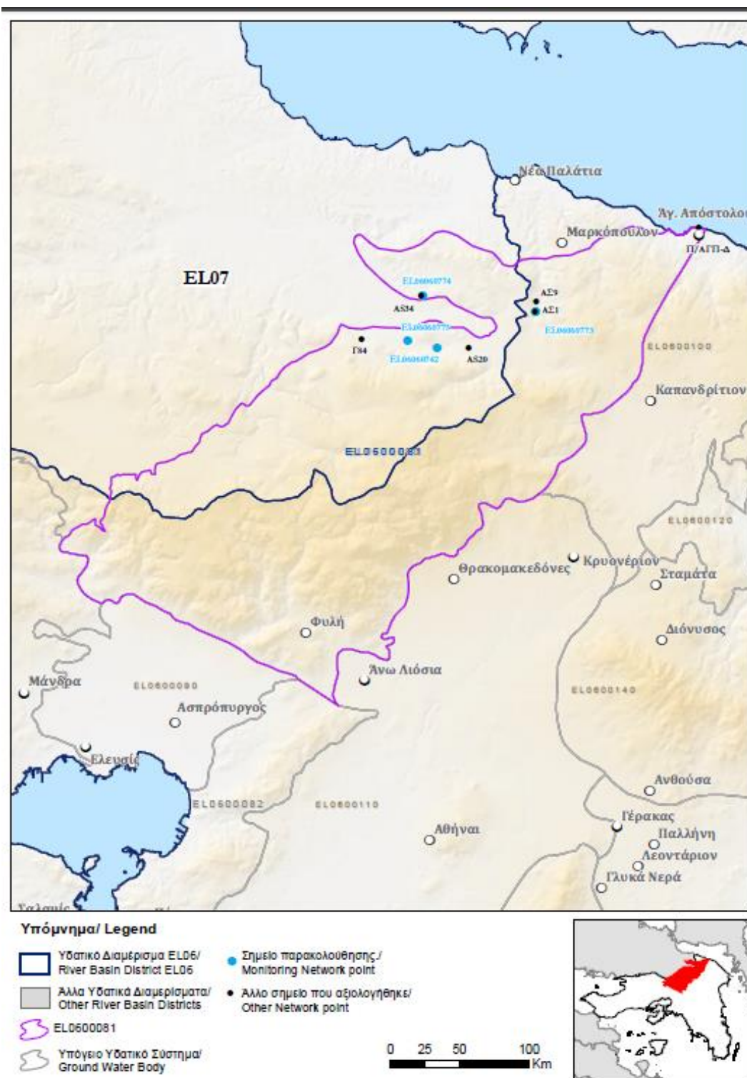
Εικόνα 5-24 Σημεία παρακολούθησης χημικής κατάστασης Υποσυστήματος ΕΛ0600081
