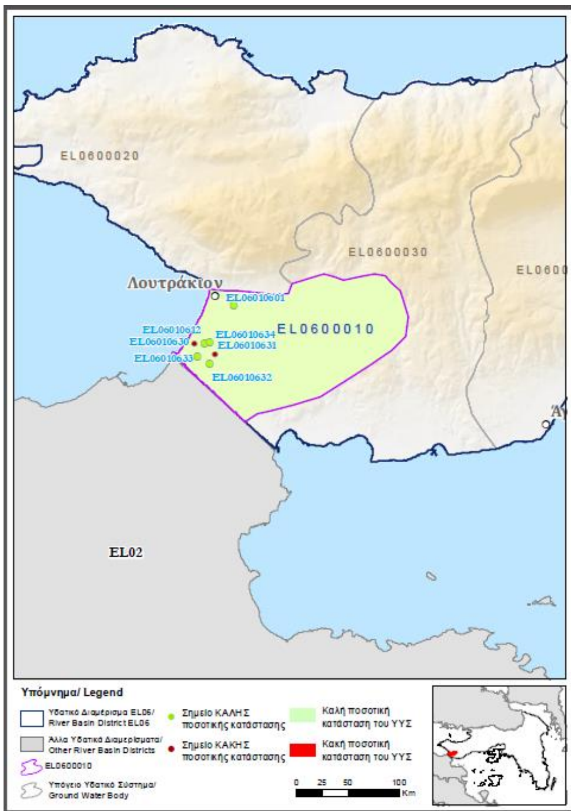
Εικόνα 6-1 Χάρτης ποσοτικής κατάστασης ΥΥΣ ΕΛ0600010
