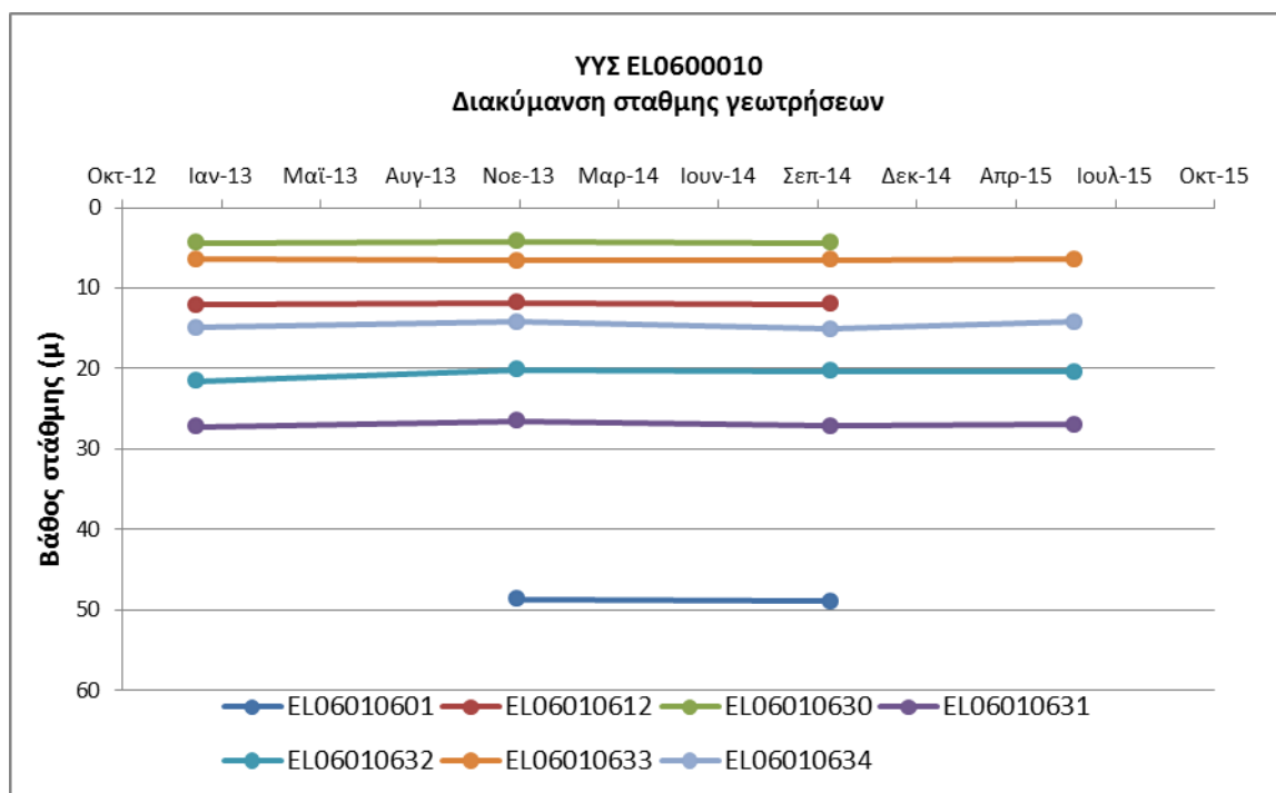
Σχήμα 6-1 Διάγραμμα διακύμανσης στάθμης υδροσημείων ΥΥΣ ΕΛ0600010
