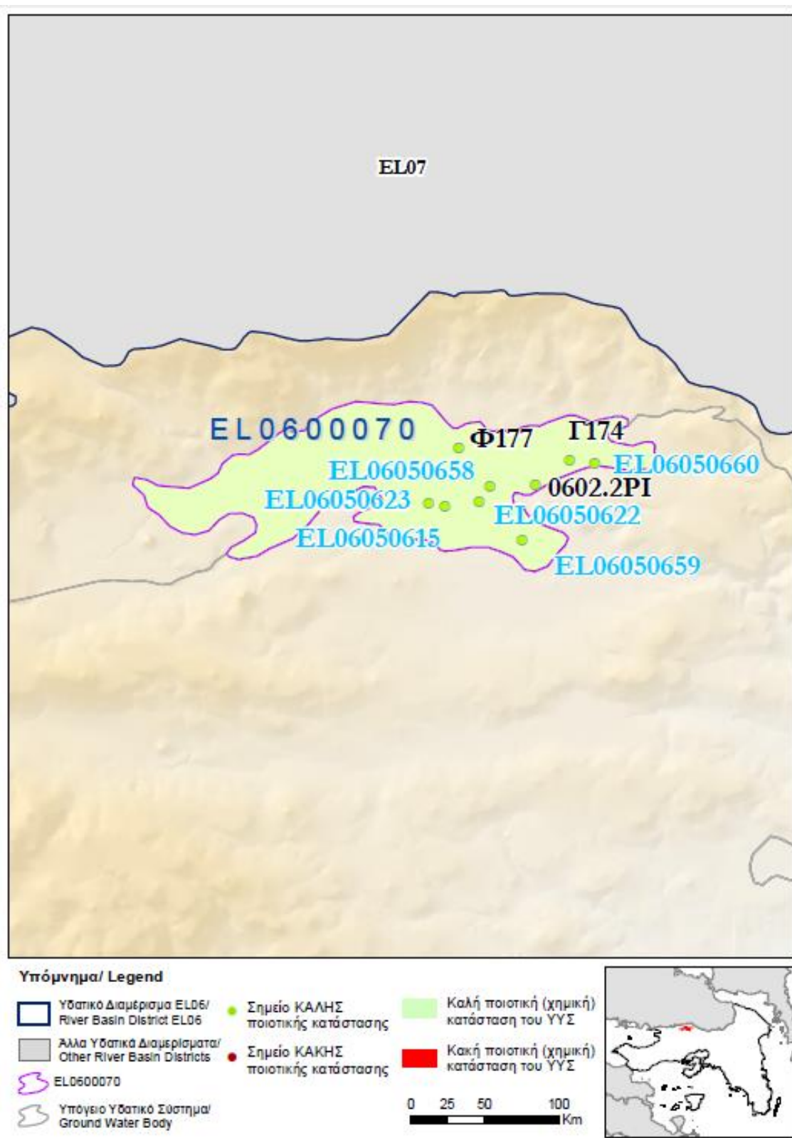
Εικόνα 5-22 Χάρτης ποιοτικής (χημικής) κατάστασης ΥΥΣ EL0600070
