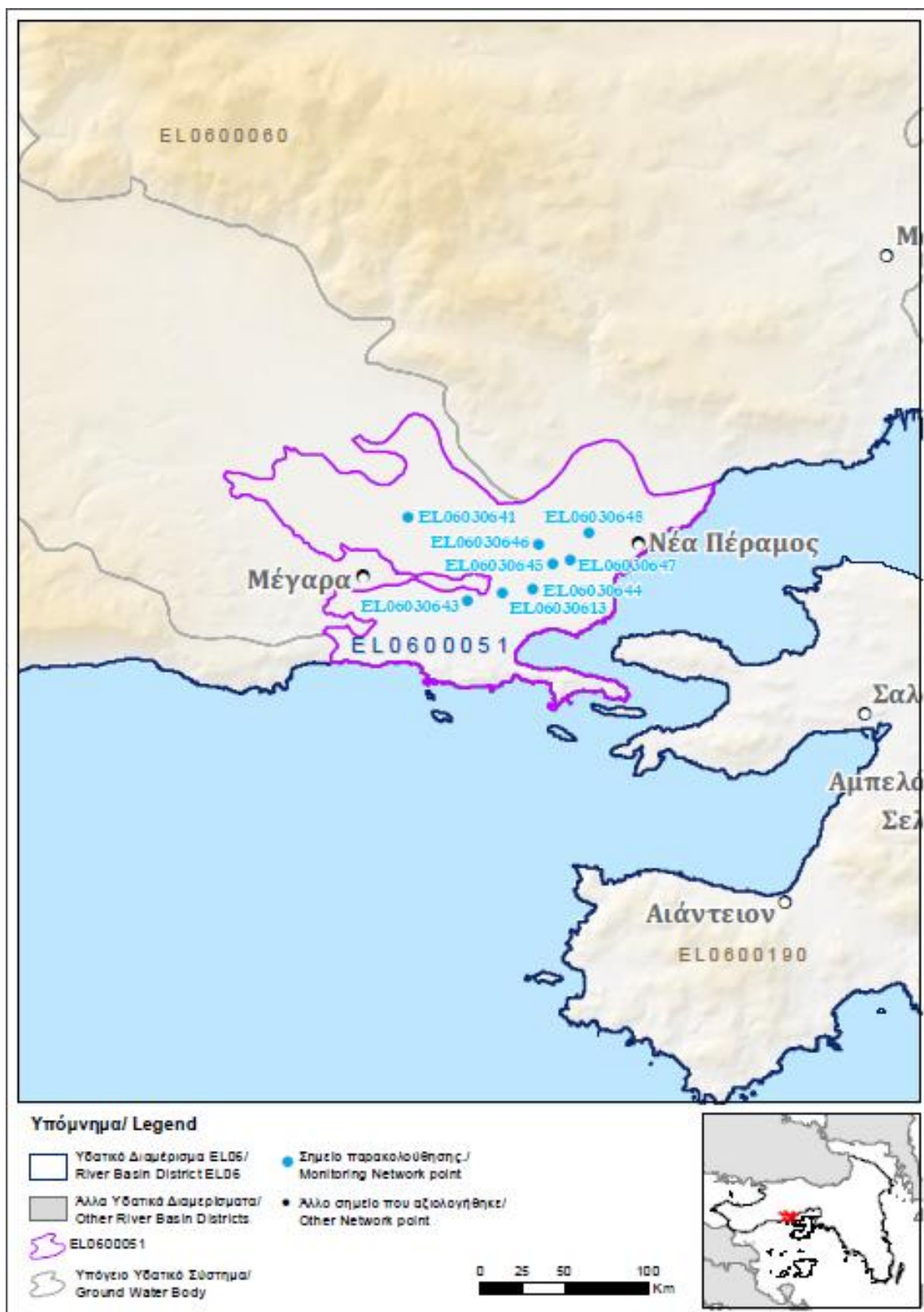
Εικόνα 5-13 Σημεία παρακολούθησης χημικής κατάστασης Υποσυστήματος ΕΛ0600051
