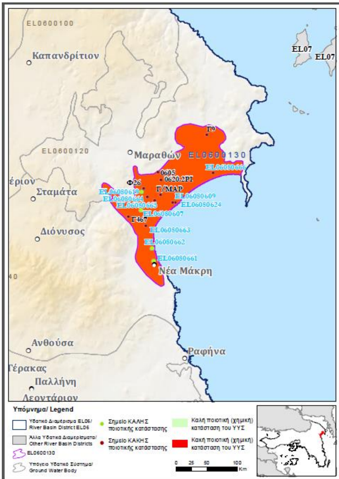
Εικόνα 5-45 Χάρτης ποιοτικής (χημικής) κατάστασης ΥΥΣ ΕΛ0600130
