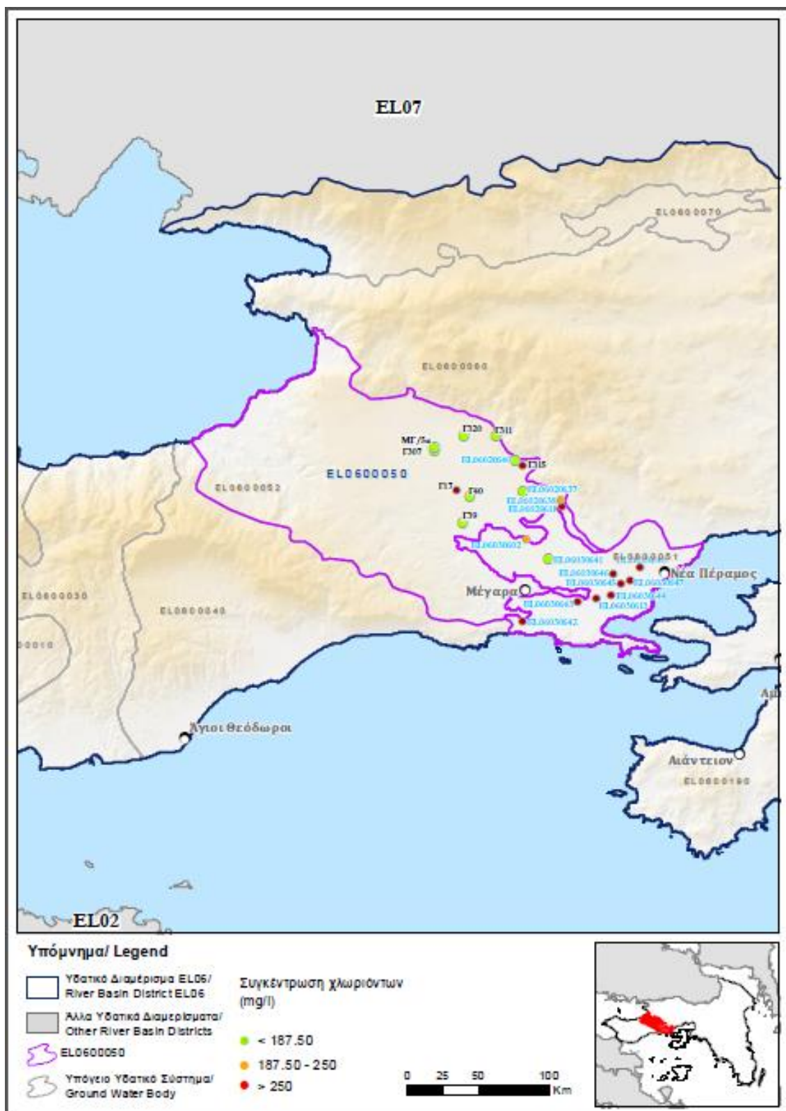
Εικόνα 5-15 Χάρτης κατανομής συγκεντρώσεων χλωριόντων στο νερό του ΥΥΣ ΕΛ0600050
