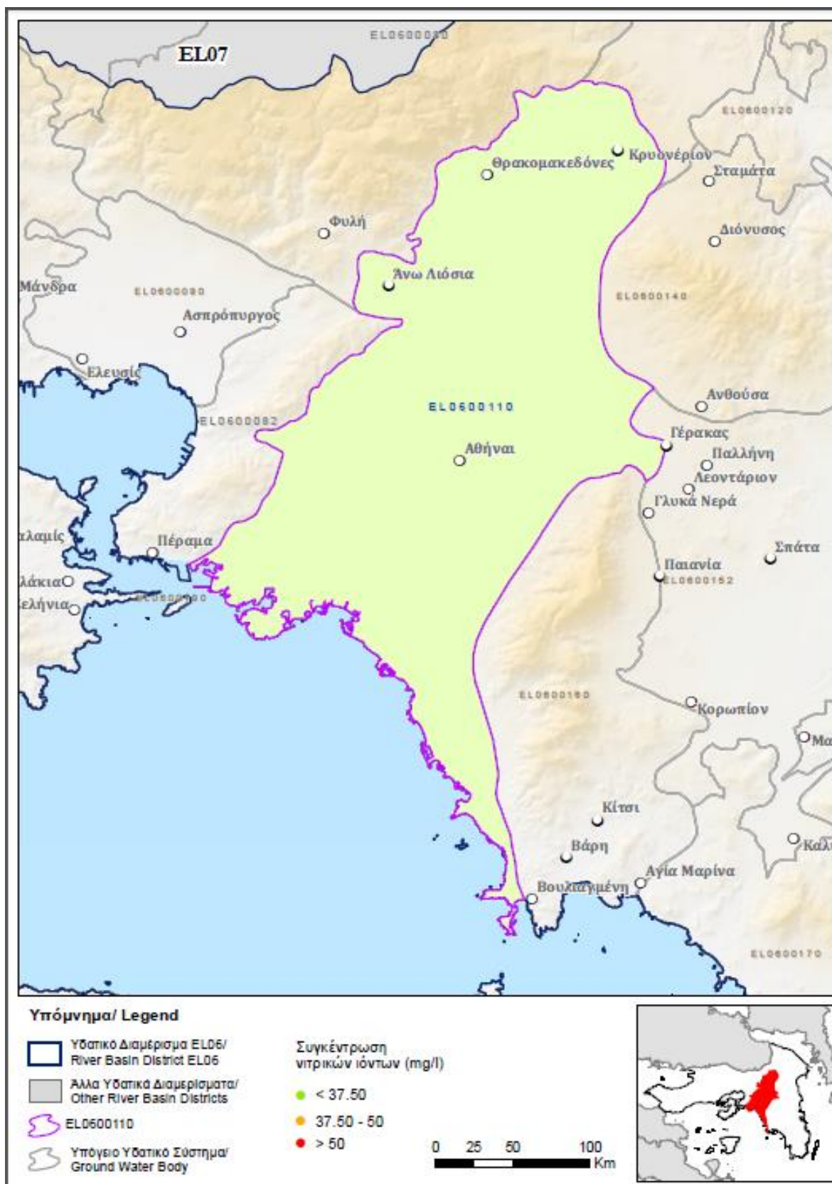
Εικόνα 6-11 Χάρτης ποσοτικής κατάστασης ΥΥΣ EL0600110
