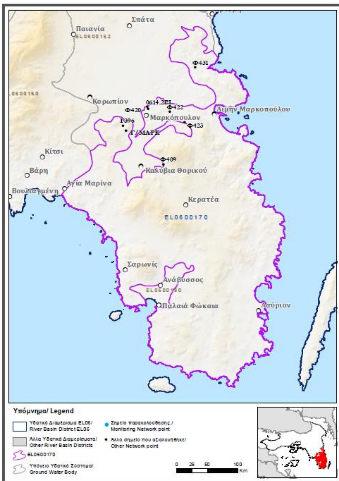
Εικόνα 5-57 Σημεία παρακολούθησης χημικής κατάστασης ΥΥΣ EL0600170
