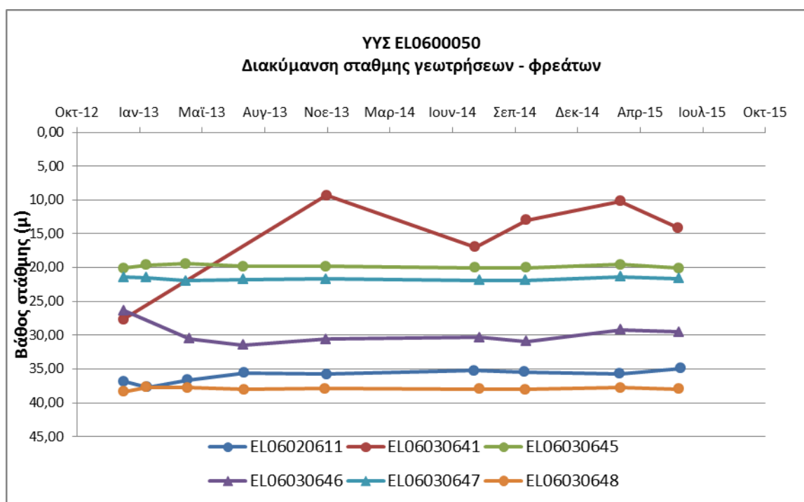
Σχήμα 6-3 Διάγραμμα διακύμανσης στάθμης υδροσημείων ΥΥΣ ΕΛ0600050
