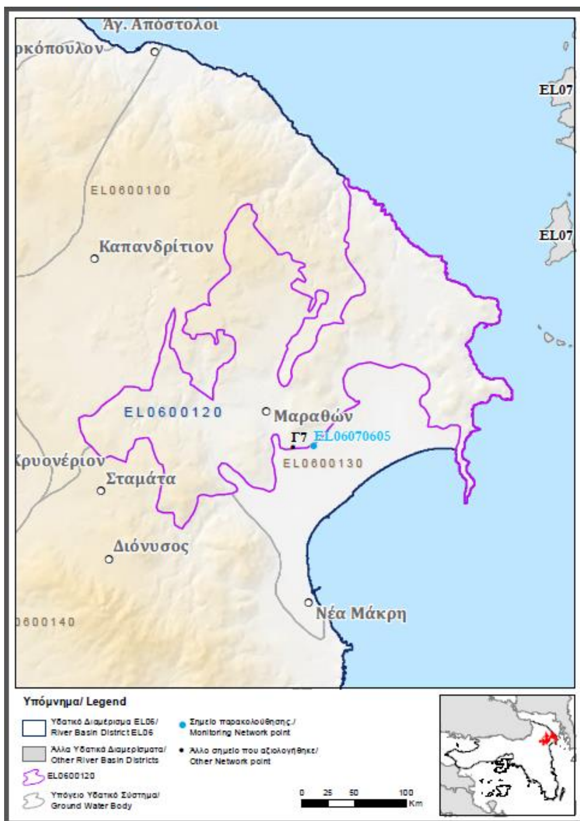
Εικόνα 5-39 Σημεία παρακολούθησης χημικής κατάστασης ΥΥΣ ΕΛ0600120
