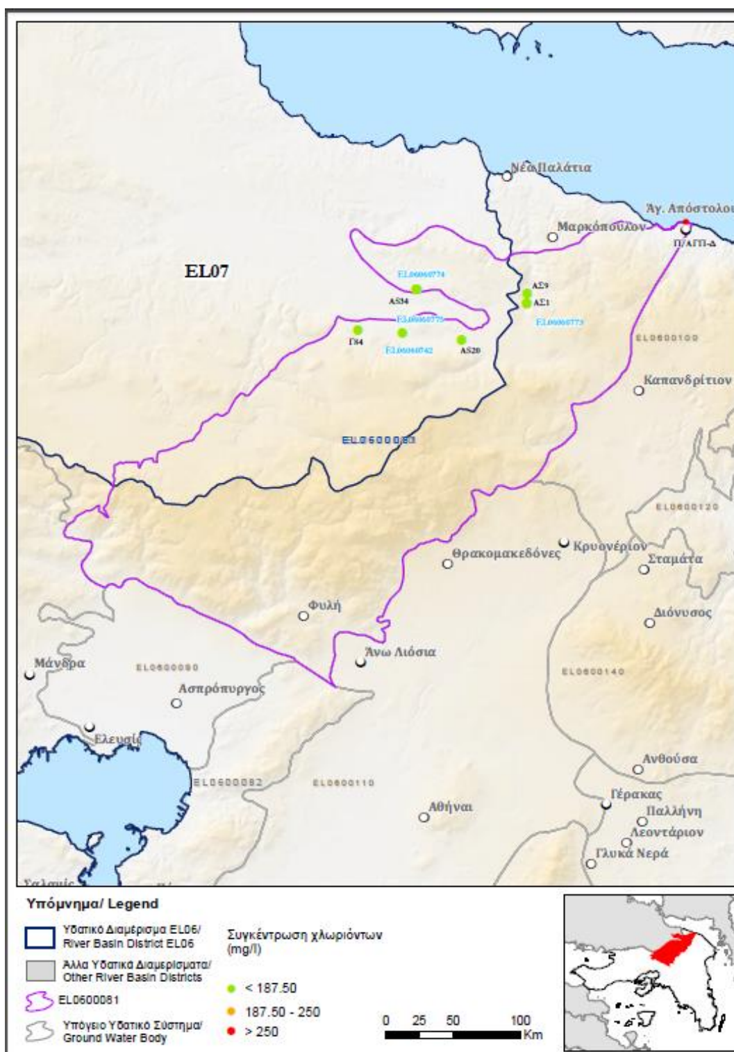
Εικόνα 5-26 Χάρτης κατανομής συγκεντρώσεων χλωριόντων υποσυστήματος EL0600081
