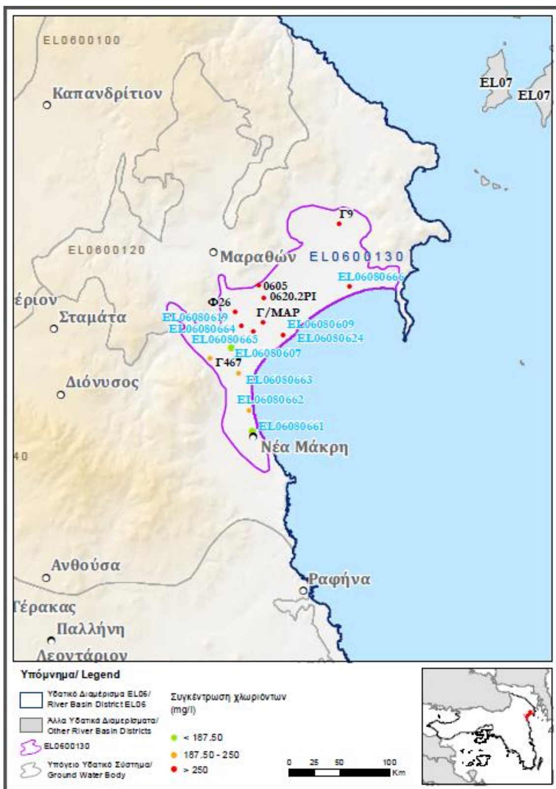
Εικόνα 5-43 Χάρτης κατανομής συγκεντρώσεων χλωριόντων στο νερό του ΥΥΣ EL0600130
