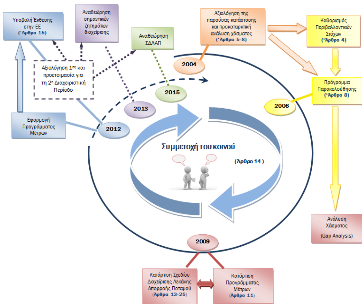
Σχήμα 0-1 Σχηματικό διάγραμμα βημάτων κατάρτισης Σχεδίων Διαχείρισης Λεκάνης Απορροής Ποταμών
