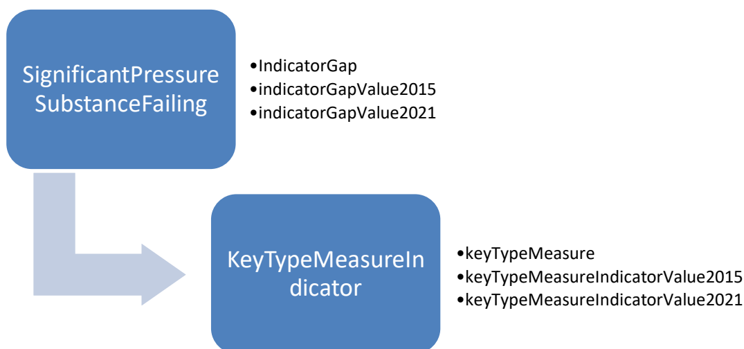
Σχήμα 0-1 Σηματικό διάγραμμα σχέσης μεταξύ πιέσεων και BTM
