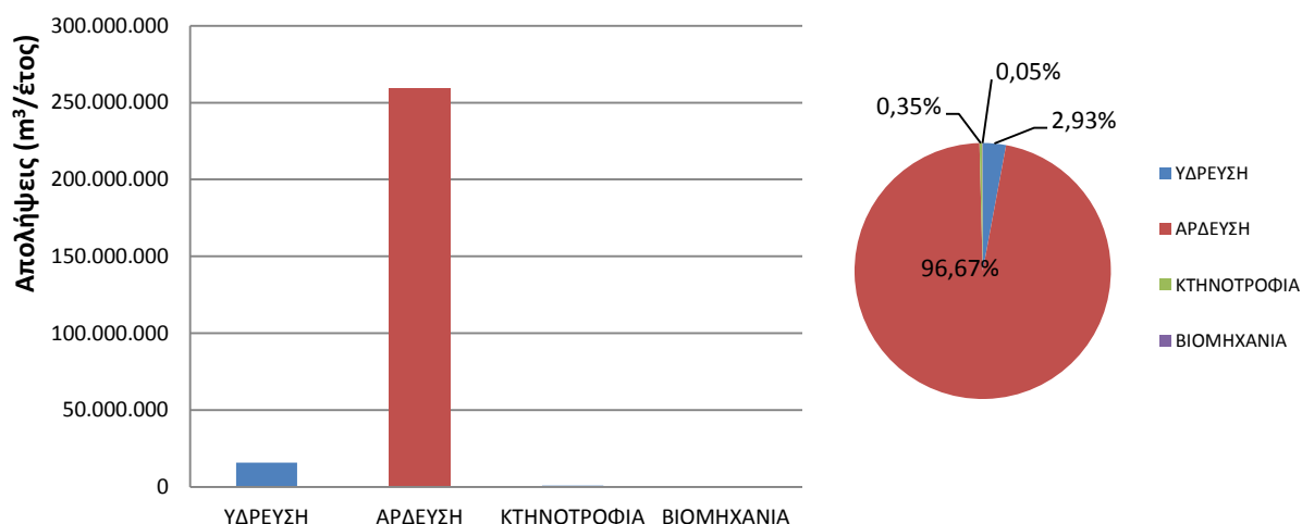
Σχήμα 5-16: Ποσότητες και κατανομή ετήσιων απολήψεων νερού στη ΛΑΠ Νέστου (ΕΛ1207)
