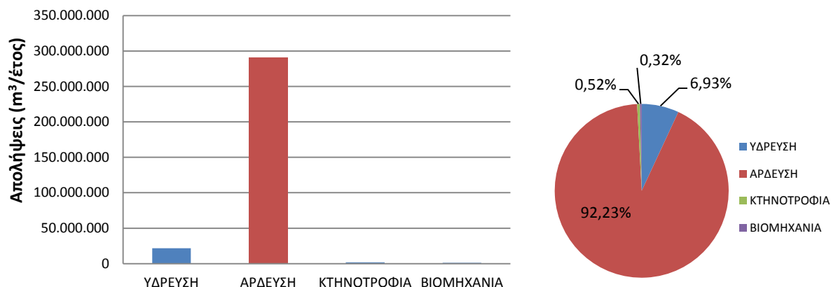
Σχήμα 5-19: Ποσότητες και κατανομή ετήσιων απολήψεων νερού στη ΛΑΠ Έβρου (EL1210)
