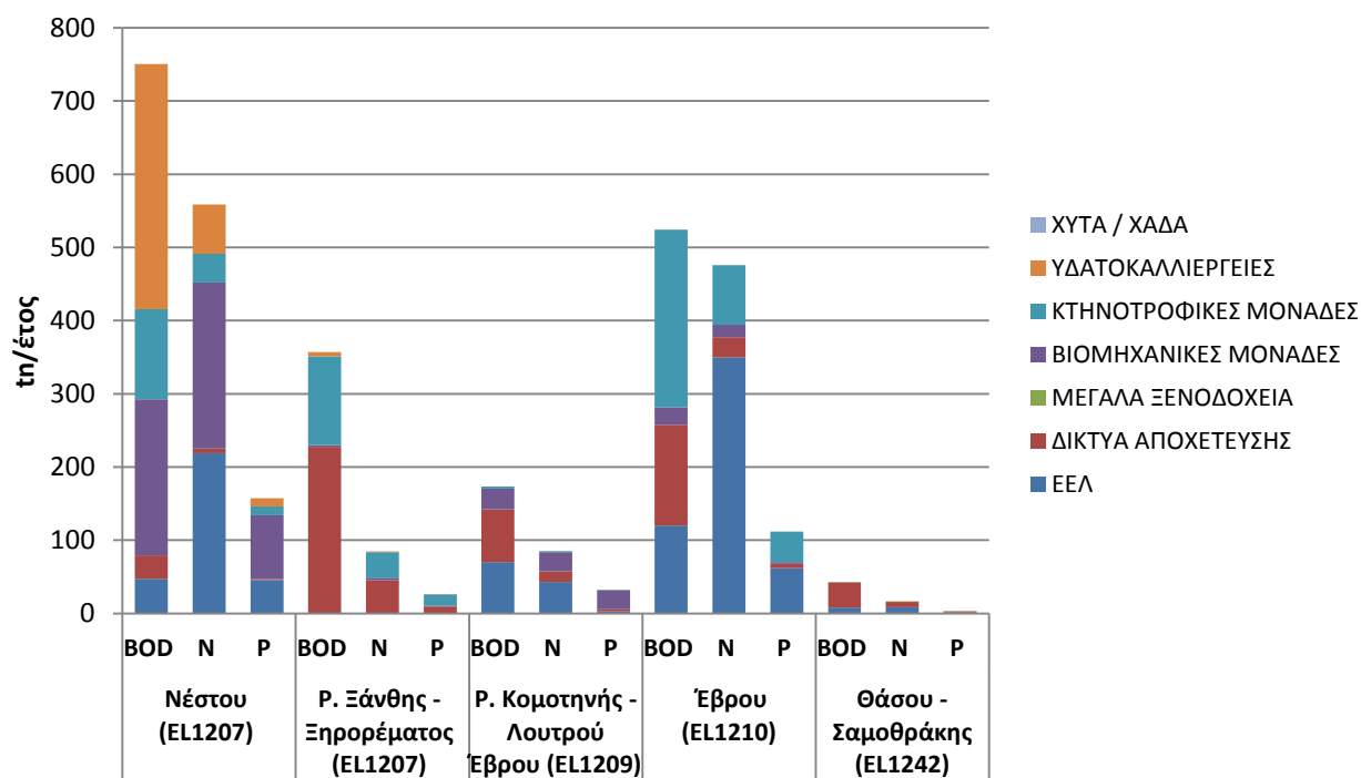
Σχήμα 5-1: Συνολικά ετήσια φορτία BOD, N και P που παράγονται στις επιμέρους ΛΑΠ του ΥΔ Θράκης (EL12) από σημειακές πηγές ρύπανσης
