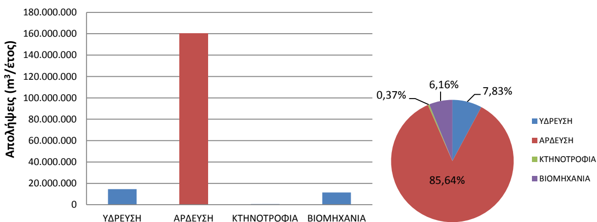
Σχήμα 5-18: Ποσότητες και κατανομή ετήσιων απολήψεων νερού στη ΛΑΠ Ρ. Κομοτηνής - Λουτρού Έβρου (EL1209)
