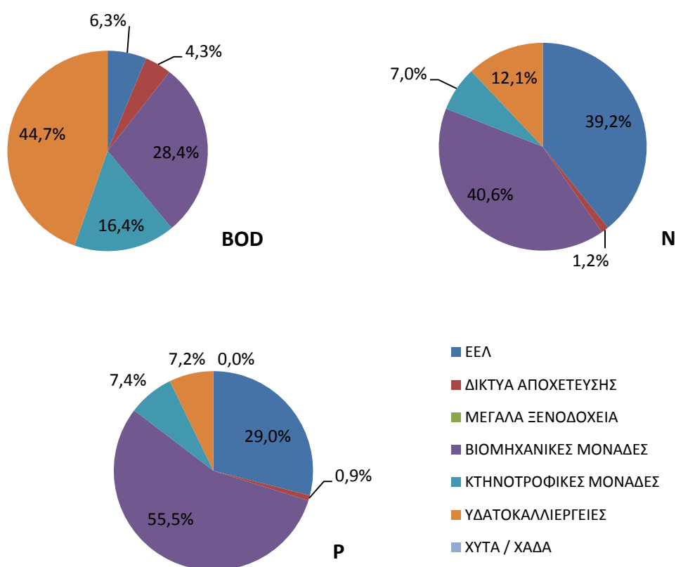
Σχήμα 5-2: Κατανομή ετήσιας επιβάρυνσης BOD, N και P από σημειακές πιέσεις στη ΛΑΠ Νέστου (EL1207) του ΥΔ Θράκης (EL12)
