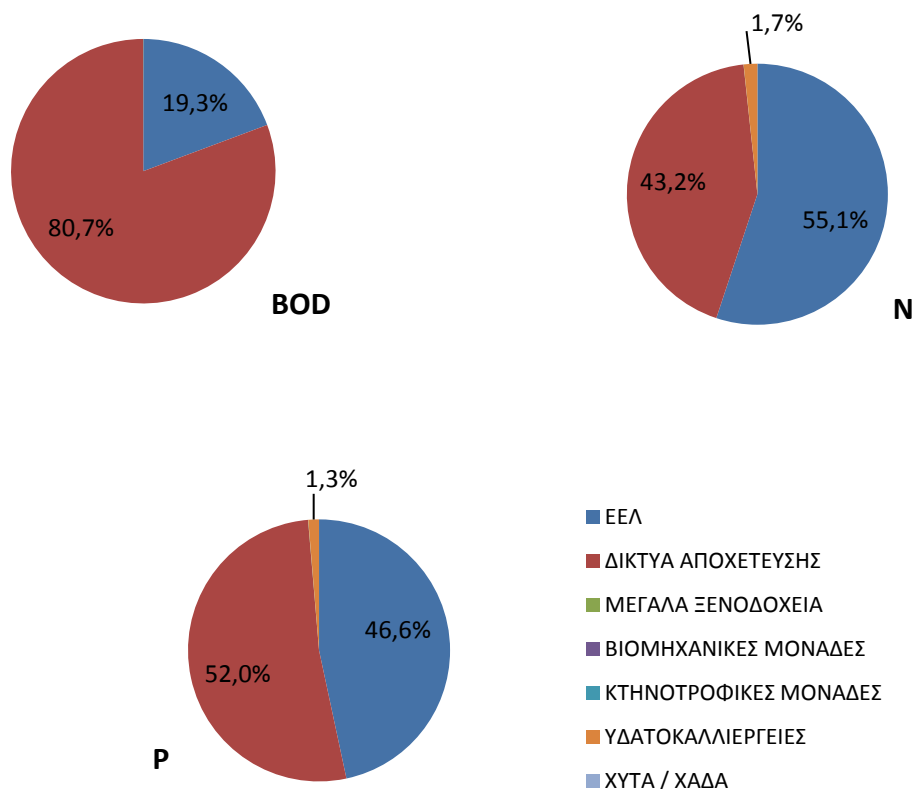
Σχήμα 5-6: Κατανομή ετήσιας επιβάρυνσης BOD, N και P από σημειακές πιέσεις στη ΛΑΠ Θάσου – Σαμοθράκης (EL1242) του ΥΔ Θράκης (EL12)
