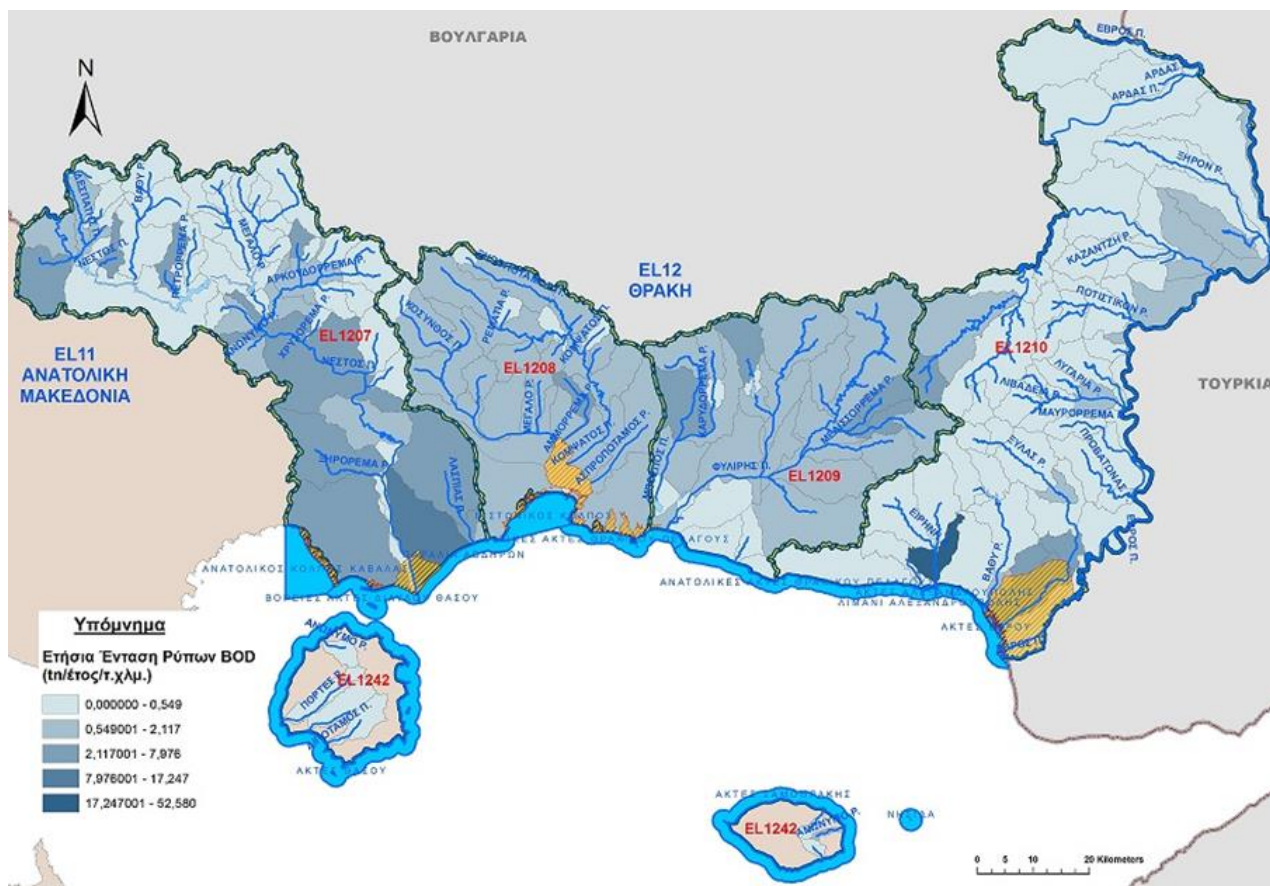
Σχήμα 5-15: Τελική ετήσια επιφανειακή ένταση ρύπων BOD, N και P (τόνοι/έτος/χλμ 2 ) από διάχυτες πηγές ρύπανσης για τις ΛΑΠ του ΥΔ Θράκης (EL12)
