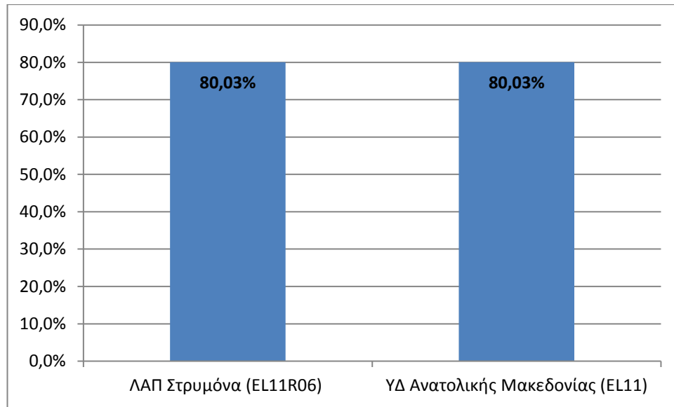
Σχήμα 7-3: Ανάκτηση χρηματοοικονομικού κόστους παροχής νερού για βιομηχανική χρήση στη ΛΑΠ του ΥΔ EL11
