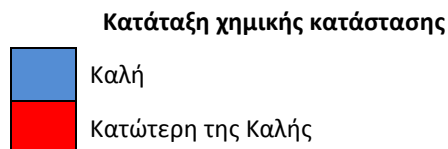
Σχήμα 6-4: Κατηγορίες αξιολόγησης της χημικής κατάστασης επιφανειακών ΥΣ
