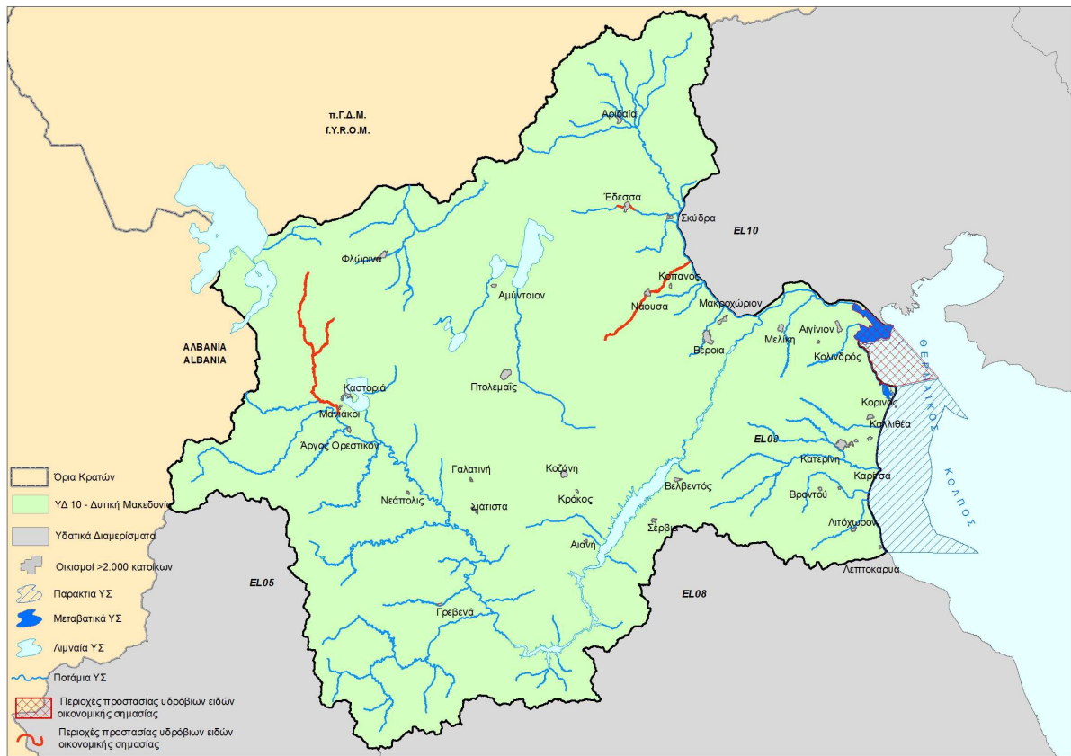
Χάρτης 13: ΥΣ Προστασίας υδρόβιων ειδών με οικονομική σημασία
