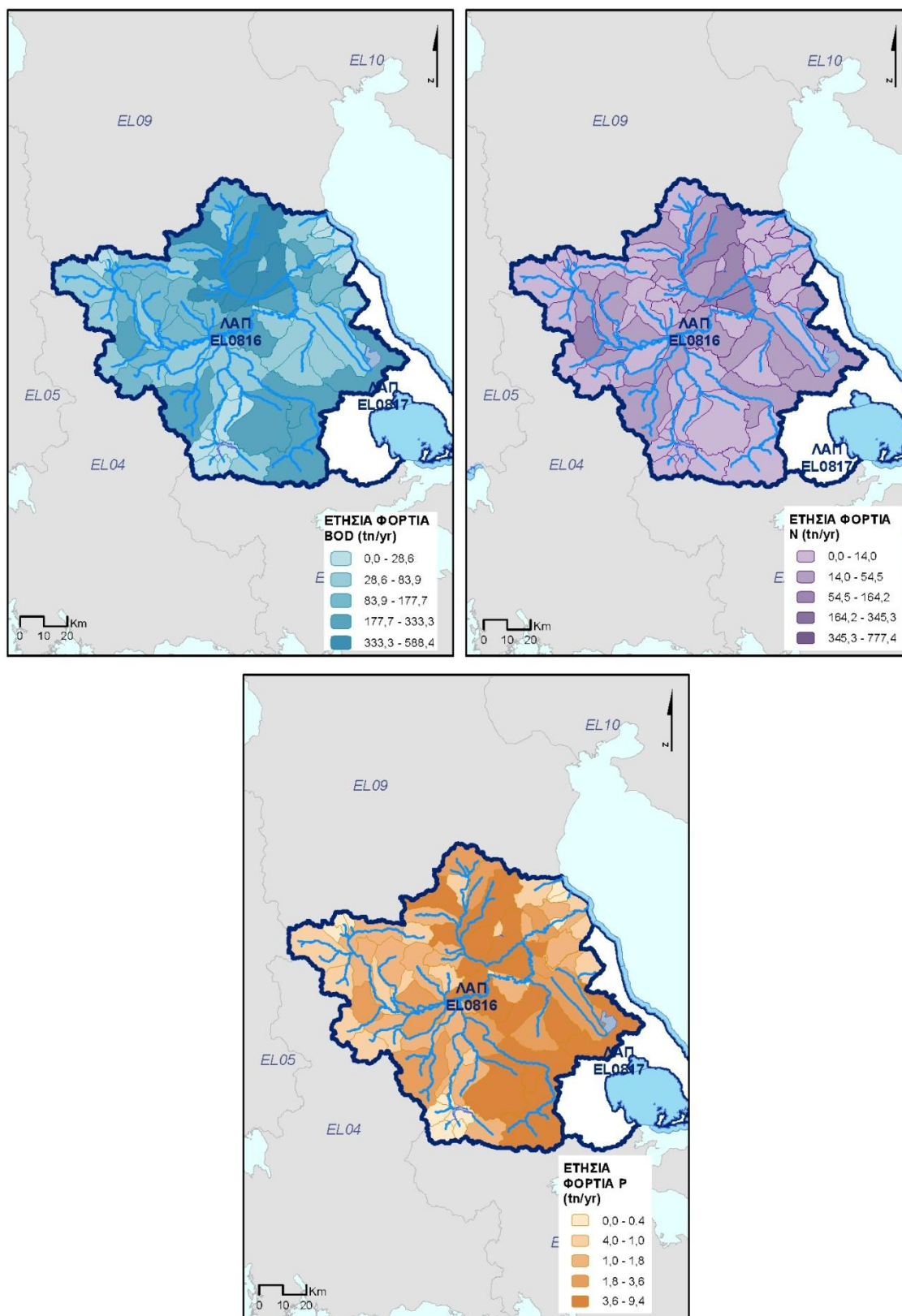
Χάρτης 20: Τελική ετήσια επιφανειακή ποσότητα ρύπων BOD, N και P (τόνοι/έτος) από διάχυτες πηγές ρύπανσης για τη ΛΑΠ Πηνειού (EL0816)
