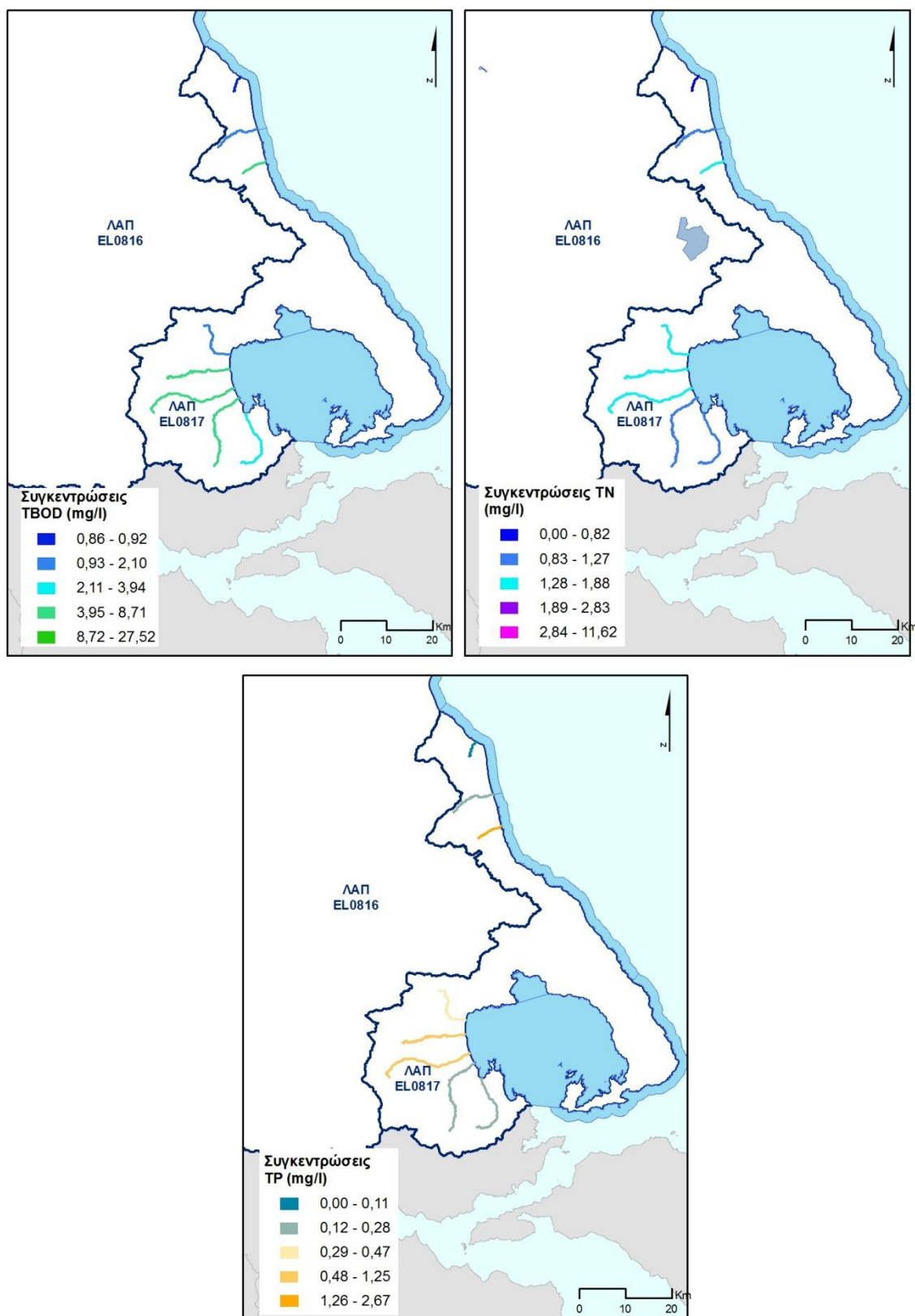
Χάρτης 25: Ετήσια διάλυση ρύπων BOD, N και P (mg/l) από το σύνολο των πηγών ρύπανσης για τη ΛΑΠ Αλμυρού-Πηλίου (EL0817)
