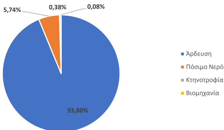
Σχήμα 5-8: Κατανομή ετήσιων απολήψεων ύδατος στη ΛΑΠ Πηνειού (EL0816)
