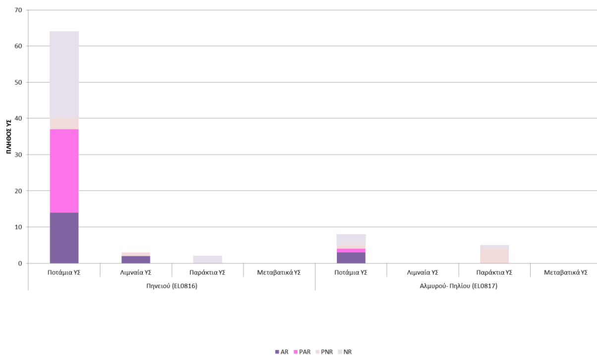
Σχήμα 5-13: Εκτίμηση κινδύνου μη επίτευξης στόχων επιφανειακών υδατικών συστημάτων στις Λεκάνες Απορροής Ποταμών (EL0816) και (EL0817)
