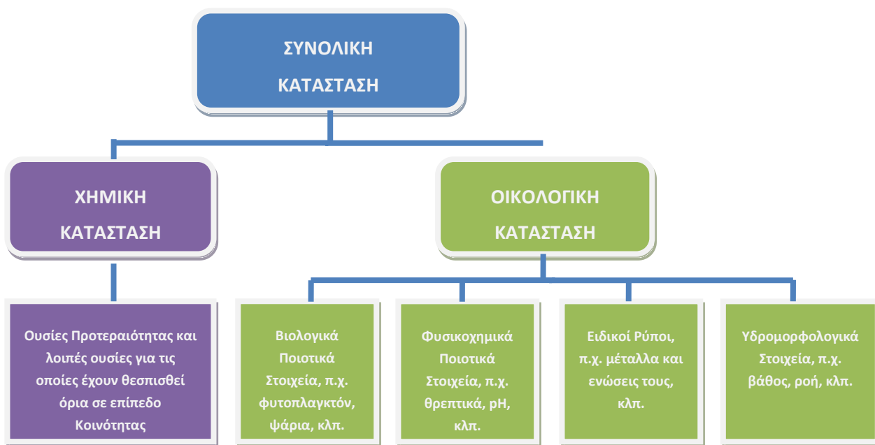
Σχήμα 6-1: Κατηγορίες ποιοτικών στοιχείων που χρησιμοποιούνται για την αξιολόγηση της κατάστασης των επιφανειακών υδατικών συστημάτων
