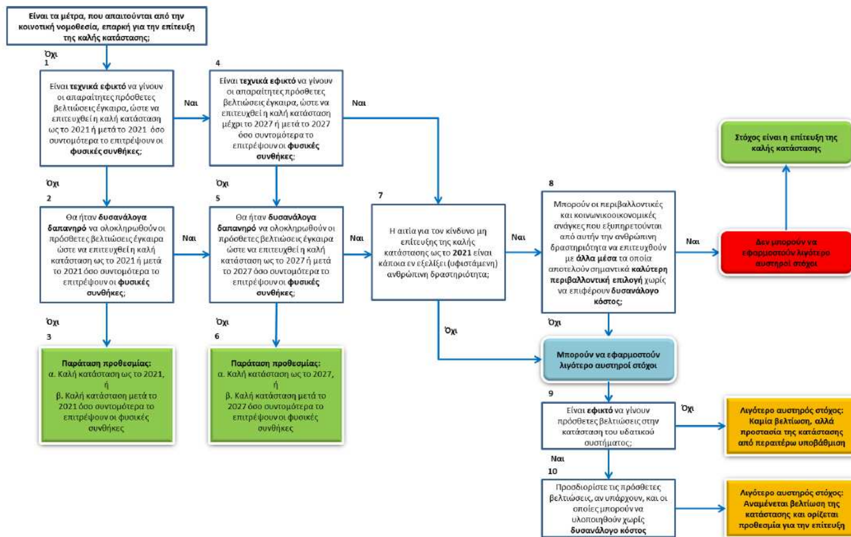
Σχήμα 4-25. Διαδικασία εφαρμογής εναλλακτικών στόχων στο πλαίσιο των Άρθρων 4.4 και 4.5 για τις ανάγκες της 1ης Αναθεώρησης του ΣΔΛΑΠ
