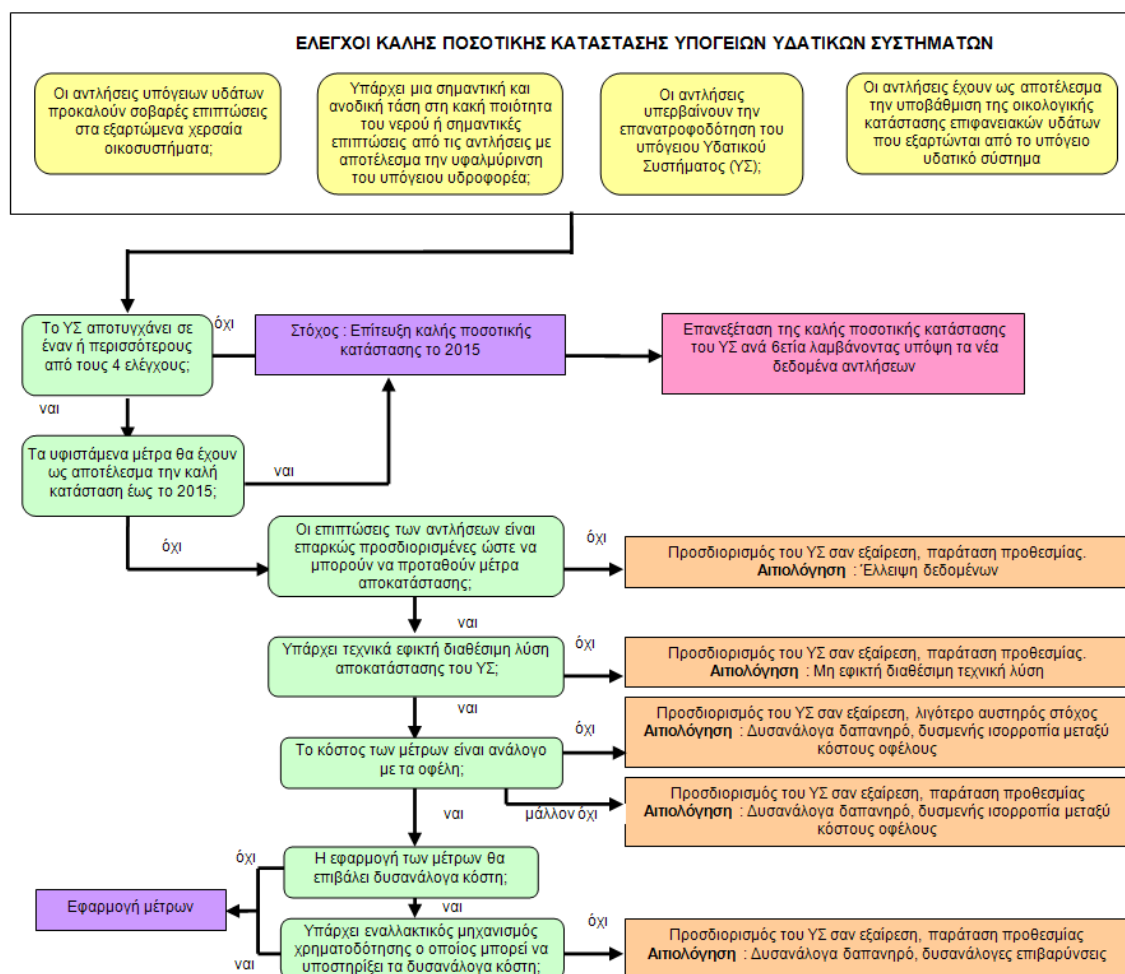
Σχήμα 4-24. Λογικό διάγραμμα καθορισμού των εξαιρέσεων στα υπόγεια ΥΣ
