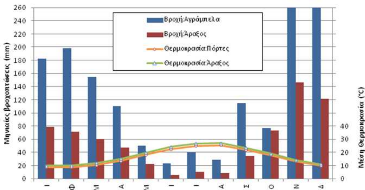
Σχήμα 6-17. Μέση μηνιαία βροχόπτωση και μέση μηνιαία θερμοκρασία σε σταθμούς της ΛΑΠ 28
