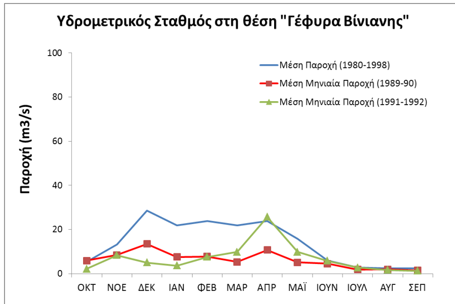
Σχήμα 8. Υδρομετρήσεις στη θέση «Γέφυρα Βίνιανης» στον π. Ταυρωπό
