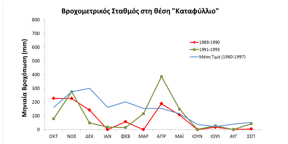
Σχήμα 3. Σύγκριση μηνιαίων βροχοπτώσεων περιόδου 1989-1993 με τη μέση τιμή της περιόδου 1980-1997 στη θέση «Καταφύλλιο»
