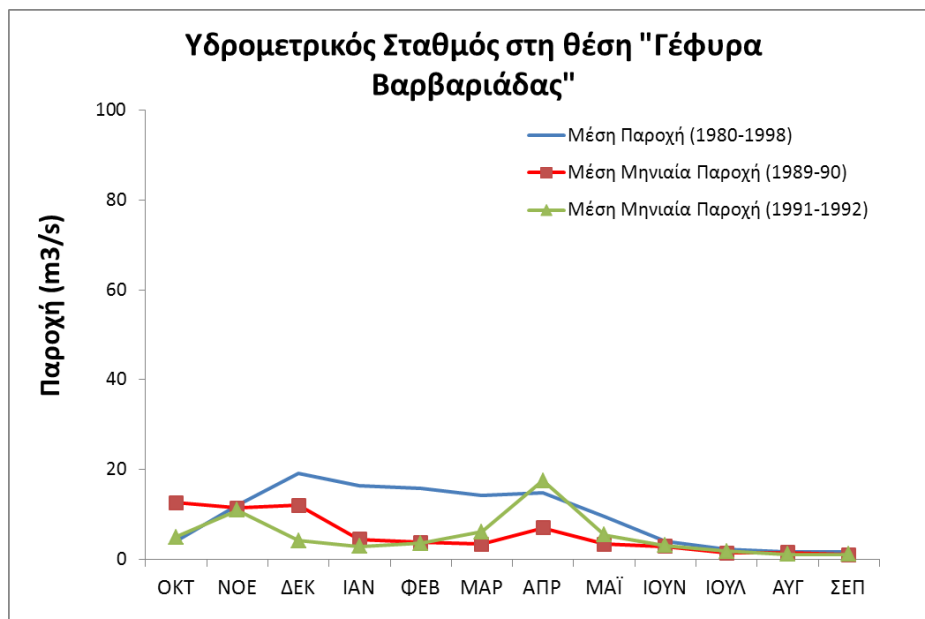
Σχήμα 7. Υδρομετρήσεις στη θέση «Γέφυρα Βαρβαριάδας» στον π. Αγραφιώτη
