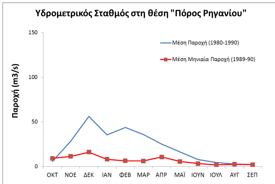
Σχήμα 9. Υδρομετρήσεις στη θέση «Πόρος Ρηγανίου» στον π. Εύηνο
