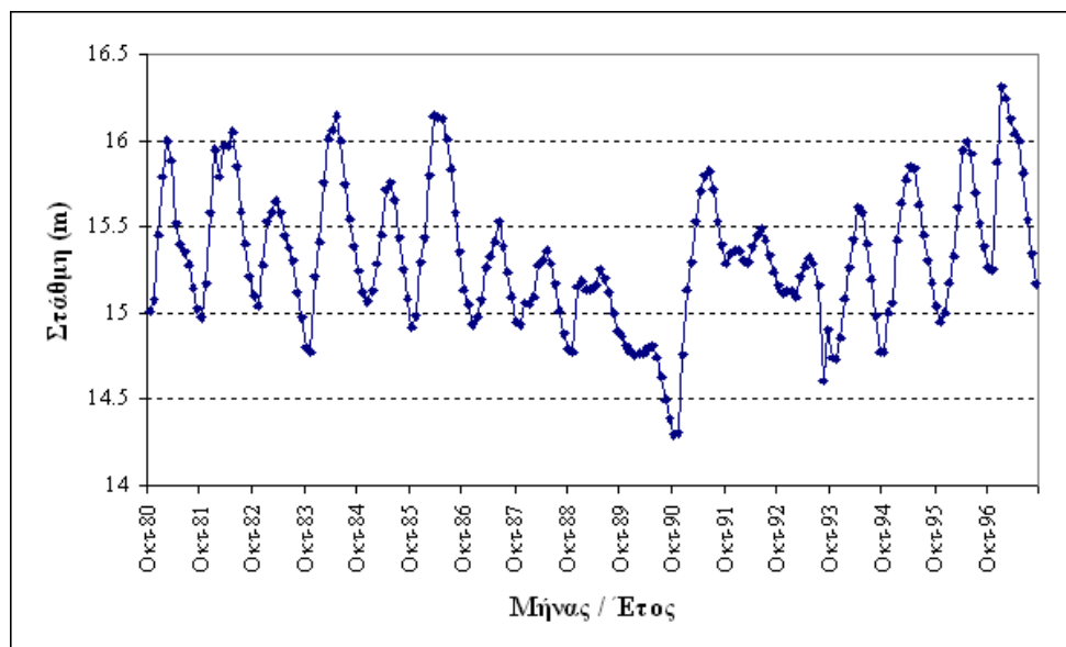
Σχήμα 16. Μέσες μηνιαίες αναγνώσεις της στάθμης στη λίμνη Τριχωνίδα
