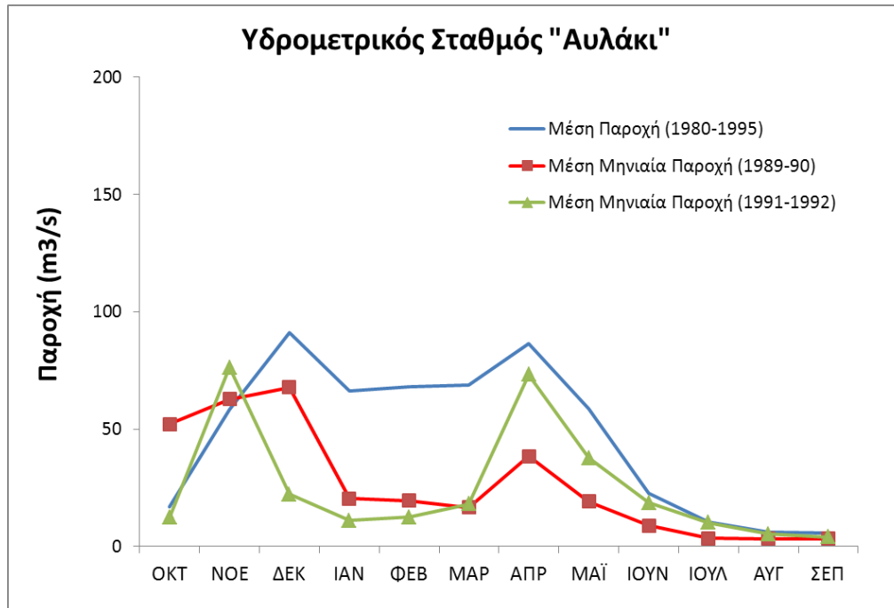
Σχήμα 6. Υδρομετρήσεις στη θέση «Αυλάκι» στον άνω Αχελώο
