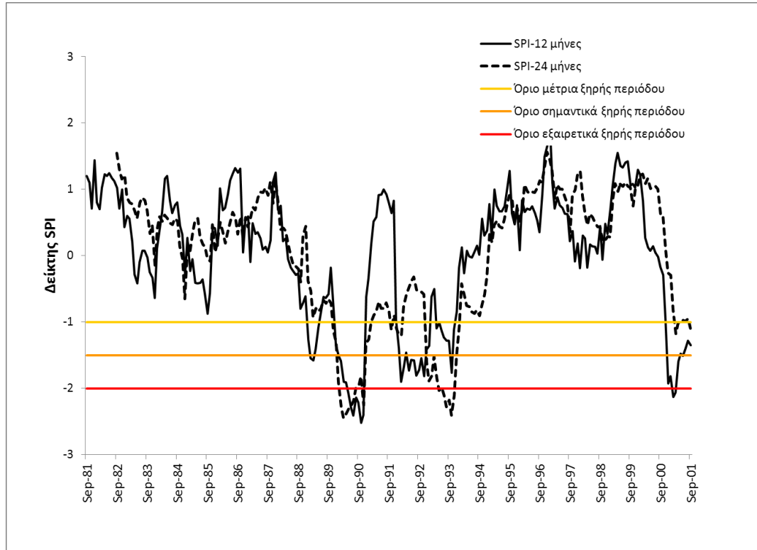
Σχήμα 19. Ο δείκτης SPI 12 και 24 μηνών με βάση τους σταθμούς ΥΠΕΚΑ στο ΥΔ Δ. Στερεάς Ελλάδας για περίοδο αναφοράς 1981-2001
