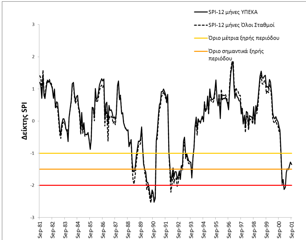
Σχήμα 21. Σύγκριση Δεικτών SPI 12 μηνών που προέκυψαν από διαφορετικό αριθμό βροχομετρικών σταθμών
