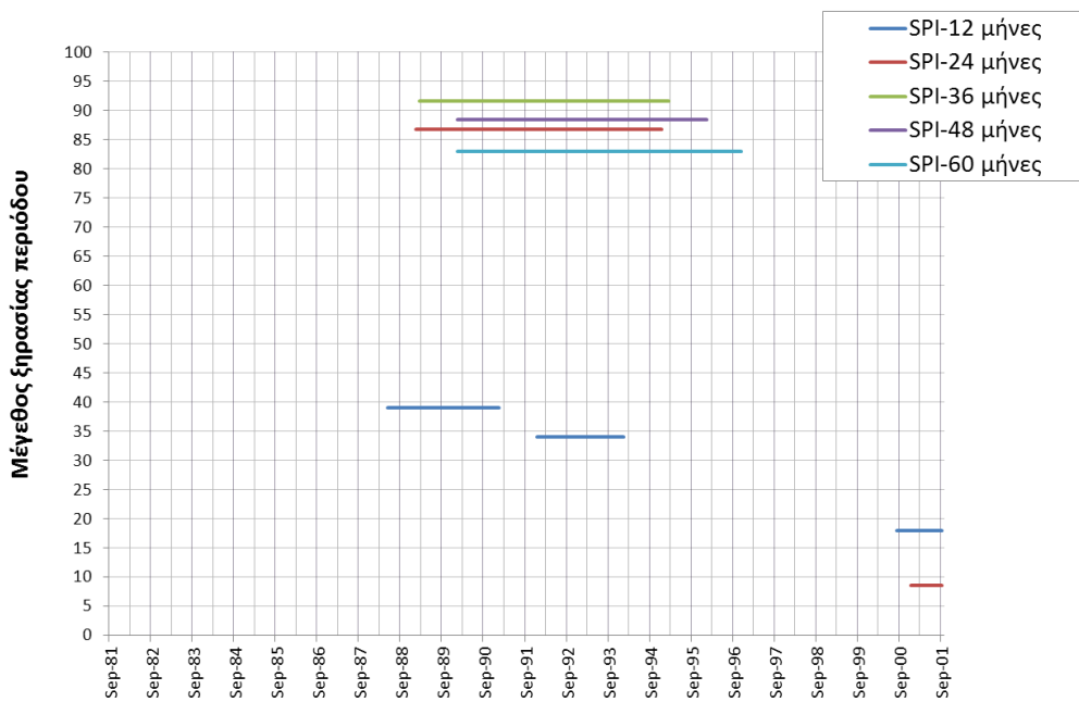
Σχήμα 22. Μέγεθος Ξηρασίας για διαφορετικές κλίμακες του Δείκτη SPI για τη Δ. Στερεά Ελλάδα
