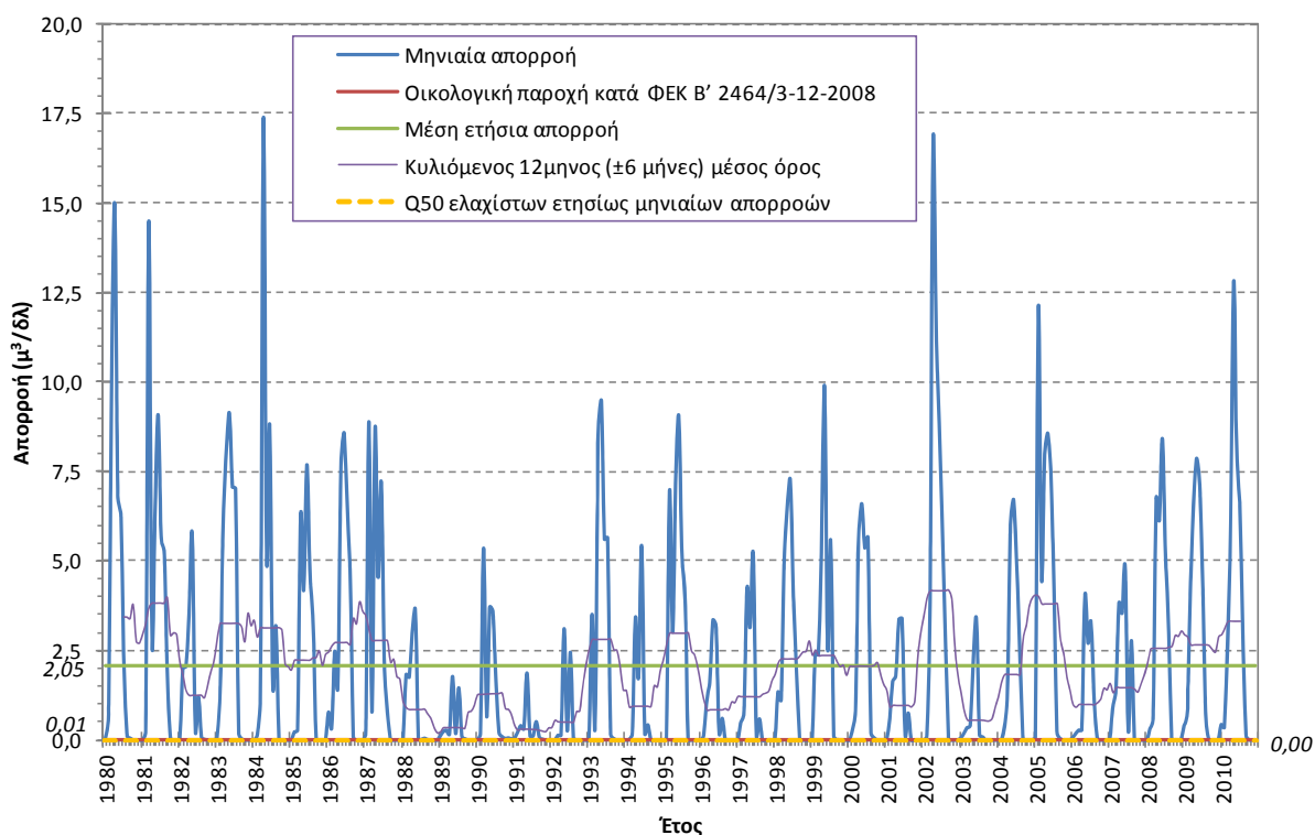
Σχήμα 8-4. Γράφημα απορροών στην εκβολή του π. Πλατύ (GR33)
