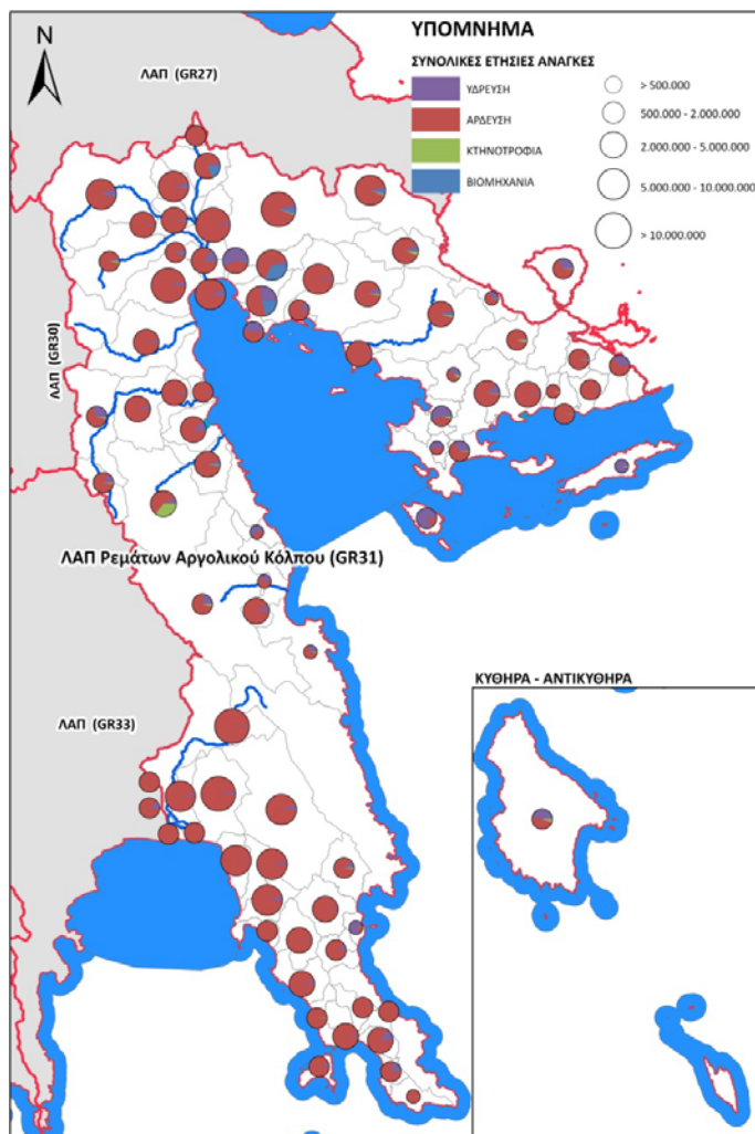
Σχήμα 7-13. Ετήσιες ανάγκες νερού ανά λεκάνη ΥΣ για τη ΛΑΠ Ρεμάτων Αργολικού Κόλπου (GR31)
