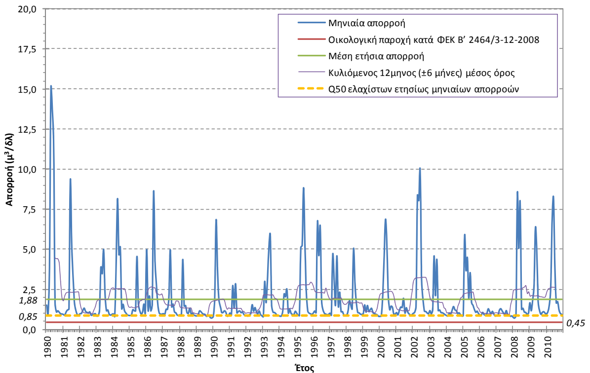
Σχήμα 8-2. Γράφημα απορροών στην εκβολή του π. Τάνου (GR31)
