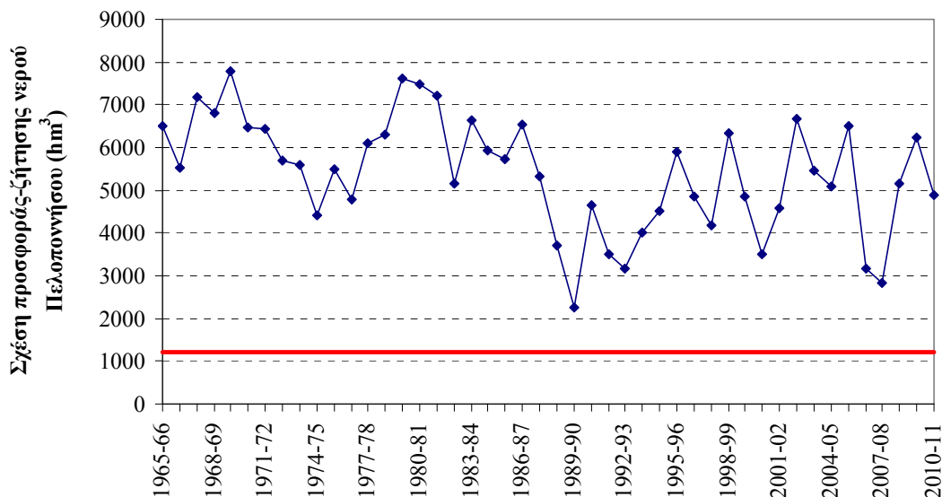
Σχήμα 7-26. Ετήσια χρονοσειρά διαθεσιμότητας υδατικών πόρων και ζήτησης νερού (συνεχής γραμμή), στο σύνολο της Πελοποννήσου.
