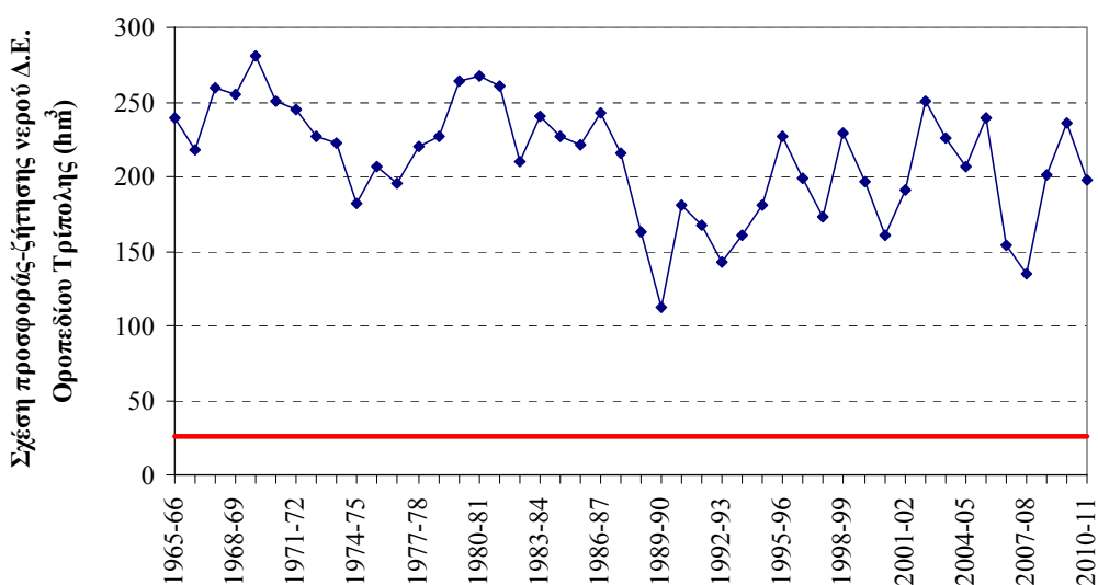
Σχήμα 7-20. Ετήσια χρονοσειρά διαθεσιμότητας υδατικών πόρων και ζήτησης νερού (συνεχής γραμμή), στην ΛΑΠ Οροπεδίου Τρίπολης.
