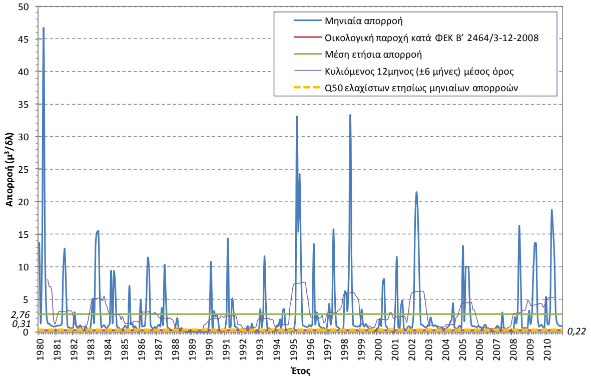
Σχήμα 8-1. Γράφημα απορροών στην εκβολή του π. Ίναχου (GR31)
