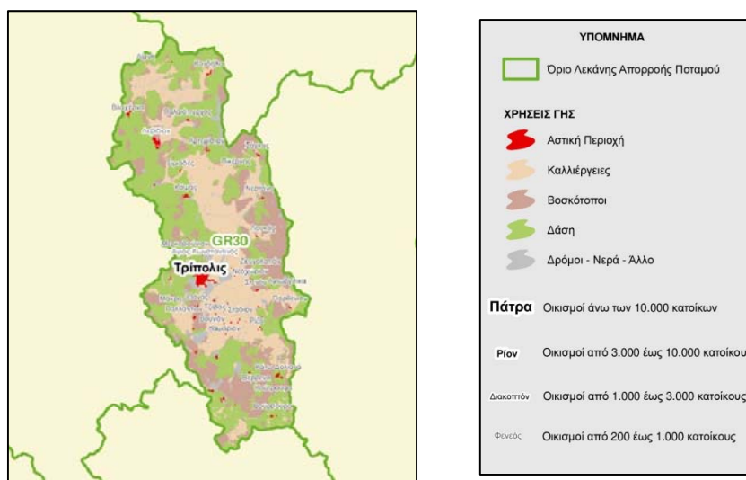
Σχήμα 7-1. Χάρτης χρήσεων γης στη Λεκάνη Απορροής Οροπεδίου Τρίπολης (GR30)
