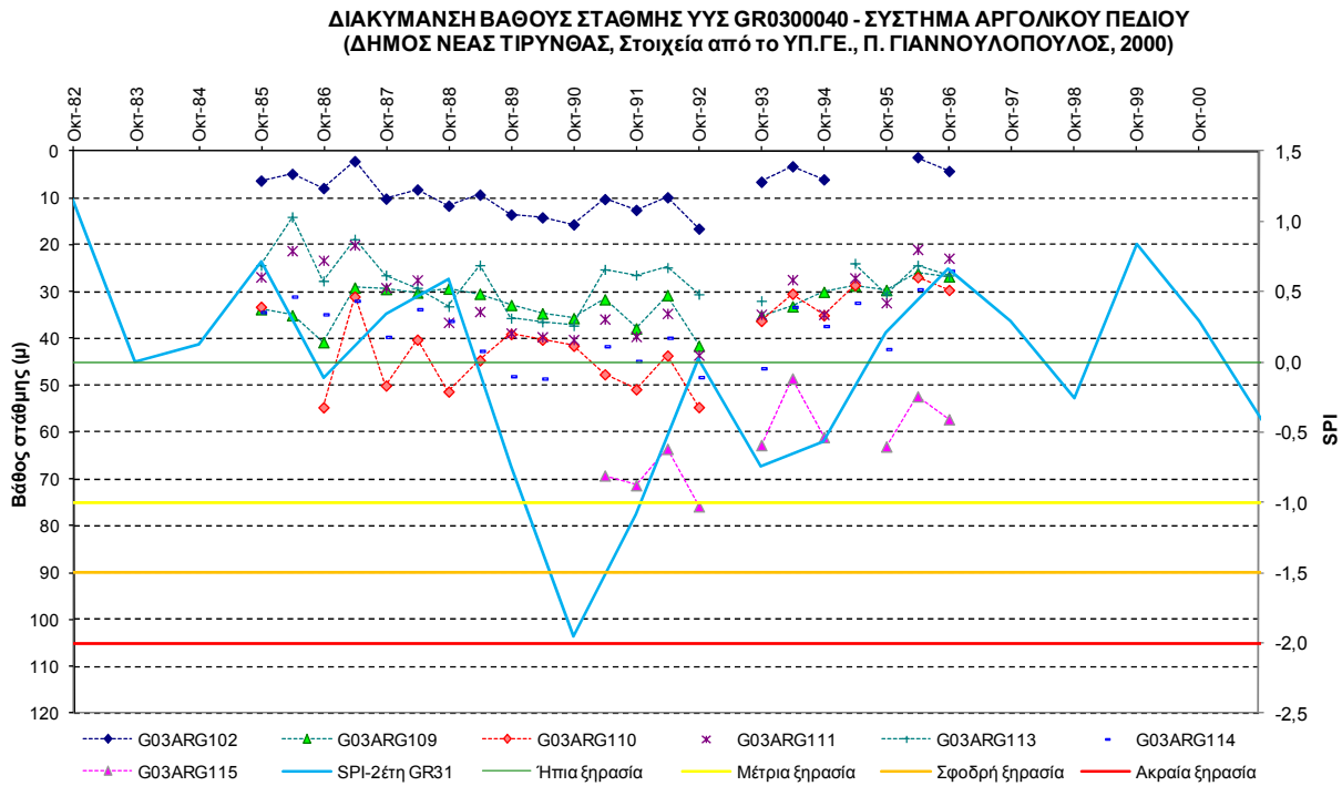
Σχήμα 5-30. Συσχέτιση SPI και όρια κατάταξής του με τη χρονοσειρά στάθμης νερού γεώτρησης στον Δήμο Νέας Τίρυνθας του ΥΥΣ GR0300040
