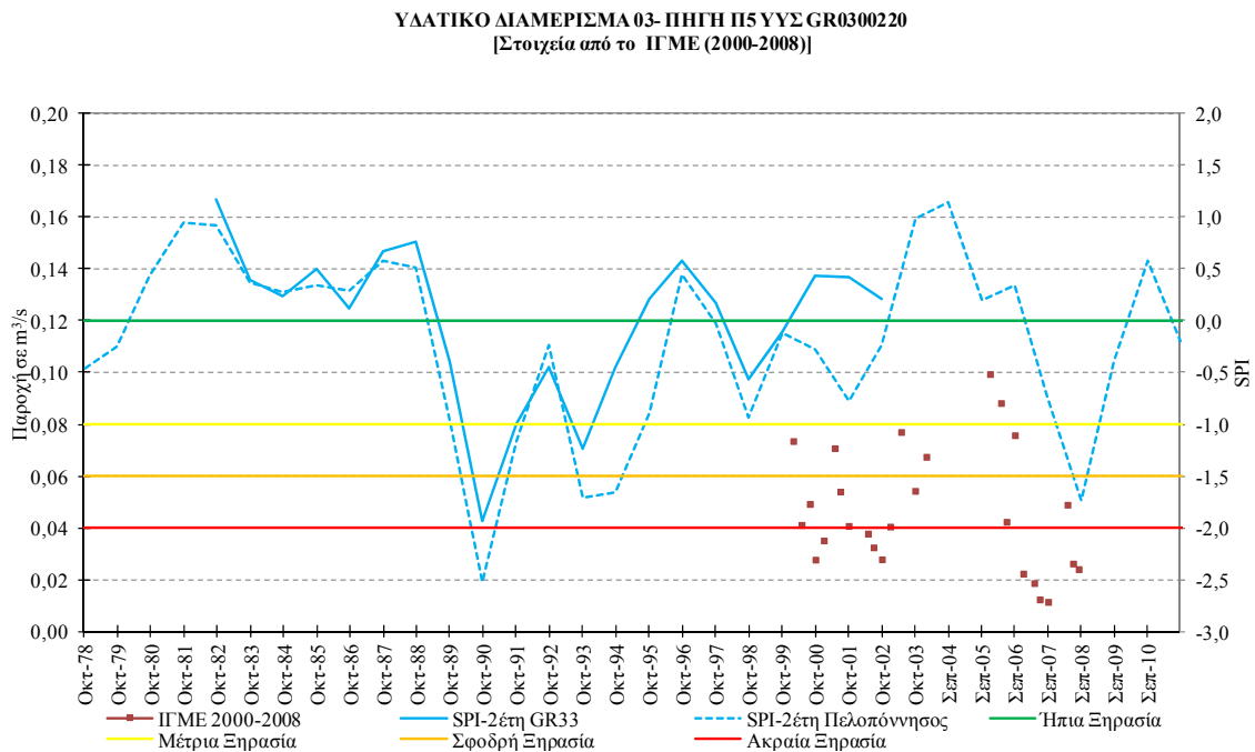
Σχήμα V-13. Συσχέτιση SPI και όρια κατάταξής του με τη χρονοσειρά παροχής της πηγής στη θέση Π5 του ΥΥΣ GR0300220
