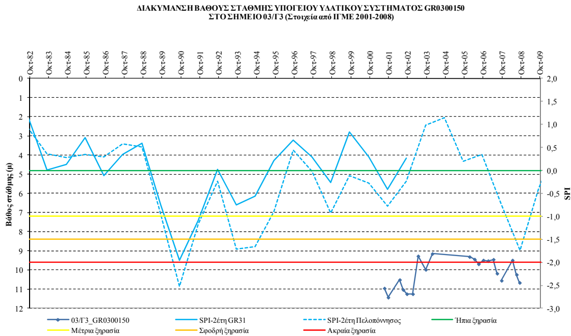
Σχήμα VI -15. Συσχέτιση SPI και όρια κατάταξής του με τη χρονοσειρά στάθμης νερού γεώτρησης στο σημείο 03/Γ3 του ΥΥΣ GR0300150
