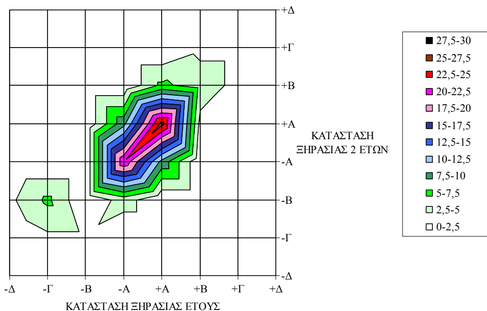
Σχήμα 9-25. Πιθανότητες μετάβασης (%) από κατηγορία ξηρασίας έτους σε κατηγορία ξηρασίας 2 ετών.
