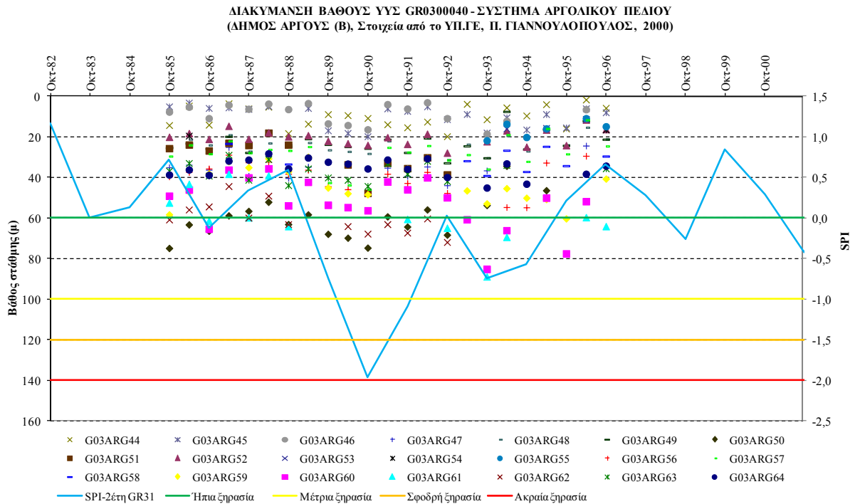
Σχήμα VI -19. Συσχέτιση SPI και όρια κατάταξής του με τη χρονοσειρά στάθμης νερού γεώτρησης στον Δήμο Άργους (Β) του ΥΥΣ GR0300040
