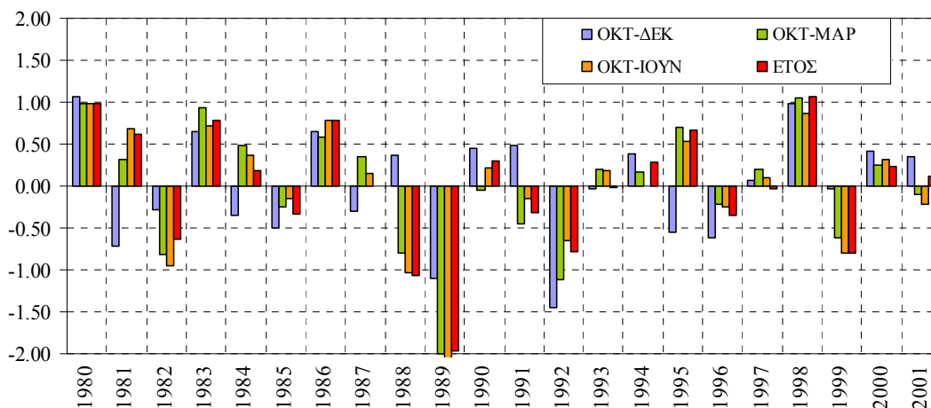
Σχήμα 5-10. Εκτίμηση δείκτη ξηρασίας διαχειριστικής ενότητας Ρεμάτων Αργολικού Κόλπου, για χρονικές κλίμακες από τρίμηνη έως ετήσια.
