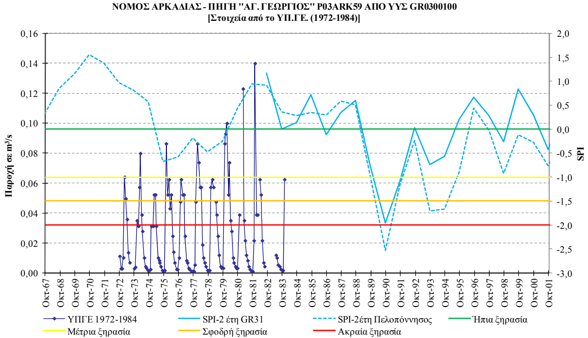
Σχήμα V -10. Συσχέτιση SPI και όρια κατάταξής του με τη χρονοσειρά παροχής της πηγής Αγίου Γεωργίου
