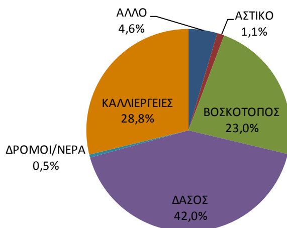
Σχήμα 7-2. Κατανομή των χρήσεων γης στη Λεκάνη Απορροής Οροπεδίου Τρίπολης (GR30)
