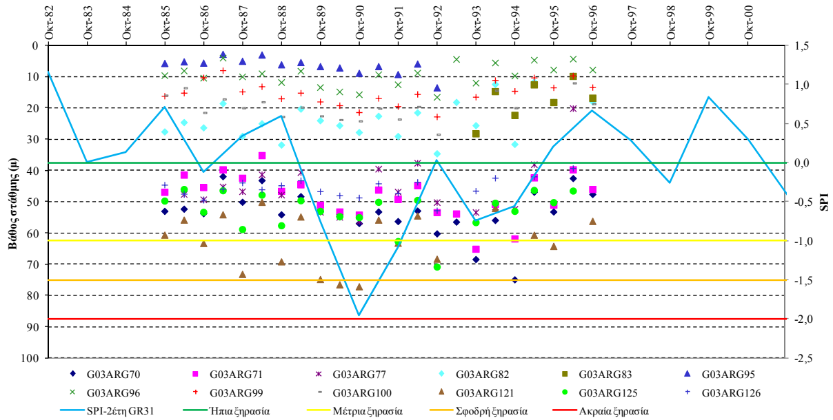
Σχήμα VI -22. Συσχέτιση SPI και όρια κατάταξής του με τη χρονοσειρά στάθμης νερού γεώτρησης στον Δήμο Μιδέας του ΥΥΣ GR0300040
