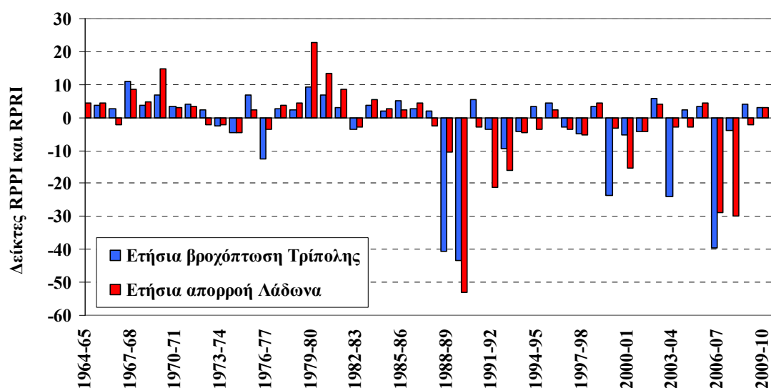
Σχήμα 5-21. Σύγκριση χρονικής εξέλιξης δείκτη RPRI ετήσιας απορροής Λάδωνα και δείκτη RPRI ετήσιας βροχόπτωσης Τρίπολης.
