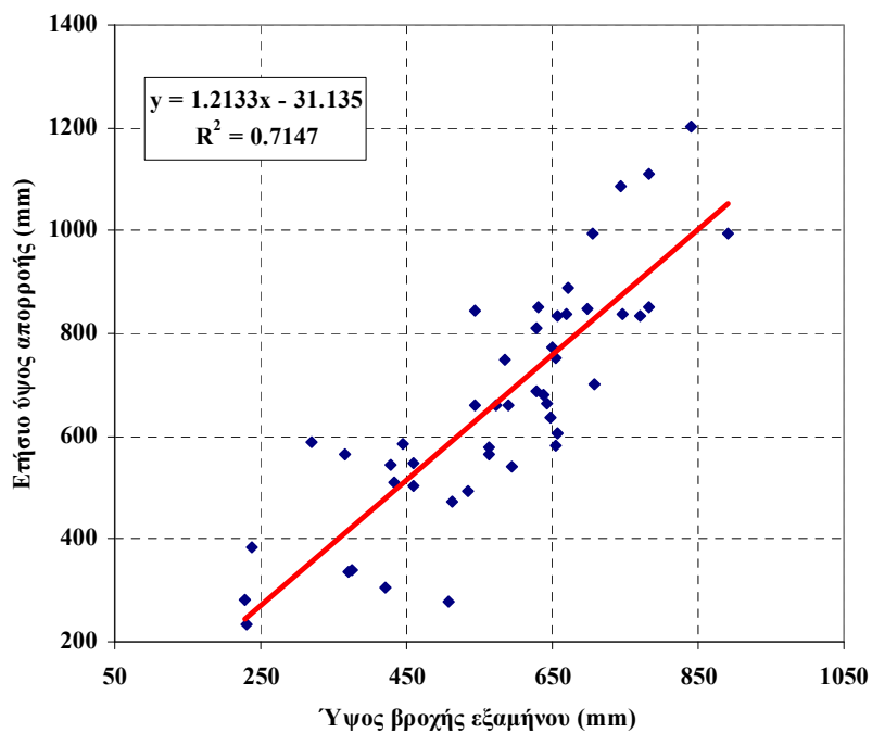
Σχήμα 9-19. Διάγραμμα διασποράς εξαμηνιαίου ύψους βροχής Τρίπολης και ετήσιου ύψους απορροής Λάδωνα.
