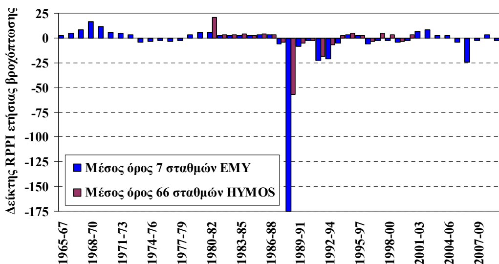
Σχήμα 5-15. Χρονική εξέλιξη δείκτη RPPI μέσης βροχόπτωσης δύο ετών σταθμών ΕΜΥ και σταθμών βάσης δεδομένων ΗΥΜΟΣ της μελέτης ανάπτυξης εργαλείων του ΥΠΑΝ.
