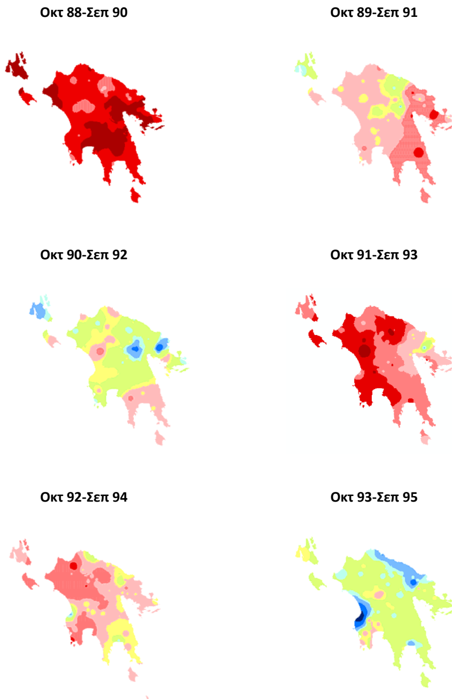
Σχήμα IV -1. Χωρική κατανομή ετήσιου δείκτη ξηρασίας ανά υδρολογικό έτος για την περίοδο 1980-2002.
