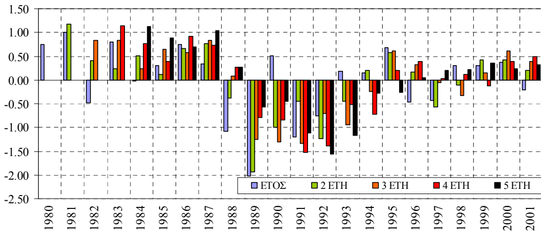
Σχήμα 5-13. Εκτίμηση δείκτη ξηρασίας διαχειριστικής ενότητας Ευρώτα, για χρονικές κλίμακες από ετήσια έως πενταετή.
