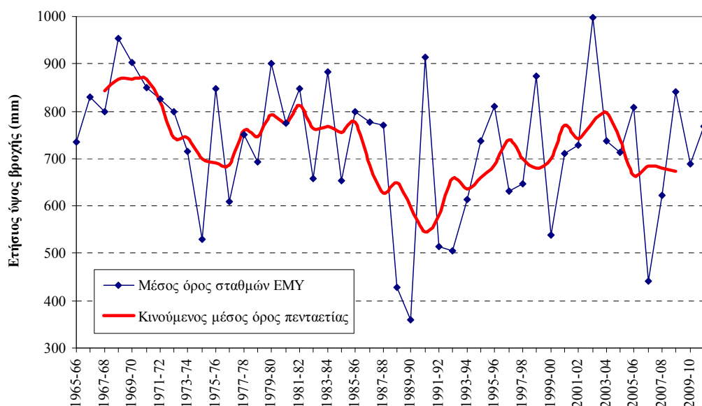
Σχήμα 4-2. Μέσο ετήσιο ύψος βροχής σταθμών EMY και κινούμενοι μέσοι όροι πέντε ετών.
