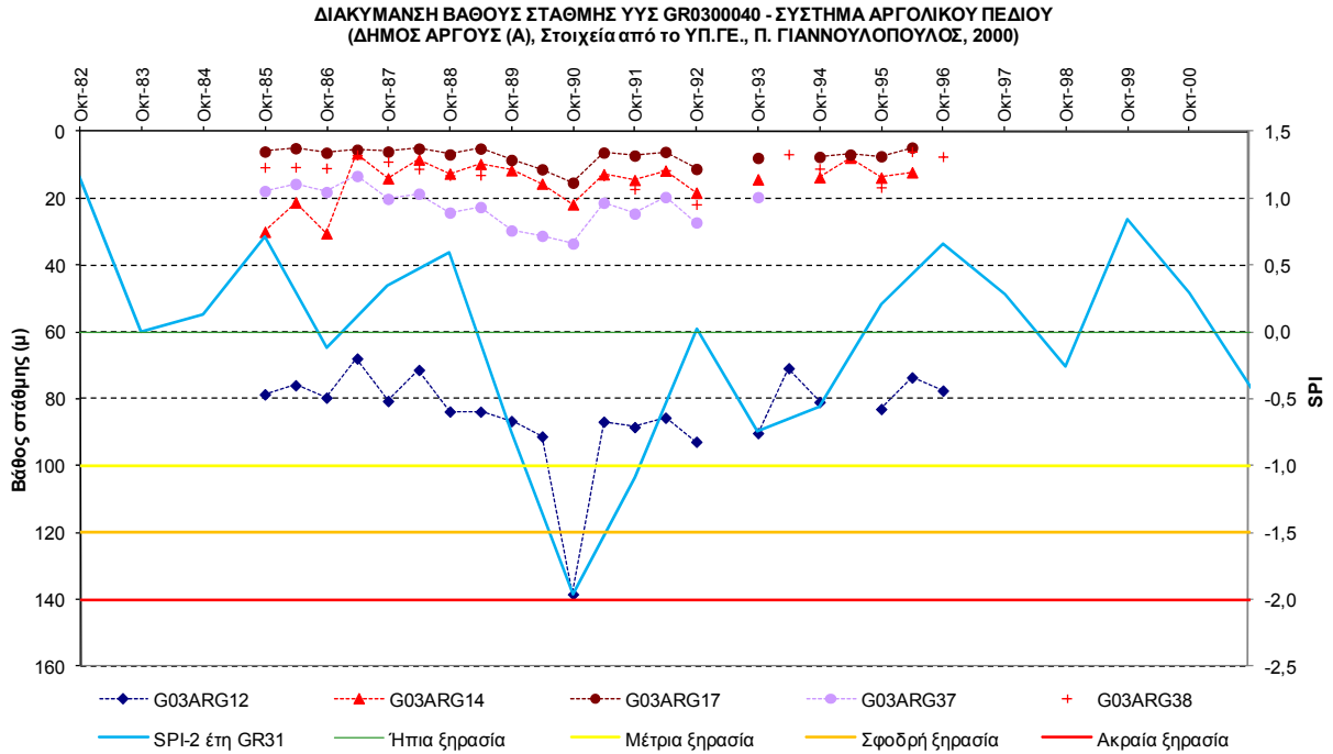
Σχήμα VI -18. Συσχέτιση SPI και όρια κατάταξής του με τη χρονοσειρά στάθμης νερού γεώτρησης στον Δήμο Άργους (Α) του ΥΥΣ GR0300040
