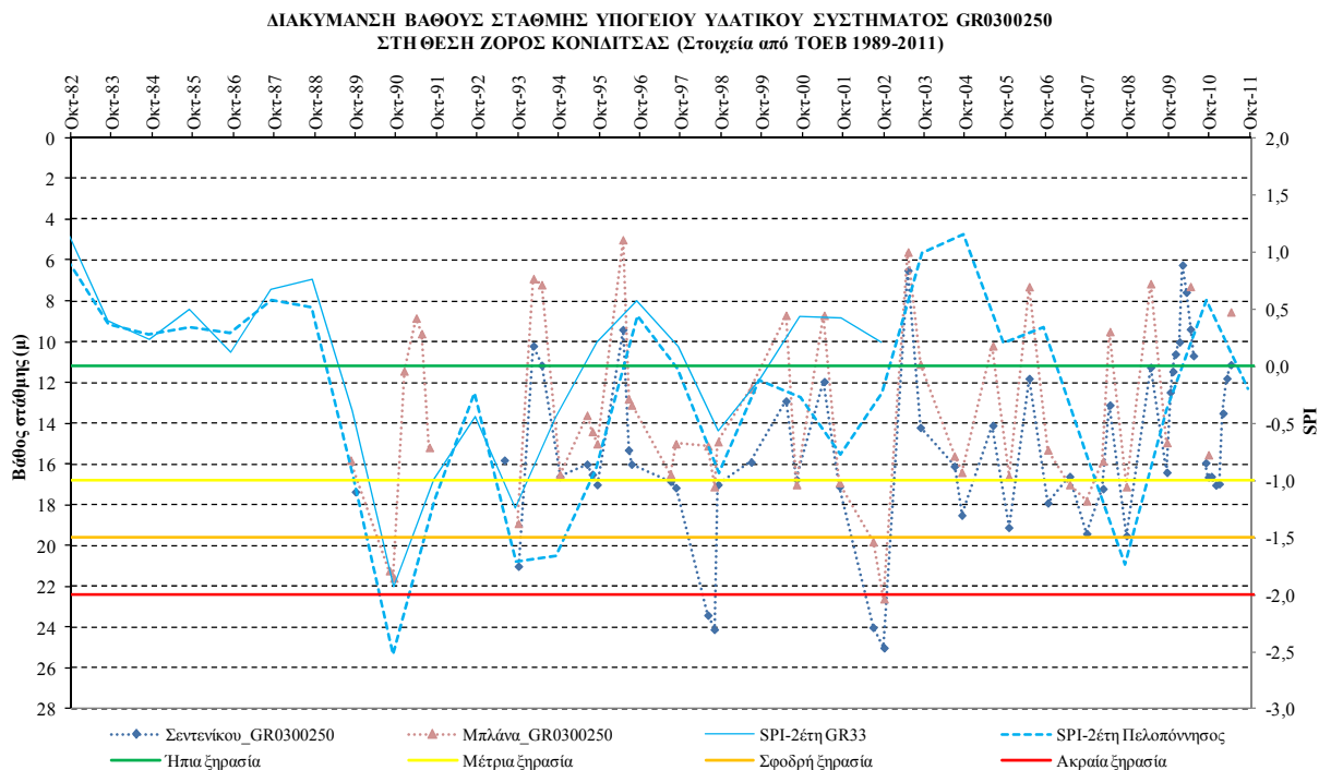
Σχήμα 5-34. Συσχέτιση SPI και όρια κατάταξης του με τη χρονοσειρά στάθμης νερού γεώτρησης στη θέση Ζόρος Κονιδίτσας του ΥΓΣ GR0300250
