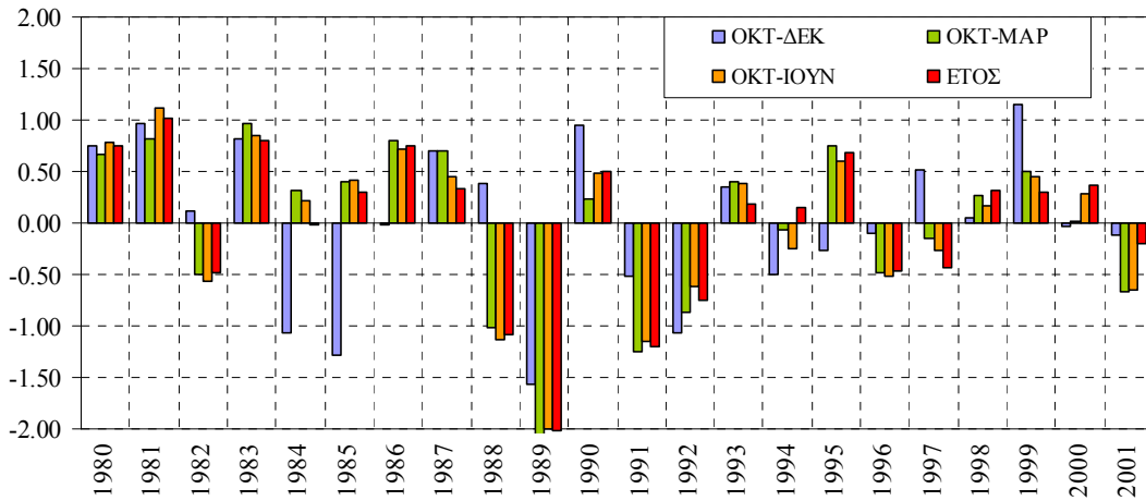
Σχήμα 5-12. Εκτίμηση δείκτη ξηρασίας διαχειριστικής ενότητας Ευρώτα, για χρονικές κλίμακες από τρίμηνη έως ετήσια.
