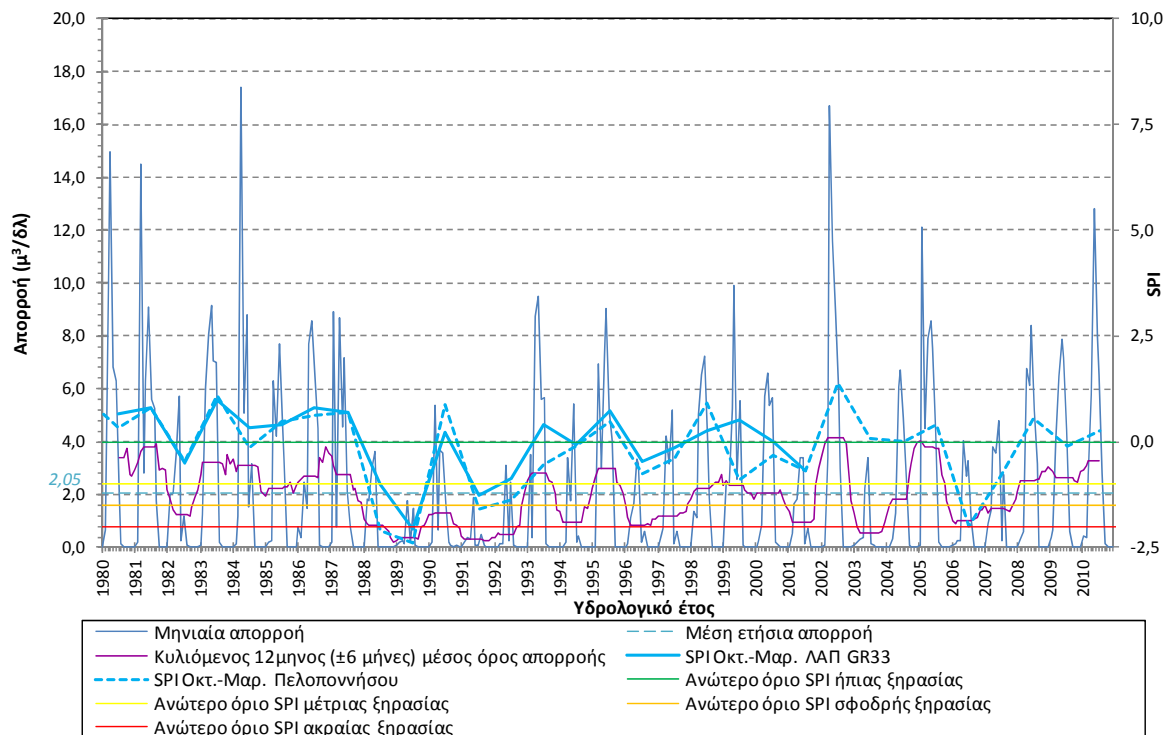
Σχήμα 5-24. Συσχέτιση SPI και όρια κατάταξης του με τη χρονοσειρά απορροής του μοντέλου Sacramento για την περιοχή της εκβολής του π.Πλατού (Σημείο 3_681_0)
