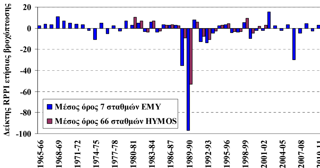
Σχήμα 5-14. Χρονική εξέλιξη δείκτη RPPI μέσης ετήσιας βροχόπτωσης σταθμών ΕΜΥ και των δεδομένων του προγράμματος ΗΥΜΟΣ της μελέτης ανάπτυξης εργαλείων του ΥΠΑΝ.
