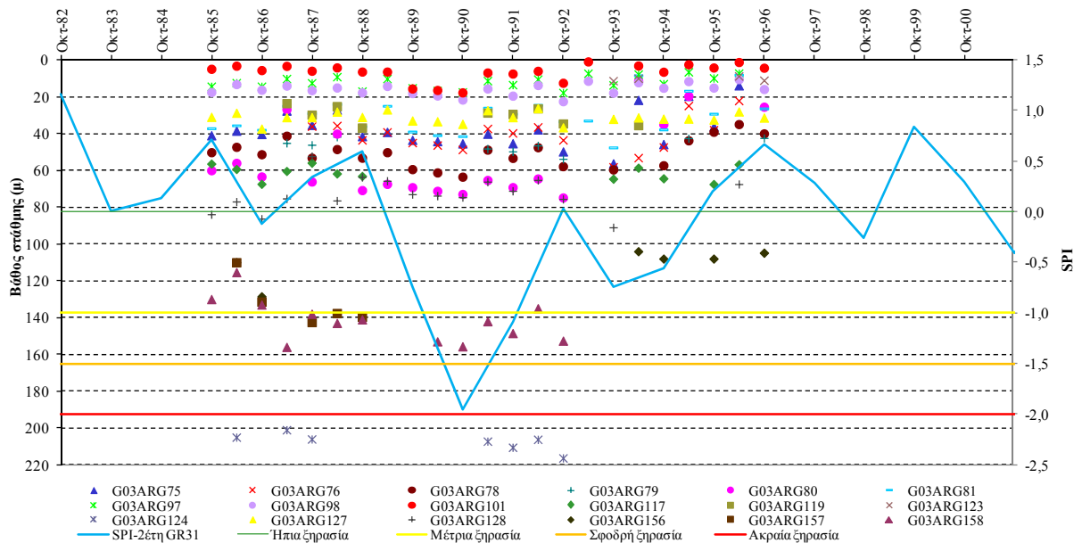
Σχήμα VI -21. Συσχέτιση SPI και όρια κατάταξής του με τη χρονοσειρά στάθμης νερού γεώτρησης στον Δήμο Μιδέας του ΥΥΣ GR0300040
