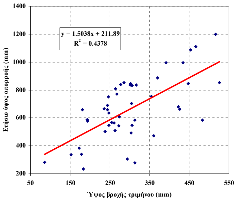
Σχήμα 9-18. Διάγραμμα διασποράς τριμηνιαίου ύψους βροχής Τρίπολης και ετήσιου ύψους απορροής Λάδωνα.
