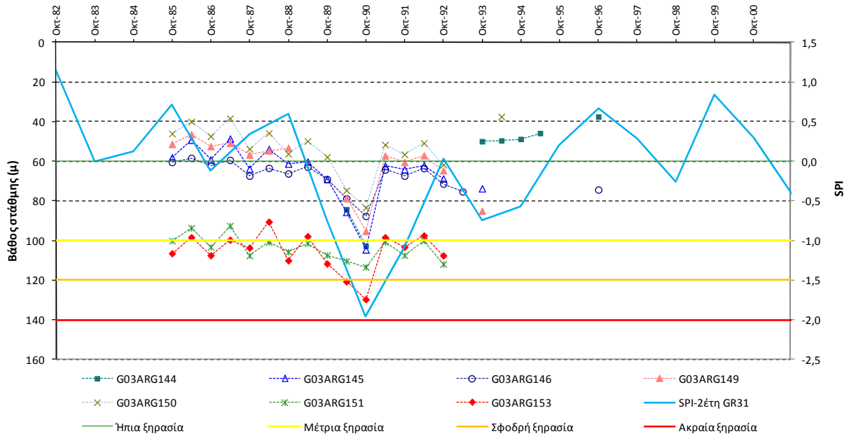
Σχήμα VI -24. Συσχέτιση SPI και όρια κατάταξης του με τη χρονοσειρά στάθμης νερού γεώτρησης στον Δήμο Μυκηναιών του ΥΥΣ GR0300040
