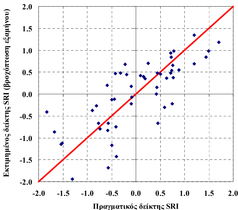
Σχήμα 10-7. Διάγραμμα διασποράς εκτιμημένου, με βάση την αθροιστική βροχόπτωση εξαμήνου (του σταθμού Τρίτολης), και πραγματικού δείκτη SRI μέσης ετήσιας απορροής στη λεκάνη η του Λάδωνα.
