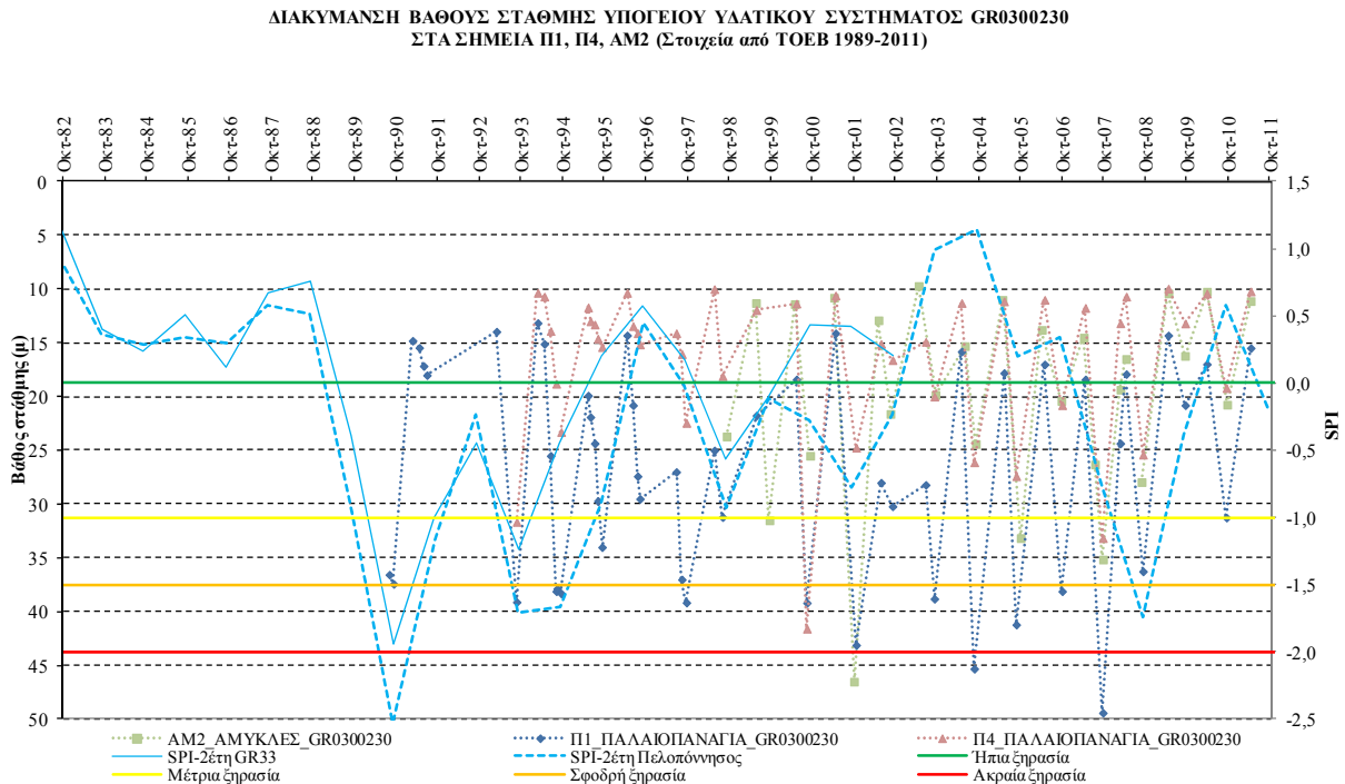
Σχήμα VI -29. Συσχέτιση SPI και όρια κατάταξής του με τη χρονοσειρά στάθμης νερού γεώτρησης στα σημεία Π1, Π4, AM2 του ΥΥΣ GR0300230
