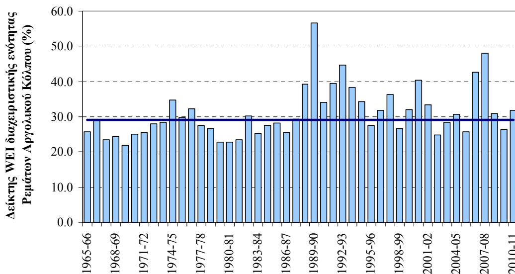
Σχήμα 7-23. Ετήσια μεταβολή του δείκτη WEI, στην ΛΑΠ 31 (με συνεχή γραμμή απεικονίζεται ο υπερετήσιος δείκτης που υπολογίστηκε με βάση τα μεγέθη του μέσου ετήσιου υδατικού ισοζυγίου της ΛΑΠ).
