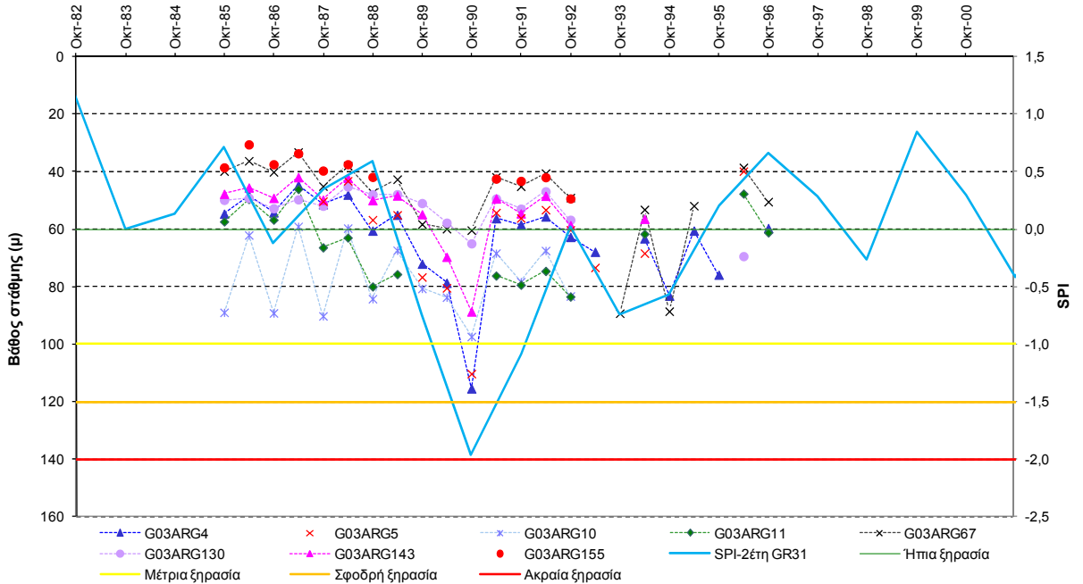
Σχήμα VI -25. Συσχέτιση SPI και όρια κατάταξης του με τη χρονοσειρά στάθμης νερού γεώτρησης στον Δήμο Κουτσοποδίου (Α) του ΥΥΣ GR0300040
