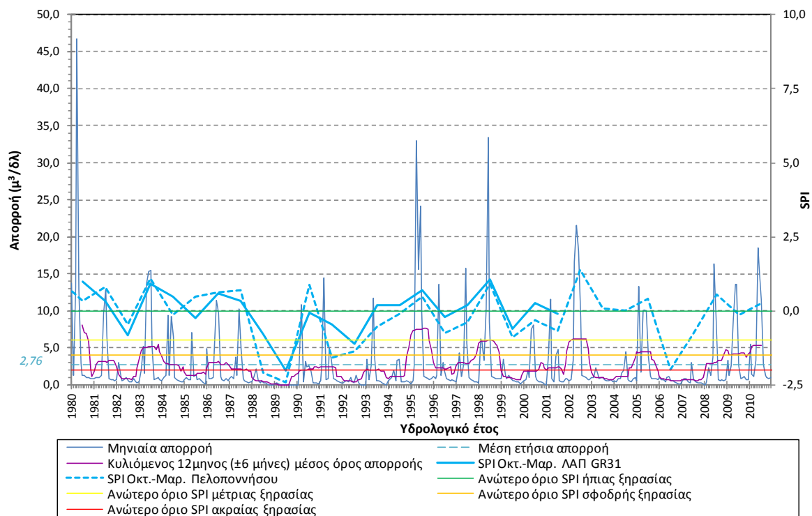
Σχήμα 5-25. Συσχέτιση SPI και όρια κατάταξης του με τη χρονοσειρά απορροής του μοντέλου Sacramento για την περιοχή της εκβολής του π.Ίναχου (Σημείο 3_601_0)
