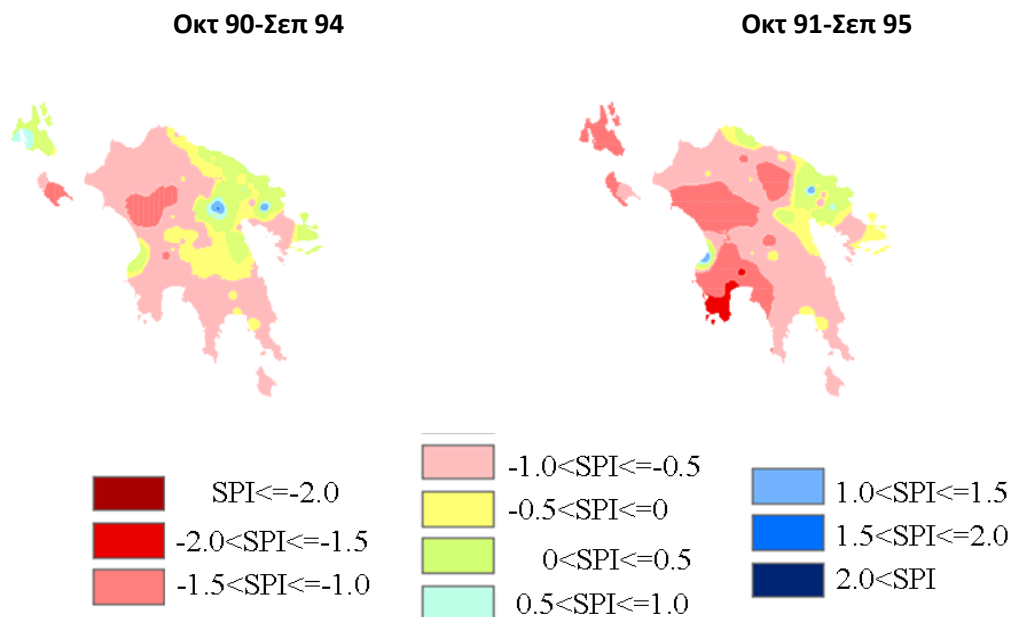
Σχήμα IV -4. Χωρική κατανομή δείκτη ξηρασίας μέσου δείκτη ξηρασίας τεσσάρων ετών για την περίοδο 1988-1995.
