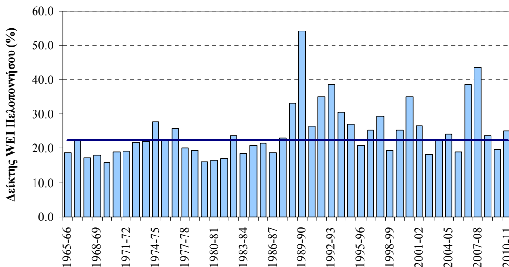
Σχήμα 7-27. Ετήσια μεταβολή του δείκτη WEI στο σύνολο της Πελοποννήσου (με συνεχή γραμμή απεικονίζεται ο υπερετήσιος δείκτης που υπολογίστηκε με βάση τα μεγέθη του μέσου ετήσιου υδατικού ισοζυγίου της περιοχής μελέτης).
