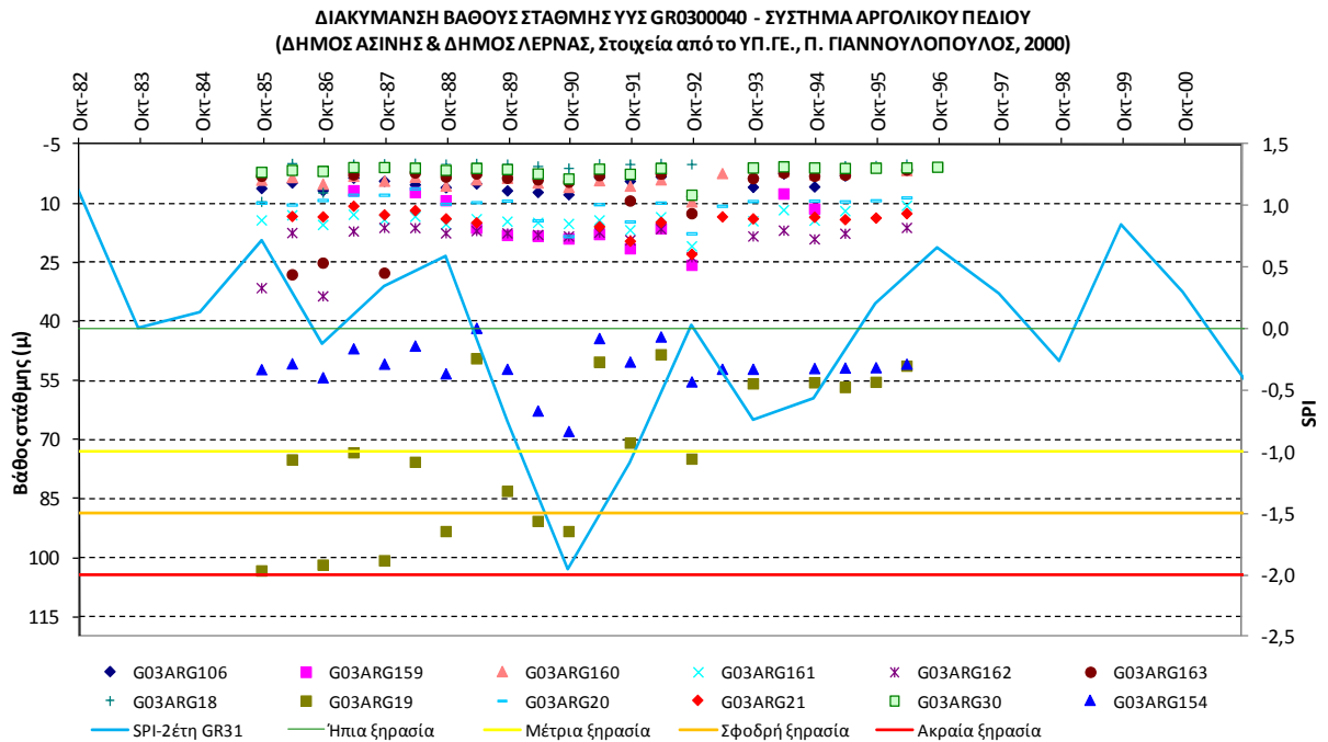
Σχήμα VI -17. Συσχέτιση SPI και όρια κατάταξής του με τη χρονοσειρά στάθμης νερού γεώτρησης στον Δήμο Ασίνης και Λέρνας του ΥΥΣ GR0300040
