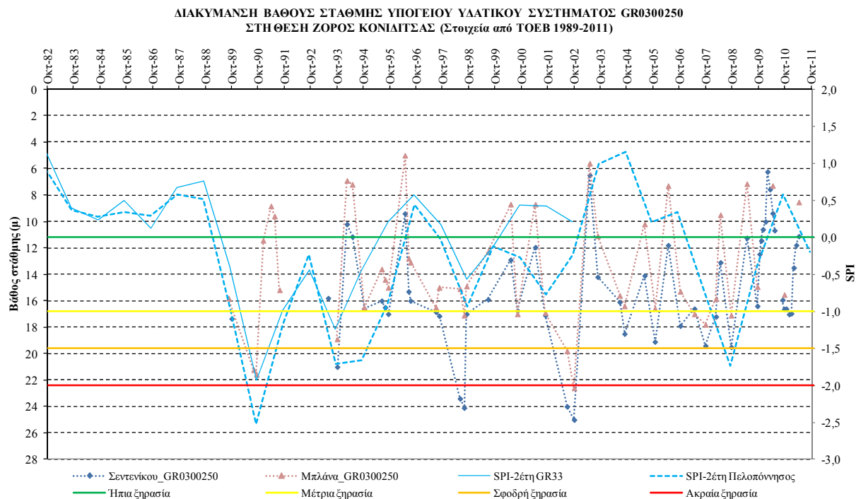
Σχήμα VI -30. Συσχέτιση SPI και όρια κατάταξης του με τη χρονοσειρά στάθμης νερού γεώτρησης στη θέση Ζόρος Κονιδίτσας του ΥΓΣ GR0300250
