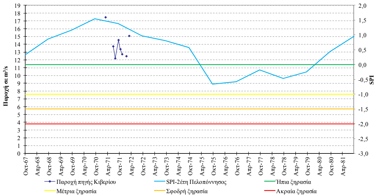
Σχήμα V -9. Συσχέτιση SPI και όρια κατάταξής του με τη χρονοσειρά παροχής της πηγής Κιβεριού (Ανάβαλος)
