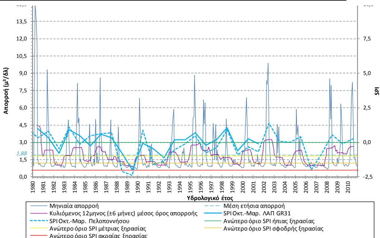
Σχήμα 5-26. Συσχέτιση SPI και όρια κατάταξής του με τη χρονοσειρά απορροής του μοντέλου Sacramento για την περιοχή της εκβολής του π. Τάνου (Σημείο 3_621_0)
