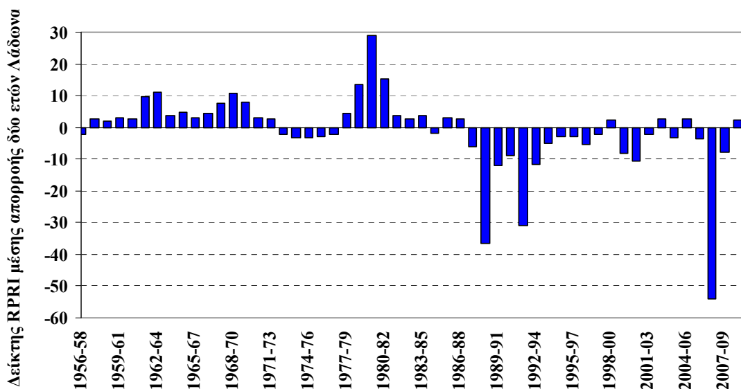
Σχήμα 5-18. Χρονική εξέλιξη δείκτη RPRI μέσης απορροής δύο ετών Λάδωνα.
