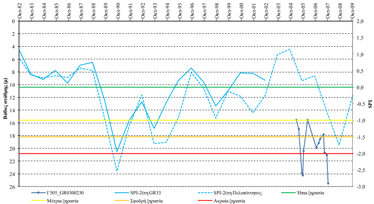
Σχήμα VI -27. Συσχέτιση SPI και όρια κατάταξής του με τη χρονοσειρά στάθμης νερού γεώτρησης στο σημείο Γ505 του ΥΥΣ GR0300230
