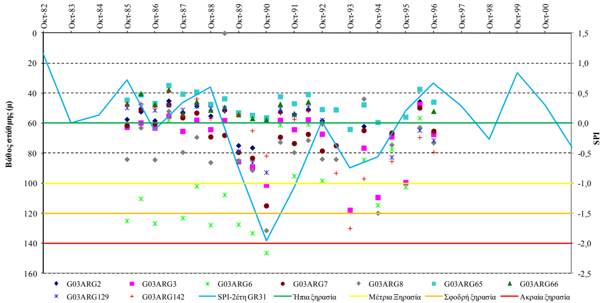
Σχήμα VI -26. Συσχέτιση SPI και όρια κατάταξής του με τη χρονοσειρά στάθμης νερού γεώτρησης στον Δήμο Κουτσοποδίου (B) του ΥΥΣ GR0300040
