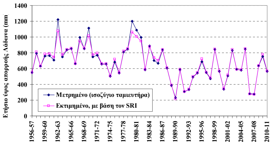
Σχήμα 7-16. Σύγκριση ετήσιων χρονοσειρών απορροής Λάδωνα, μετρημένων (υπολογισμός από το υδατικό ισοζύγιο του ταμιευτήρα) και εκτιμημένων, με βάση τη σχέση (7.7).
