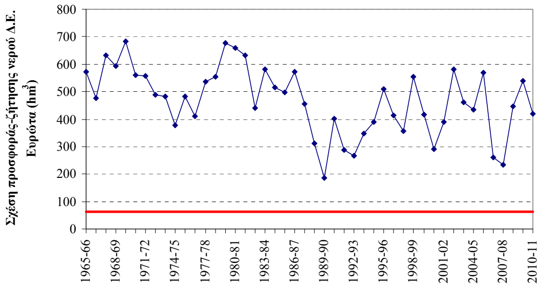
Σχήμα 7-24. Ετήσια χρονοσειρά διαθεσιμότητας υδατικών πόρων και ζήτησης νερού (συνεχής γραμμή), στην ΛΑΠ Ευρώτα.
