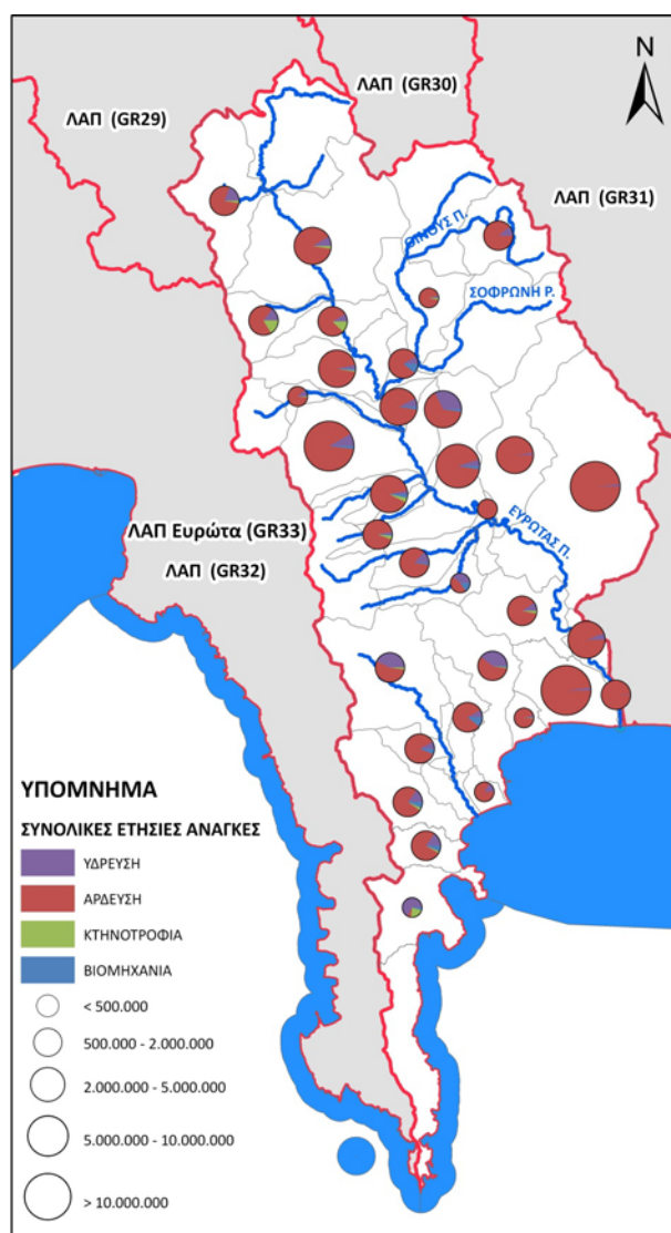
Σχήμα 7-15. Ετήσιες ανάγκες νερού ανά λεκάνη ΥΣ για τη ΛΑΠ Ευρώτα (GR33)
