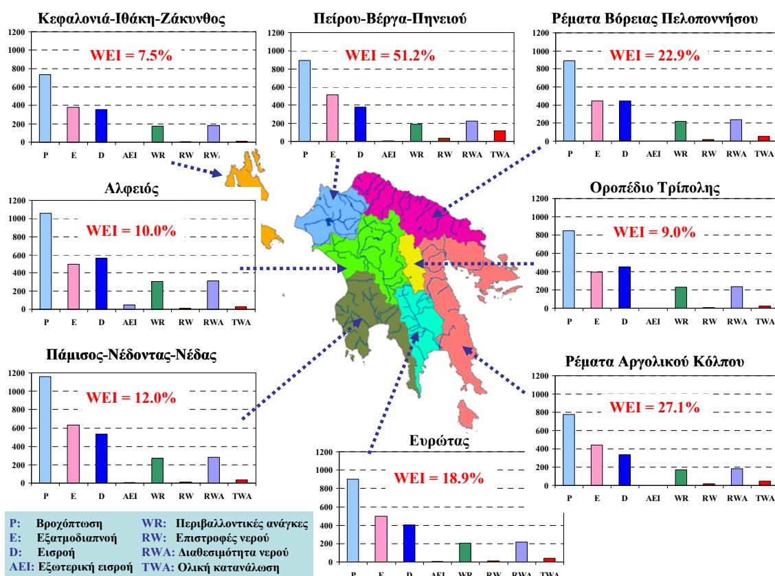
Σχήμα 7-19. Τιμές δείκτη WEI ανά διαχειριστική ενότητα και συνιστώσες μέσου ετήσιου υδατικού ισοζυγίου (τιμές σε mm).
