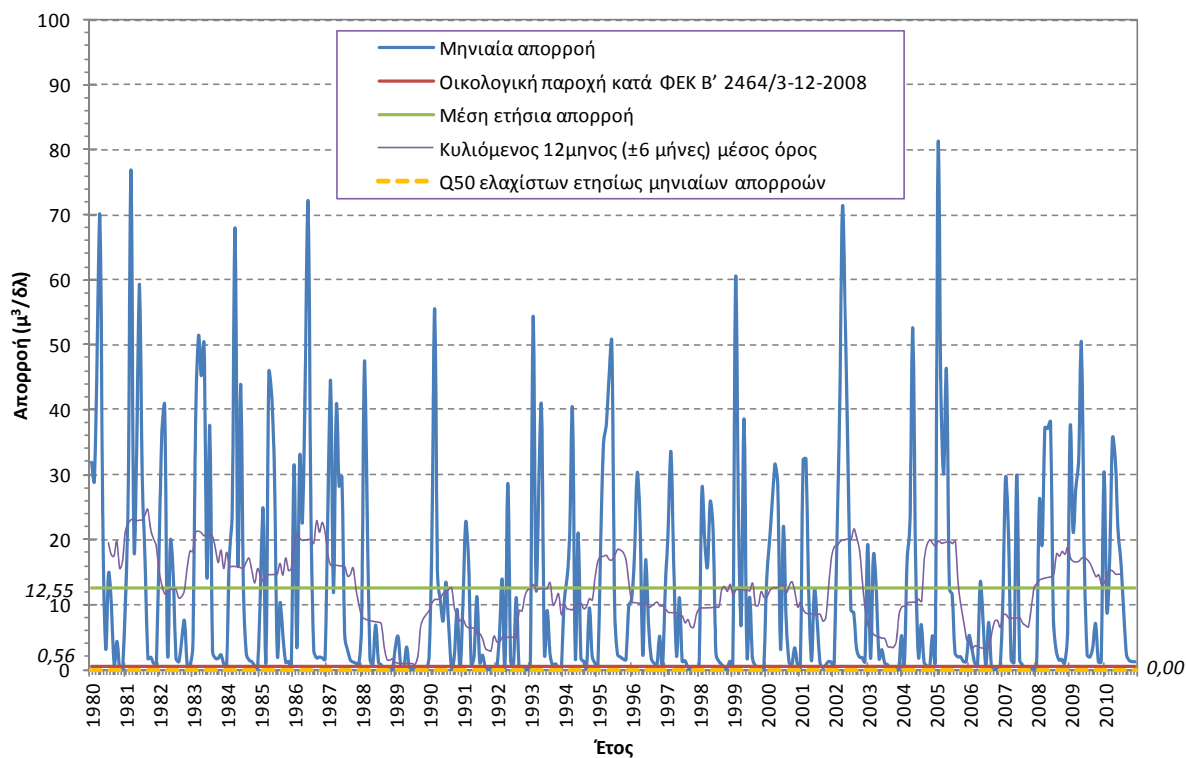
Σχήμα 8-3. Γράφημα απορροών στην εκβολή του π. Ευρώτα (GR33)
