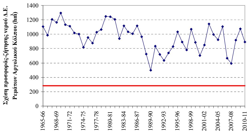
Σχήμα 7-22. Ετήσια χρονοσειρά διαθεσιμότητας υδατικών πόρων και ζήτησης νερού (συνεχής γραμμή), στην ΛΑΠ Ρεμάτων Αργολικού Κόλπου.
