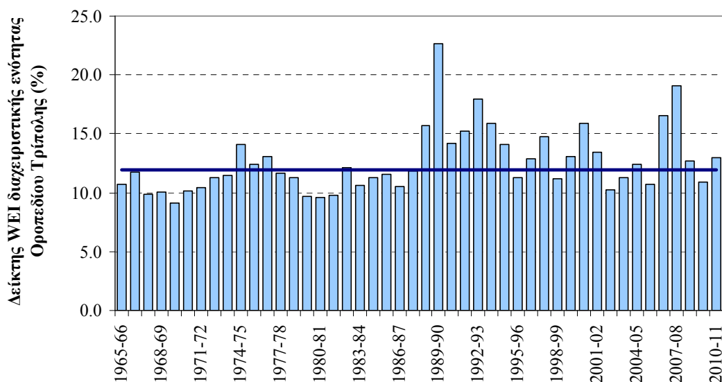
Σχήμα 7-21. Ετήσια μεταβολή του δείκτη WEI, στην ΛΑΠ 30(με συνεχή γραμμή απεικονίζεται ο υπερετήσιος δείκτης που υπολογίστηκε με βάση τα μεγέθη του μέσου ετήσιου υδατικού ισοζυγίου της ΛΑΠ).
