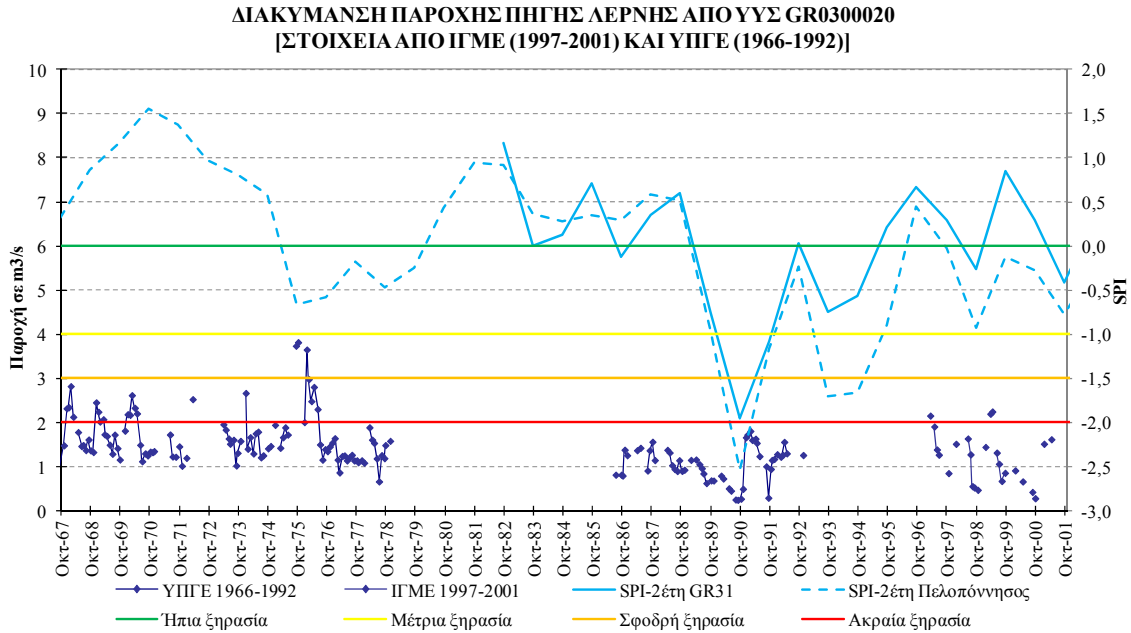
Σχήμα V-6. Συσχέτιση SPI και όρια κατάταξης του με τη χρονοσειρά παροχής της πηγής Λέρνης
