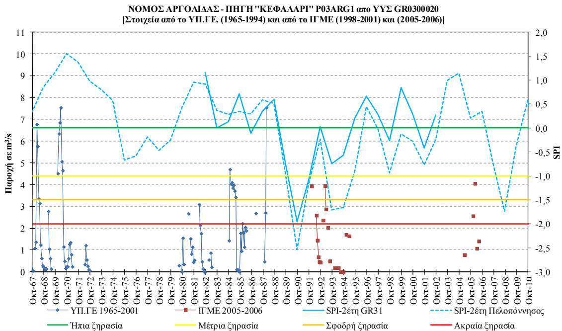
Σχήμα V-7. Συσχέτιση SPI και όρια κατάταξης του με τη χρονοσειρά παροχής της πηγής Κεφαλάρι
