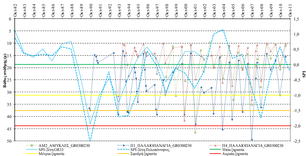
Σχήμα 5-33. Συσχέτιση SPI και όρια κατάταξής του με τη χρονοσειρά στάθμης νερού γεώτρησης στα σημεία Π1, Π4, ΑΜ2 του ΥΥΣ GR0300230
