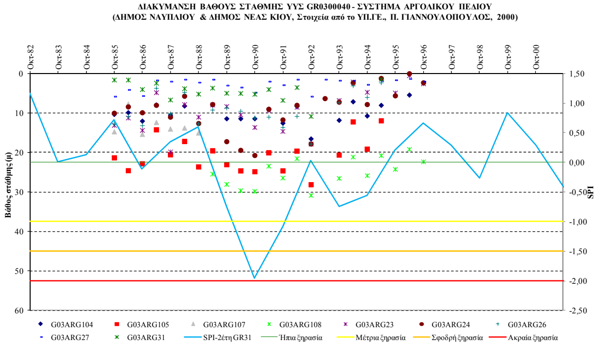
Σχήμα VI -16. Συσχέτιση SPI και όρια κατάταξής του με τη χρονοσειρά στάθμης νερού γεώτρησης στον Δήμο Ναυπλίου και Νέας Κίου του ΥΥΣ GR0300040
