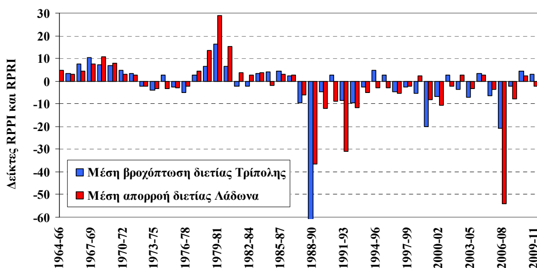
Σχήμα 5-22. Σύγκριση χρονικής εξέλιξης δείκτη RPRI απορροής διετίας Λάδωνα και δείκτη RPRI βροχόπτωσης διετίας Τρίπολης.
