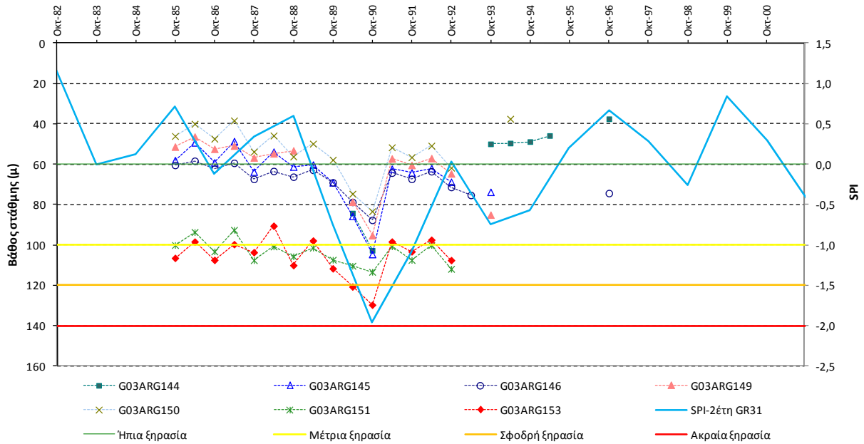
Σχήμα 5-31. Συσχέτιση SPI και όρια κατάταξης του με τη χρονοσειρά στάθμης νερού γεώτρησης στον Δήμο Μυκηναιών του ΥΥΣ GR0300040
