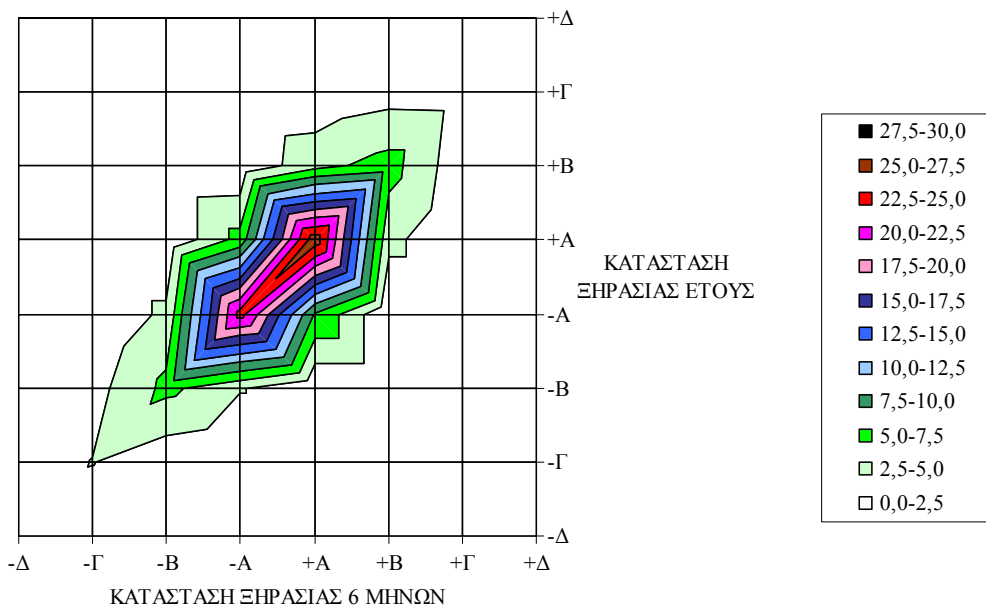
Σχήμα 9-4. Πιθανότητες μετάβασης (%) από κατηγορία ξηρασίας 6 μηνών σε κατηγορία ξηρασίας υδρολογικού έτους
