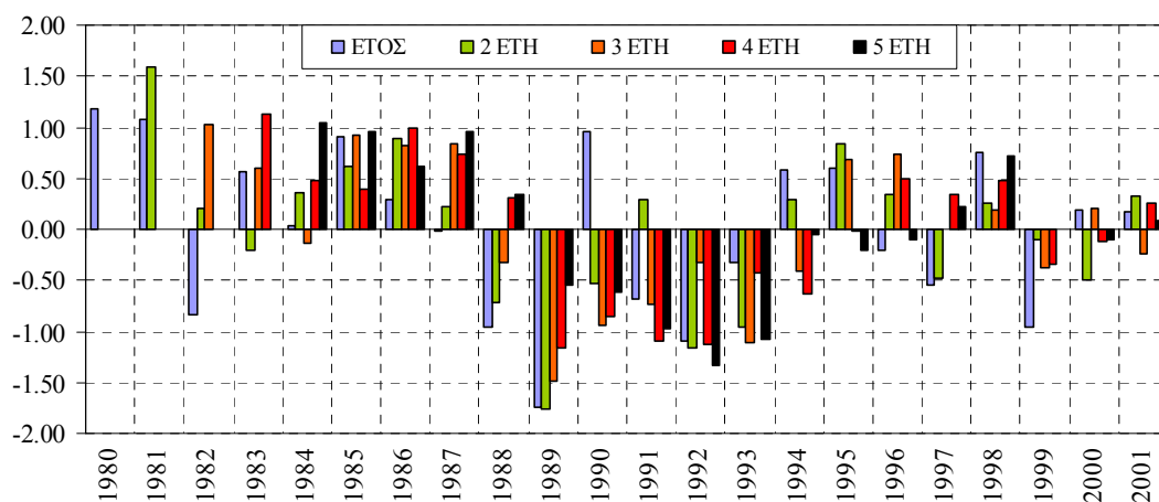
Σχήμα 5-9. Εκτίμηση δείκτη ξηρασίας διαχειριστικής ενότητας Οροπεδίου Τρίπολης, για χρονικές κλίμακες από ετήσια έως πενταετή.
