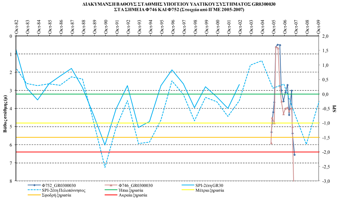
Σχήμα VI-14. Συσχέτιση SPI και όρια κατάταξής του με τη χρονοσειρά στάθμης νερού γεώτρησης στα σημεία Φ752 και Φ746 του ΥΥΣ GR0300030
