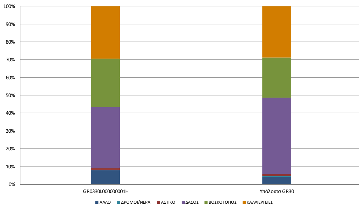
Σχήμα 7-3. Κατανομή των χρήσεων γης στις υπολεκάνες της ΛΑΠ Οροπεδίου Τρίπολης (GR30)
