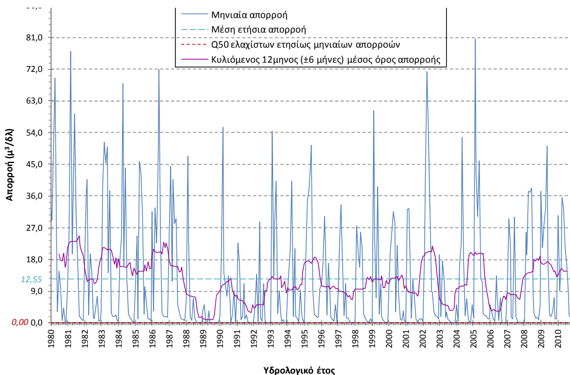
Σχήμα 4-8. Χρονοσειρά απορροής, μέση ετήσια απορροή, κυλιόμενος μέσος όρος και Q 50 ελαχίστων για την περιοχή της εκβολής του π.Ευρώτα (Σημείο 3_101_0)
