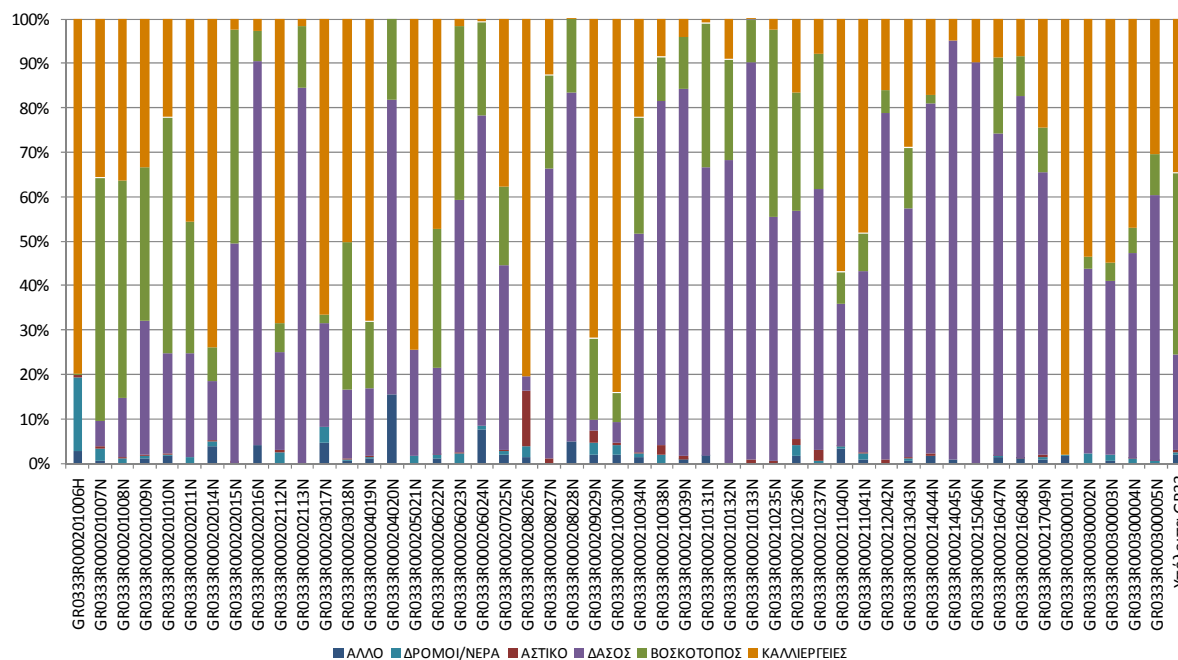
Σχήμα 7-9. Κατανομή των χρήσεων γης στις υπολεκάνες της ΛΑΠ Ευρώτα (GR33)
