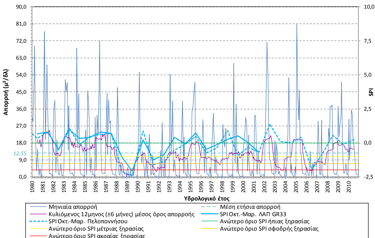
Σχήμα 5-23. Συσχέτιση SPI και όρια κατάταξης του με τη χρονοσειρά απορροής του μοντέλου Sacramento για την περιοχή της εκβολής του π.Ευρώτα (Σημείο 3_101_0)
