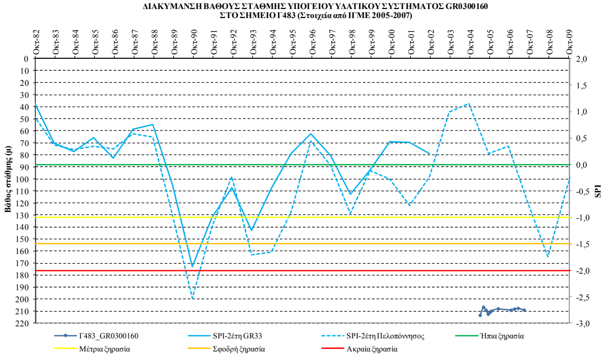
Σχήμα VI -28. Συσχέτιση SPI και όρια κατάταξής του με τη χρονοσειρά στάθμης νερού γεώτρησης στο σημείο Γ483 του ΥΥΣ GR0300160
