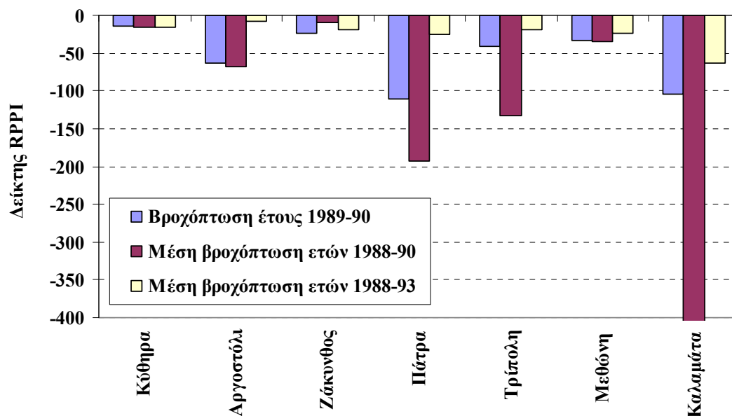
Σχήμα 5-16. Χρονική εξέλιξη δείκτη RPPI σημειακής βροχόπτωσης σταθμών ΕΜΥ για χαρακτηριστικές χρονικές περιόδους.
