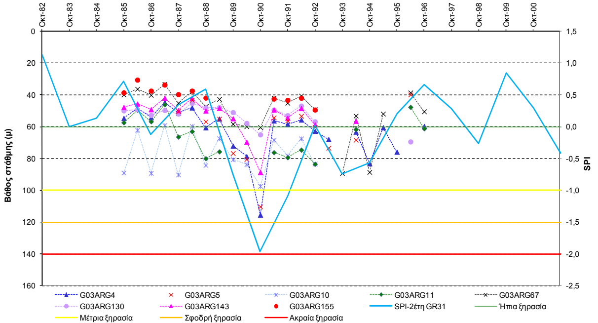
Σχήμα 5-32. Συσχέτιση SPI και όρια κατάταξης του με τη χρονοσειρά στάθμης νερού γεώτρησης στον Δήμο Κουτσοποδίου του ΥΥΣ GR0300040
