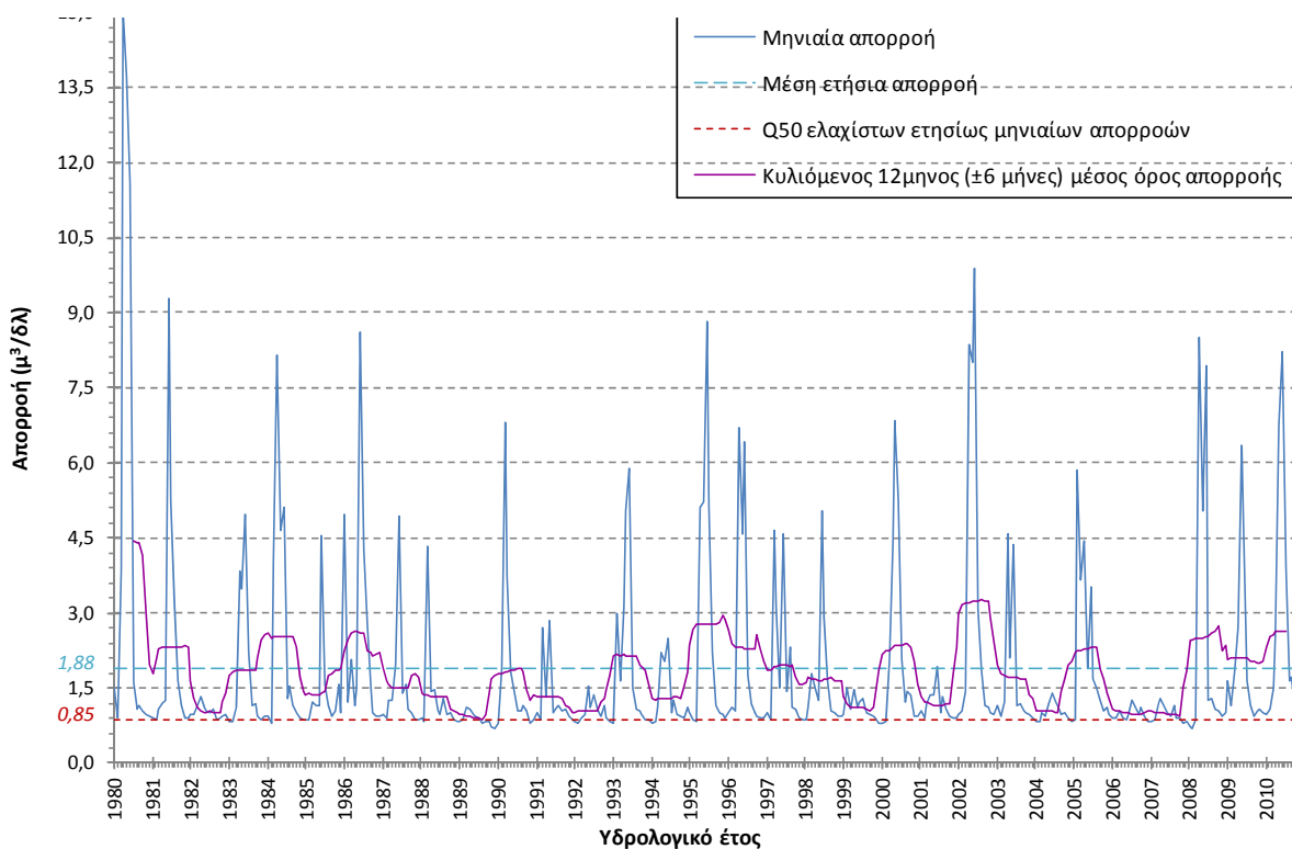
Σχήμα 4-10. Χρονοσειρά απορροής, μέση ετήσια απορροή, κυλιόμενος μέσος όρος και Q 50 ελαχίστων για την περιοχή της εκβολής του π. Τάνου (Σημείο 3_621_0)
