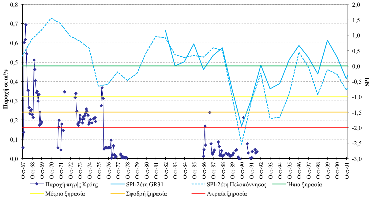
Σχήμα V -8. Συσχέτιση SPI και όρια κατάταξής του με τη χρονοσειρά παροχής της πηγής Κρόης
