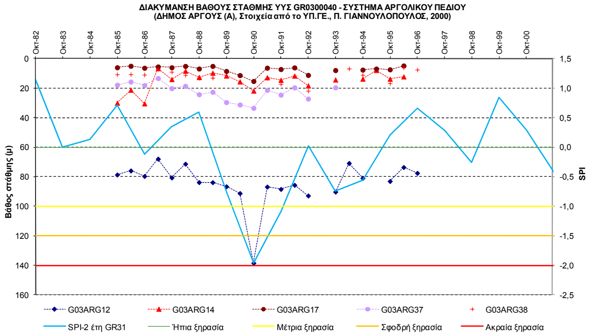
Σχήμα 5-29. Συσχέτιση SPI και όρια κατάταξής του με τη χρονοσειρά στάθμης νερού γεώτρησης στον Δήμο Άργους του ΥΥΣ GR0300040
