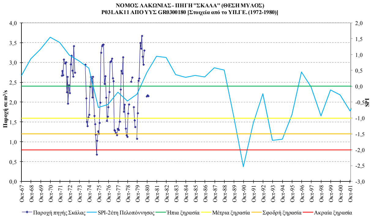
Σχήμα V -11. Συσχέτιση SPI και όρια κατάταξής του με τη χρονοσειρά παροχής της πηγής Σκάλας (Θέση Μύλος)
