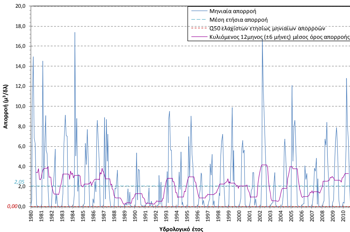
Σχήμα 4-11. Χρονοσειρά απορροής, μέση ετήσια απορροή, κυλιόμενος μέσος όρος και Q 50 ελαχίστων για την περιοχή της εκβολής του π.Πλατύ (Σημείο 3_681_0)
