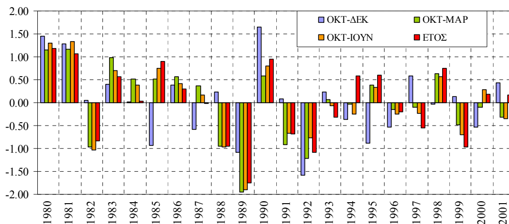
Σχήμα 5-8. Εκτίμηση δείκτη ξηρασίας διαχειριστικής ενότητας Οροπεδίου Τρίπολης, για χρονικές κλίμακες από τρίμηνη έως ετήσια.
