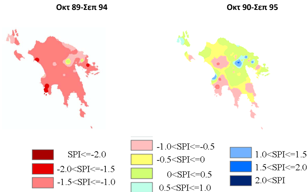
Σχήμα IV -5. Χωρική κατανομή δείκτη ξηρασίας μέσου δείκτη ξηρασίας πέντε ετών για την περίοδο 1988-1995.
