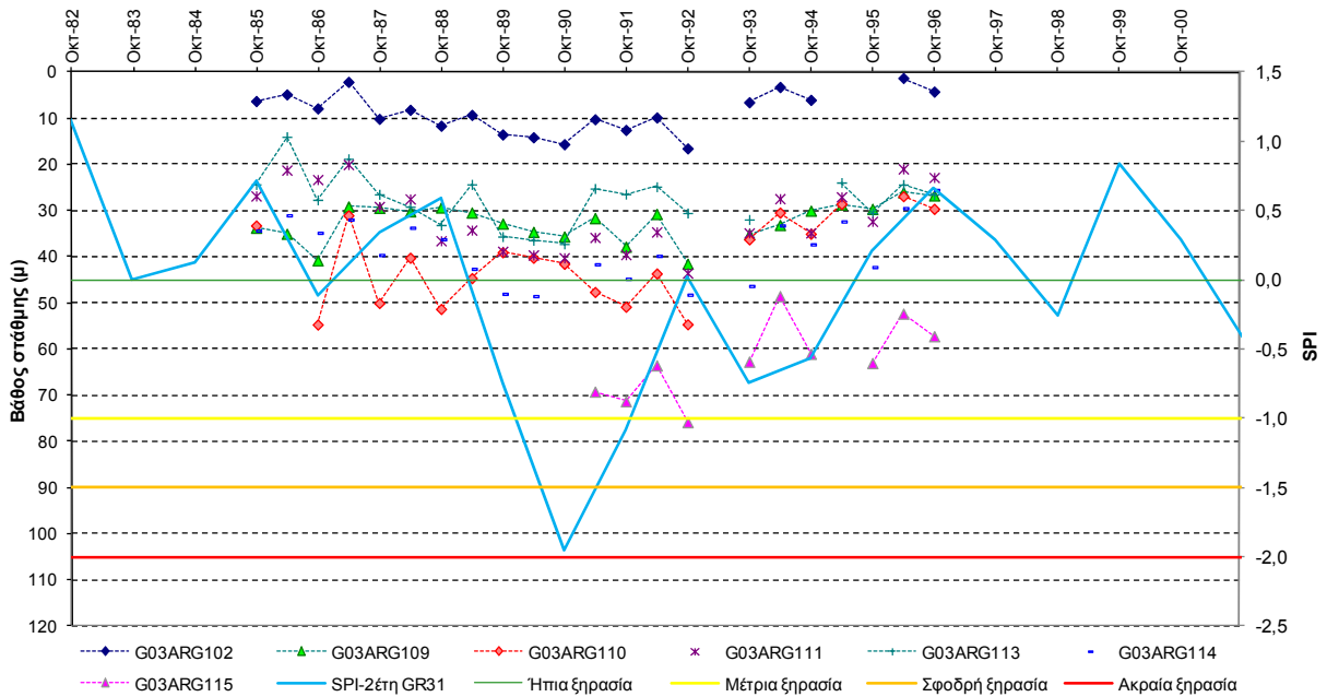
Σχήμα VI -23. Συσχέτιση SPI και όρια κατάταξής του με τη χρονοσειρά στάθμης νερού γεώτρησης στον Δήμο Νέας Τίρυνθας του ΥΥΣ GR0300040
