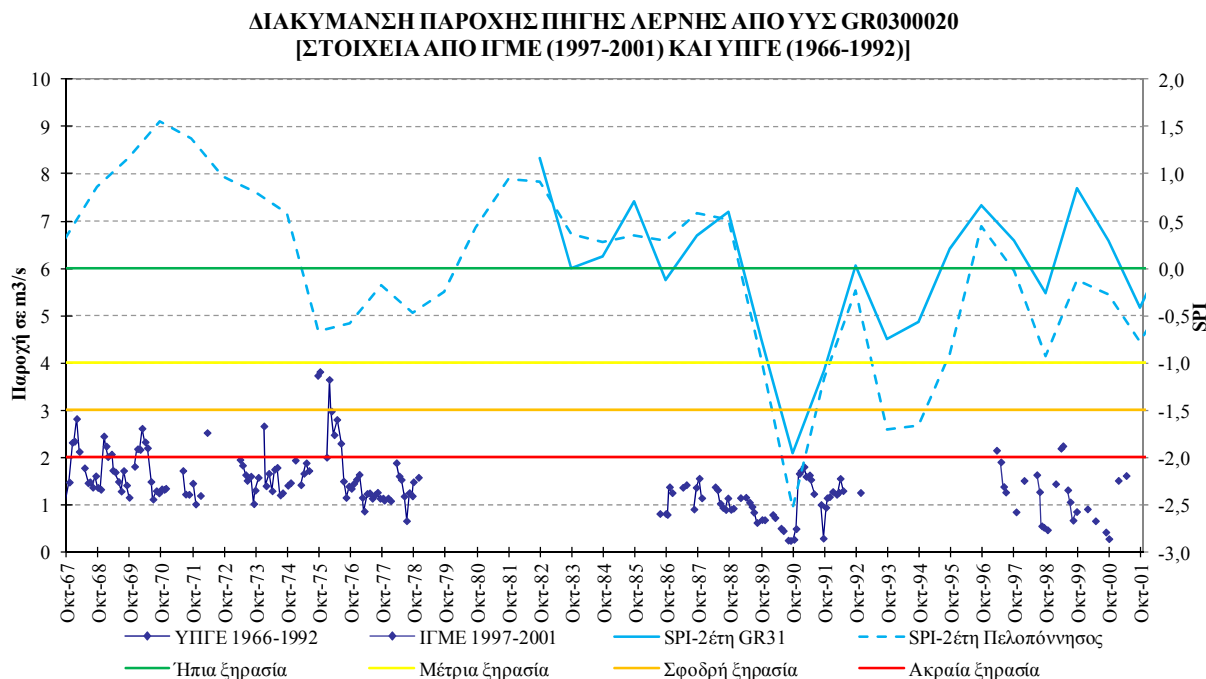
Σχήμα 5-28. Συσχέτιση SPI και όρια κατάταξής του με τη χρονοσειρά παροχής της πηγής Λέρνης
