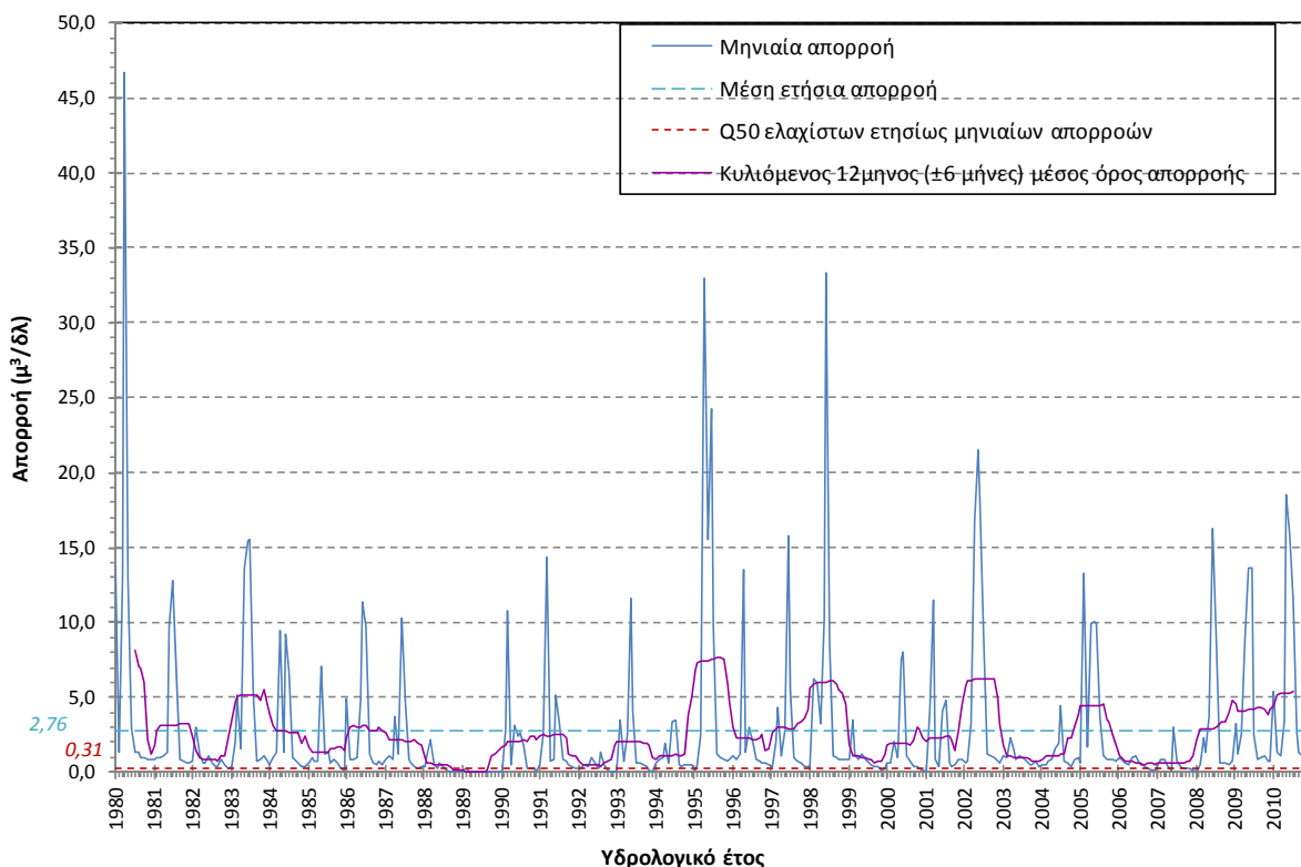
Σχήμα 4-9. Χρονοσειρά απορροής, μέση ετήσια απορροή, κυλιόμενος μέσος όρος και Q 50 ελαχίστων για την περιοχή της εκβολής του π. Ίναχου (Σημείο 3_601_0)
