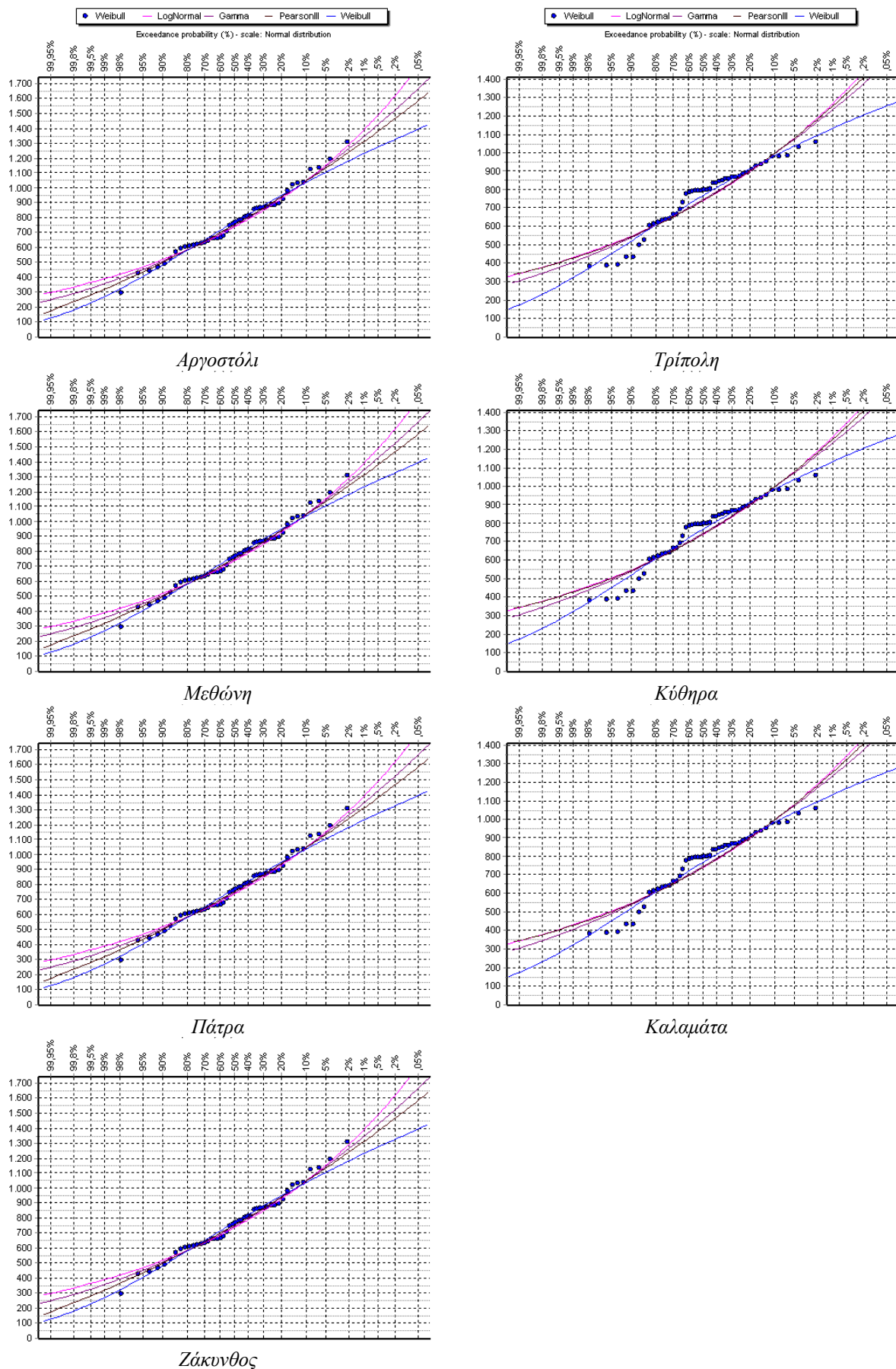
Σχήμα 5-4. Προσαρμογή θεωρητικών κατανομών στα ετήσια ύψη βροχής (σταθμοί ΕΜΥ).
