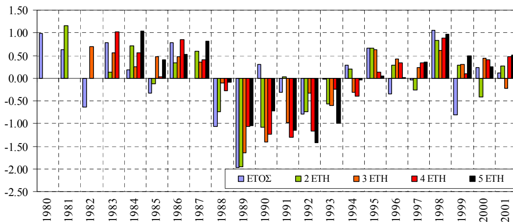
Σχήμα 5-11. Εκτίμηση δείκτη ξηρασίας διαχειριστικής ενότητας Ρεμάτων Αργολικού Κόλπου, για χρονικές κλίμακες από ετήσια έως πενταετή.
