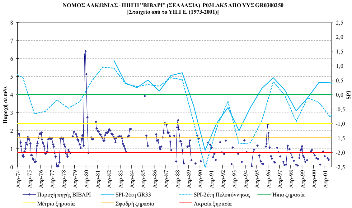
Σχήμα V -12. Συσχέτιση SPI και όρια κατάταξής του με τη χρονοσειρά παροχής της πηγής Βιβάρι (Σελλάσια)
