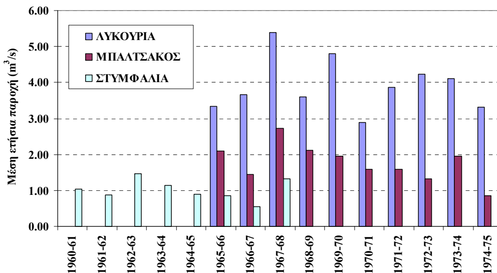
Σχήμα 4-12. Μέση ετήσια παροχή πηγών Λυκουριάς (Λάδωνα), Μπαλτσακού (Παναγίτσα) και Στυμφαλίας, για τα υδρολογικά έτη 1960-61 έως 1974-75.
