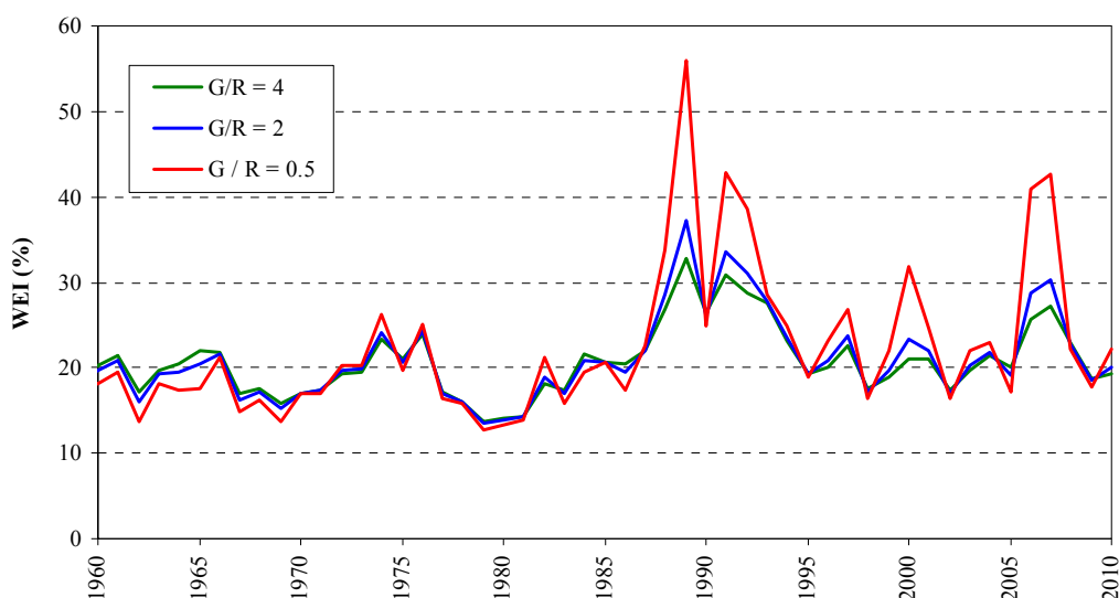
Σχήμα 7-18. Χρονική εξέλιξη του WEI για διάφορες σχέσεις αναλογίας μεταξύ των ετήσιων υπογείων αποθεμάτων προς την ετήσια απορροή.
