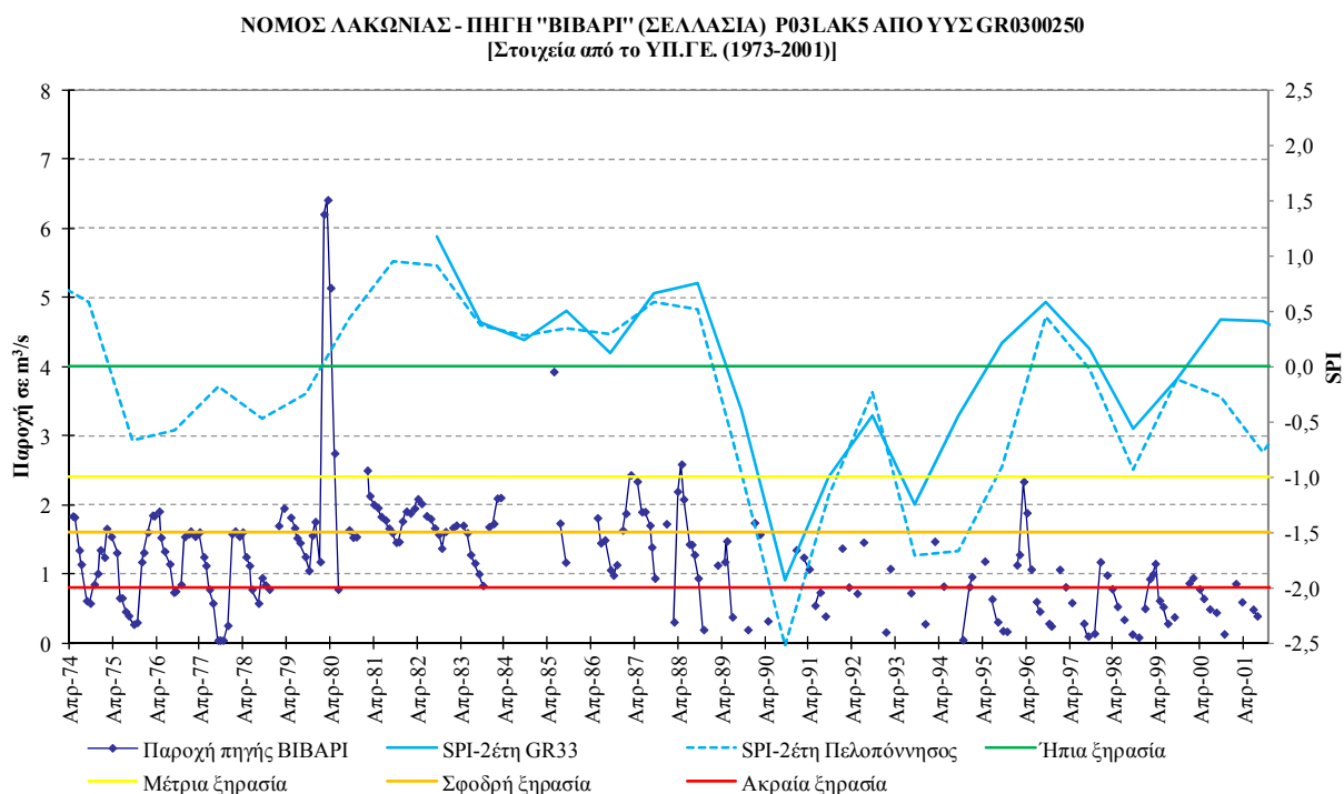
Σχήμα 5-27. Συσχέτιση SPI και όρια κατάταξής του με τη χρονοσειρά παροχής της πηγής Βιβάρι (Σελλασία)
