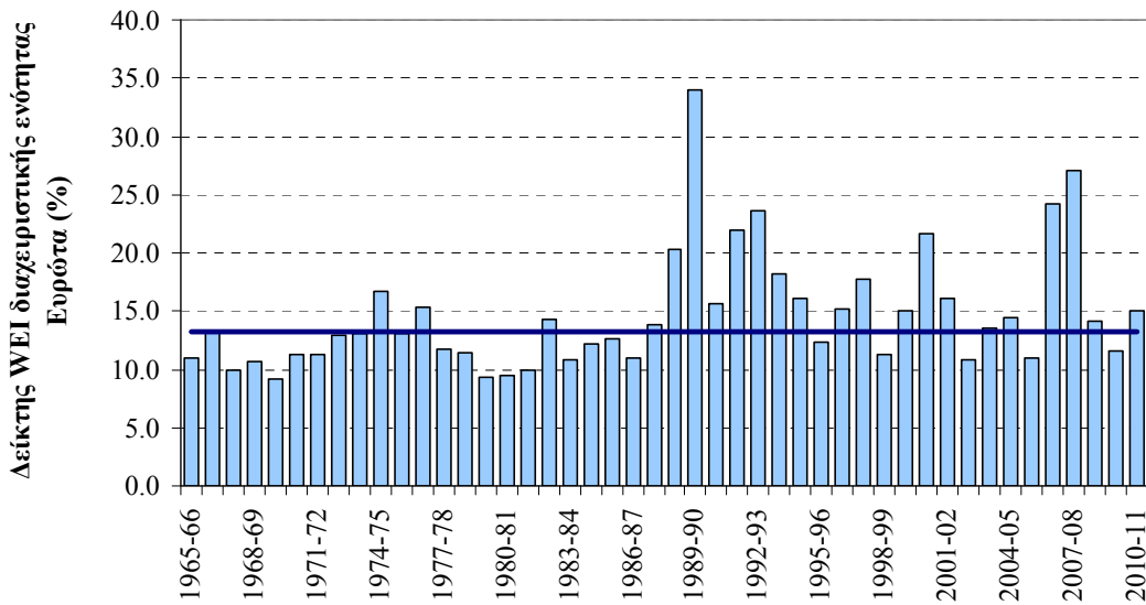
Σχήμα 7-25. Ετήσια μεταβολή του δείκτη WEI, στη ΛΑΠ 33 (με συνεχή γραμμή απεικονίζεται ο υπερετήσιος δείκτης που υπολογίστηκε με βάση τα μεγέθη του μέσου ετήσιου υδατικού ισοζυγίου της ΛΑΠ).
