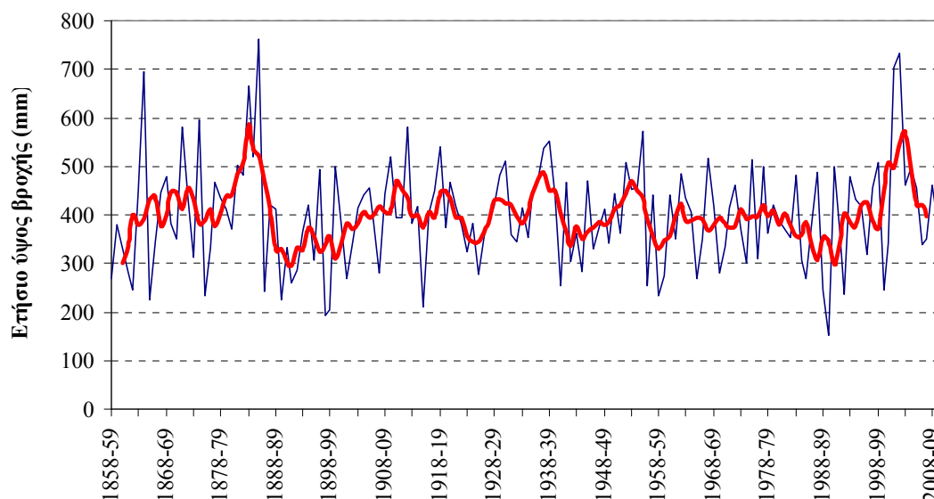
Σχήμα 5-2. Ετήσιο ύψος βροχής Αθηνών (Θησείο) και κινούμενοι μέσοι όροι πέντε ετών. Πίνακας 5-1. Στατιστικά χαρακτηριστικά βροχόπτωσης Εθνικού Αστεροσκοπείου Αθηνών (Θησείο) σε διάφορες χρονικές κλίμακες, για τα υδρολογικά έτη 1857-58 έως 2010-11.
