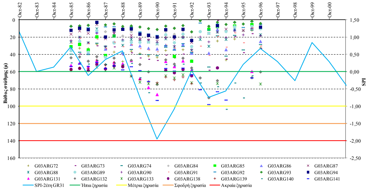
Σχήμα VI -20. Συσχέτιση SPI και όρια κατάταξής του με τη χρονοσειρά στάθμης νερού γεώτρησης στον Δήμο Άργους (Γ) του ΥΥΣ GR0300040
