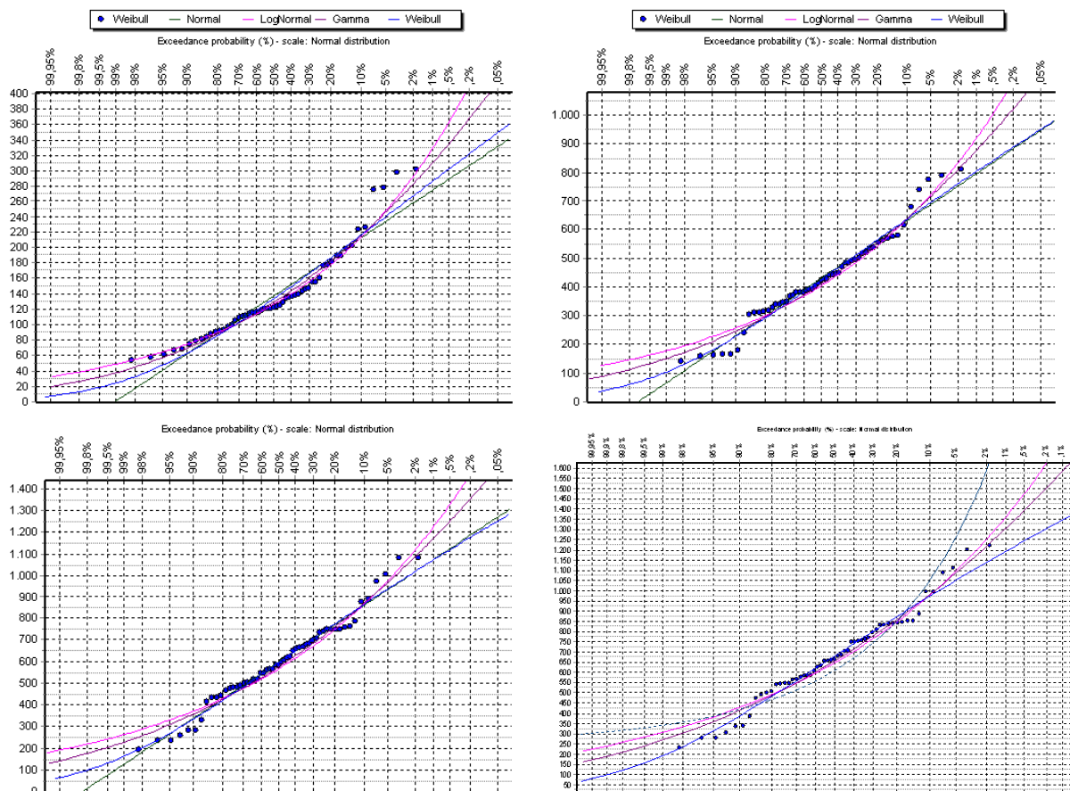
Σχήμα 5-5. Προσαρμογή θεωρητικών κατανομών στα δείγματα μηνιαίων υψών απορροής του Λάδωνα, για χρονικές κλίμακες τριών μηνών (πάνω αριστερά), έξι μηνών (πάνω δεξιά), εννέα μηνών (κάτω αριστερά), και έτους (κάτω δεξιά).
