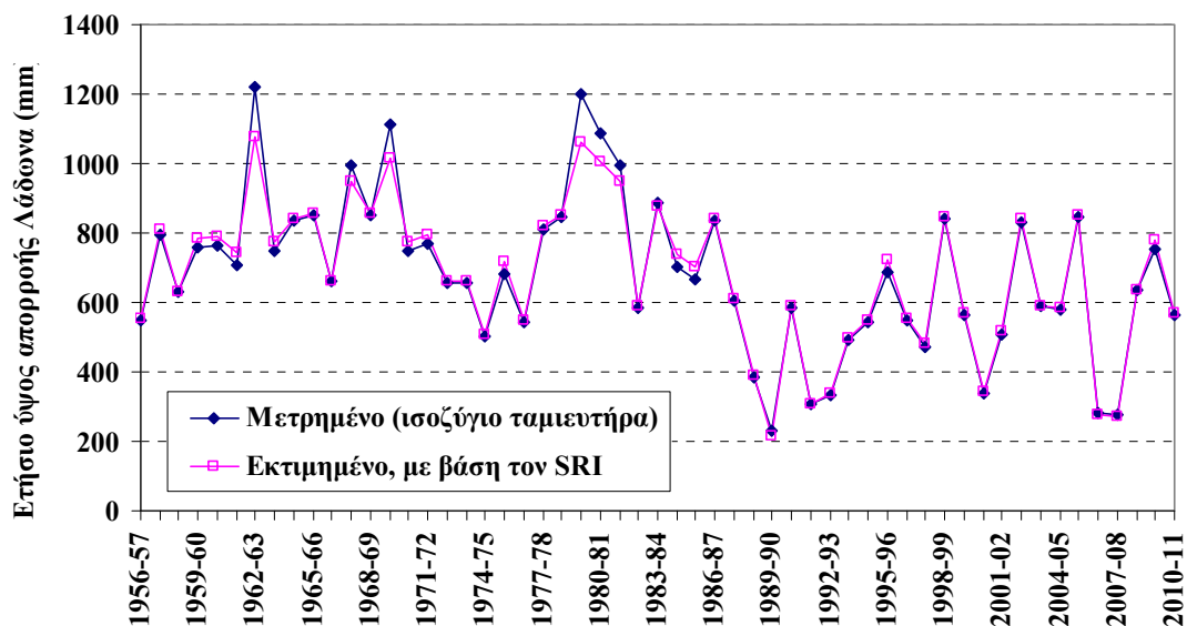
Σχήμα 7-16. Σύγκριση ετήσιων χρονοσειρών απορροής Λάδωνα, μετρημένων (υπολογισμός από το υδατικό ισοζύγιο του ταμειυτήρα) και εκτιμημένων, με βάση τη σχέση (7.7).
