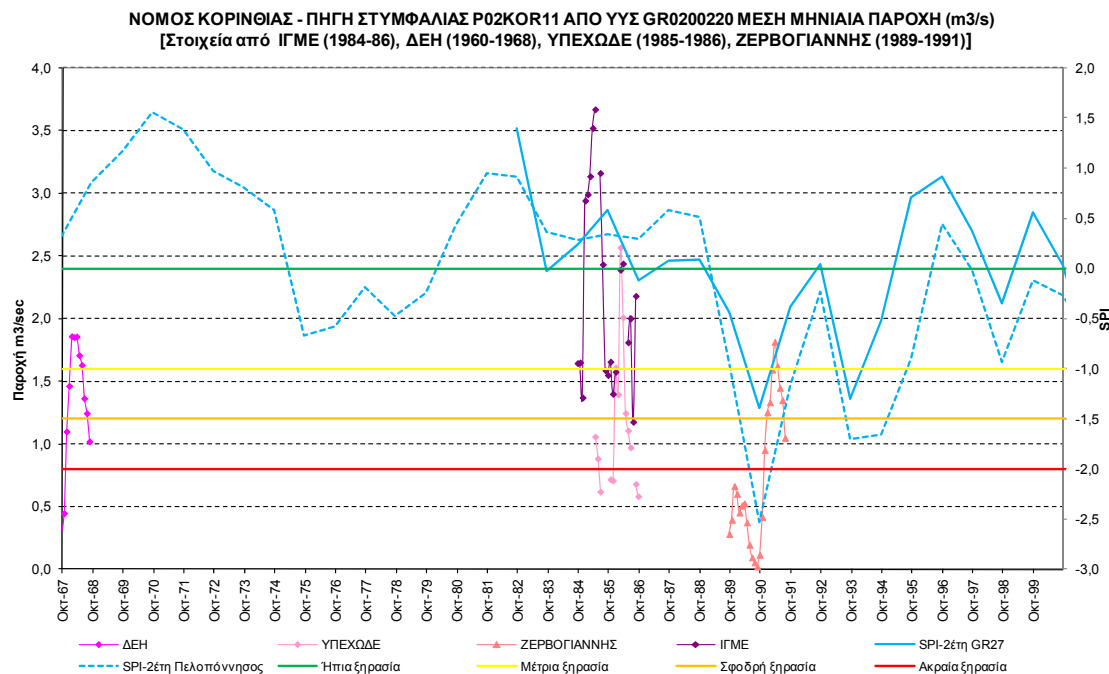
Σχήμα V-6. Συσχέτιση SPI και όρια κατάταξής του με τη χρονοσειρά παροχής της πηγής Στυμφαλίας
