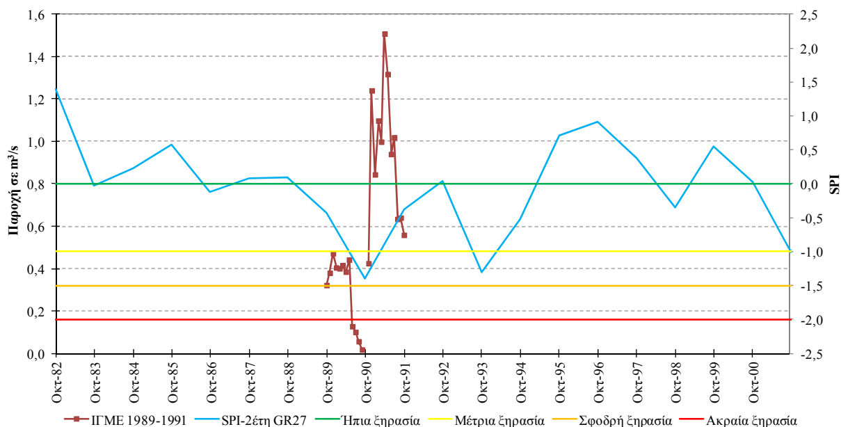
Σχήμα V-11. Συσχέτιση SPI και όρια κατάταξής του με τη χρονοσειρά παροχής της πηγής Στυμφαλίας στη θέση Πόρτα, στη γέφυρα Βοχαϊκού Αύλακα
