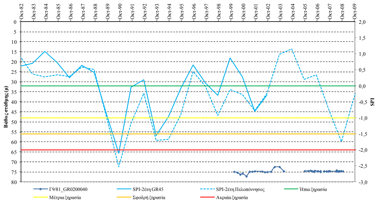
Σχήμα VI-16. Συσχέτιση SPI και όρια κατάταξής του με τη χρονοσειρά στάθμης νερού γεώτρησης στο σημείο Γ9/81 του ΥΥΣ GR0200040
