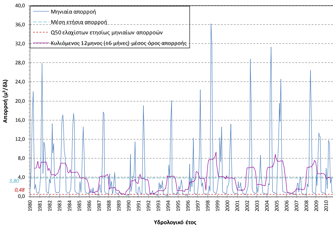
Σχήμα 4-9. Χρονοσειρά απορροής, μέση ετήσια απορροή, κυλιόμενος μέσος όρος και Q_{50} ελαχίστων για την περιοχή της εκβολής του π. Πείρου (Σημείο 2_201_0)
