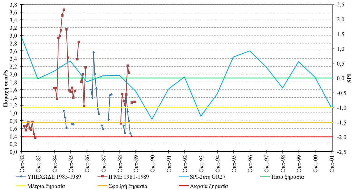
Σχήμα V-9. Συσχέτιση SPI και όρια κατάταξής του με τη χρονοσειρά παροχής πηγής (2) Στη Στυμφαλία
