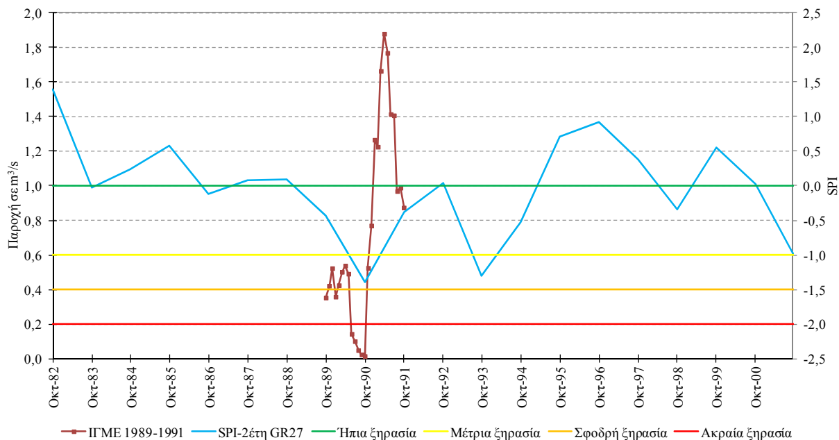
Σχήμα V-10. Συσχέτιση SPI και όρια κατάταξής του με τη χρονοσειρά παροχής της πηγής Στυμφαλίας στη θέση Πασσαλοσανίδα Κορινθίας
