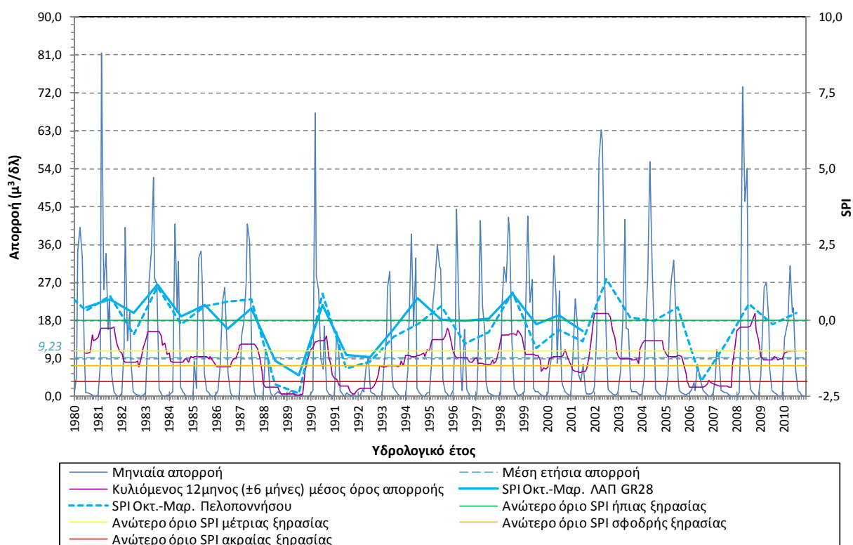
Σχήμα 5-23. Συσχέτιση SPI και όρια κατάταξης του με τη χρονοσειρά απορροής του μοντέλου Sacramento για την περιοχή της εκβολής του π. Πηνειού (Σημείο 2_101_0)
