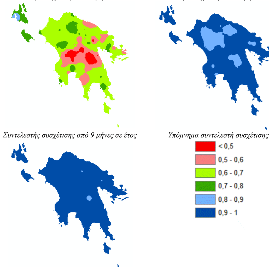
Σχήμα 9-1. Επιφανειακή ολοκλήρωση συντελεστών συσχέτισης του δείκτη ξηρασίας μεταξύ των τιμών τριμήνου, εξαμήνου και εννιαμήνου και της αντίστοιχης ετήσιας τιμής.
