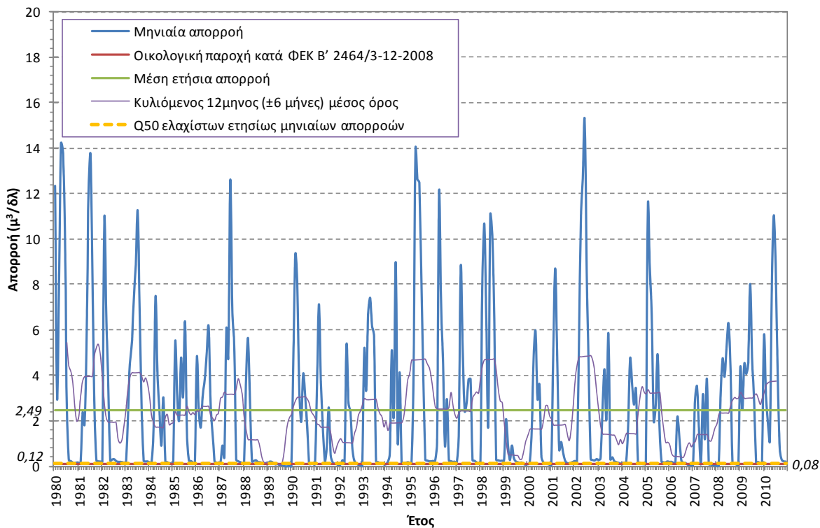
Σχήμα 8-2. Γράφημα απορροών στην εκβολή του π. Ασωπού (GR27)
