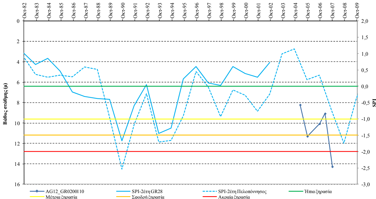
Σχήμα VI-15. Συσχέτιση SPI και όρια κατάταξής του με τη χρονοσειρά στάθμης νερού γεώτρησης στο σημείο AG12 του ΥΥΣ GR0200110
