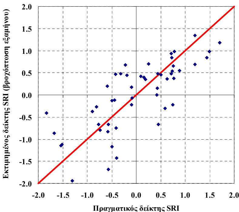
Σχήμα 10-7. Διάγραμμα διασποράς εκτιμημένου, με βάση την αθροιστική βροχόπτωση εξαμήνου (του σταθμού Τρίτολης), και πραγματικού δείκτη SRI μέσης ετήσιας απορροής στη λεκάνη η του Λάδωνα.
