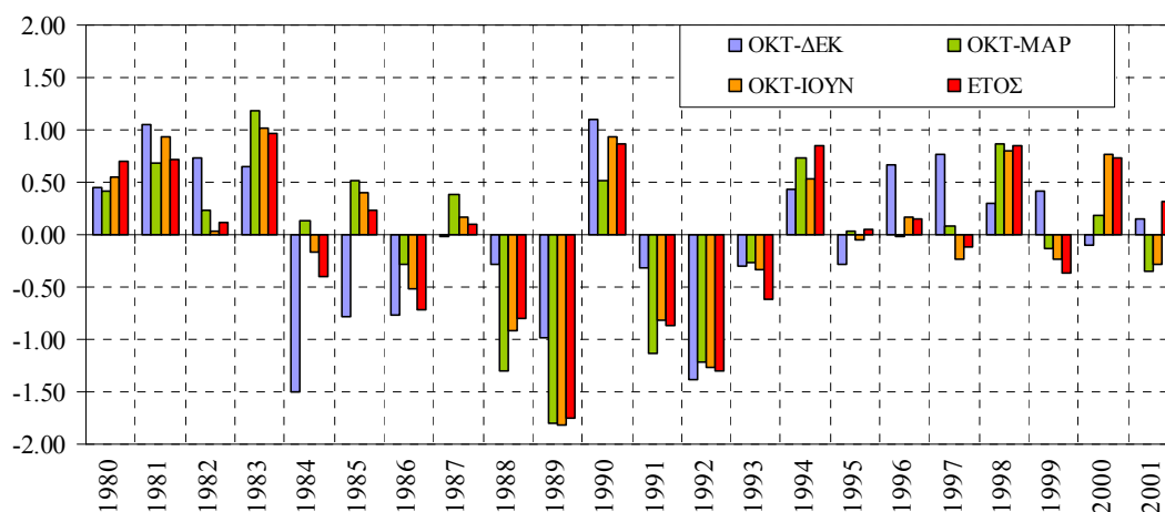
Σχήμα 5-10. Εκτίμηση δείκτη ξηρασίας διαχειριστικής ενότητας Πείρου-Βέργα-Πηνειού, για χρονικές κλίμακες από τρίμηνη έως ετήσια.
