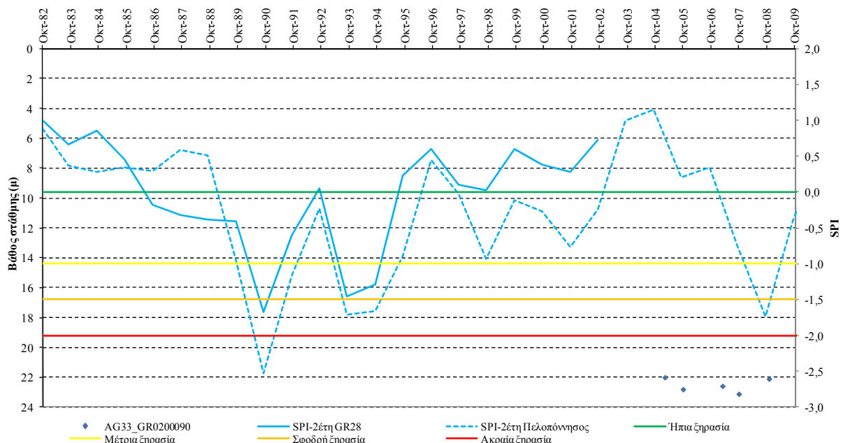
Σχήμα VI-14. Συσχέτιση SPI και όρια κατάταξής του με τη χρονοσειρά στάθμης νερού γεώτρησης στο σημείο AG33 του ΥΥΣ GR0200090
