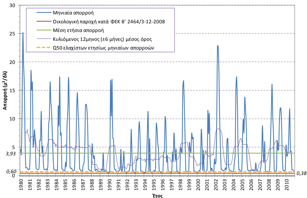
Σχήμα 8-3. Γράφημα απορροών στην εκβολή του π. Βουραϊκού (GR27)
