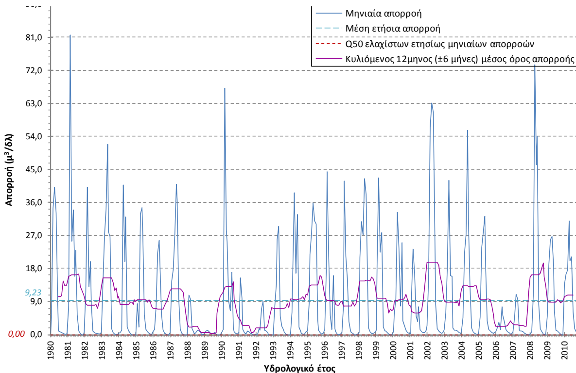
Σχήμα 4-8. Χρονοσειρά απορροής, μέση ετήσια απορροή, κυλιόμενος μέσος όρος και Q_{50} ελαχίστων για την περιοχή της εκβολής του π. Πηνειού (Σημείο 2_101_0)
