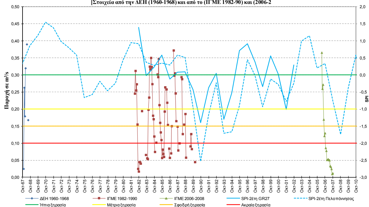
Σχήμα 5-29. Συσχέτιση SPI και όρια κατάταξής του με τη χρονοσειρά παροχής της πηγής Συβίστα (κεφαλόβρυσο)
