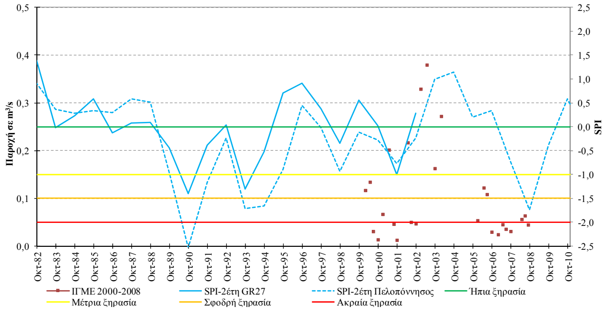
Σχήμα V-8. Συσχέτιση SPI και όρια κατάταξής του με τη χρονοσειρά παροχής της πηγής Κ/Π21 Στυμφαλίας
