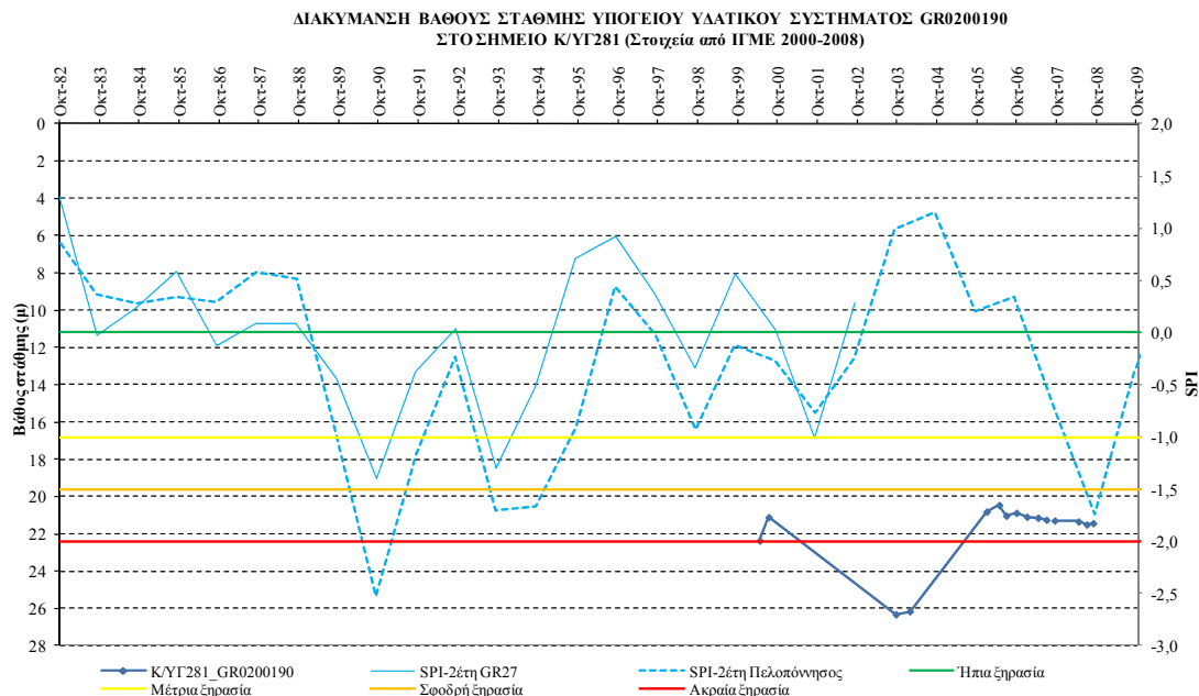
Σχήμα VI-12. Συσχέτιση SPI και όρια κατάταξής του με τη χρονοσειρά στάθμης νερού γεώτρησης στο σημείο Κ/ΥΓ281 του ΥΥΣ GR0200190
