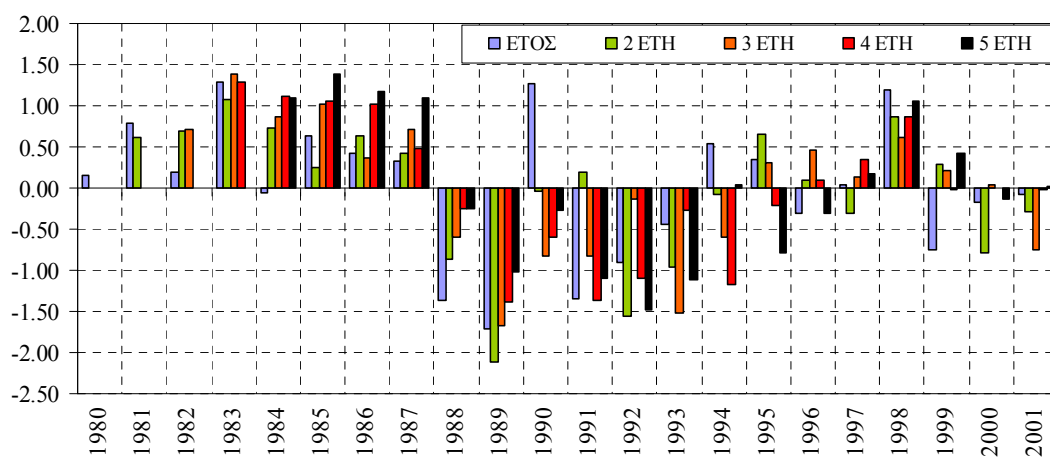
Σχήμα 5-13. Εκτίμηση δείκτη ξηρασίας διαχειριστικής ενότητας Κεφαλονιάς-Ιθάκης-Ζακύνθου, για χρονικές κλίμακες από ετήσια έως πενταετή.
