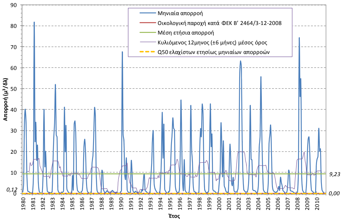
Σχήμα 8-4. Γράφημα απορροών στην εκβολή του π. Πηνειού (GR28)
