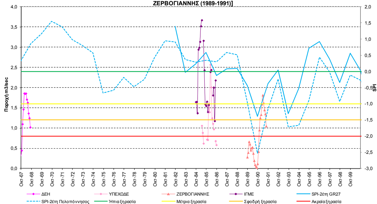
Σχήμα 5-28. Συσχέτιση SPI και όρια κατάταξής του με τη χρονοσειρά παροχής της πηγής Στυμφαλίας
