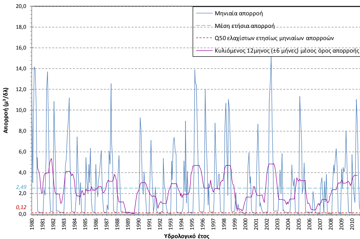
Σχήμα 4-11. Χρονοσειρά απορροής, μέση ετήσια απορροή, κυλιόμενος μέσος όρος και Q 50 ελαχίστων για την περιοχή της εκβολής του π. Ασωπού (Σημείο 2_611_0)
