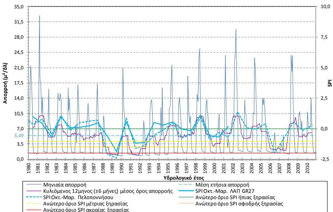
Σχήμα 5-25. Συσχέτιση SPI και όρια κατάταξης του με τη χρονοσειρά απορροής του μοντέλου Sacramento για την περιοχή της εκβολής του π. Σελινούντα (Σημείο 2_601_0)
