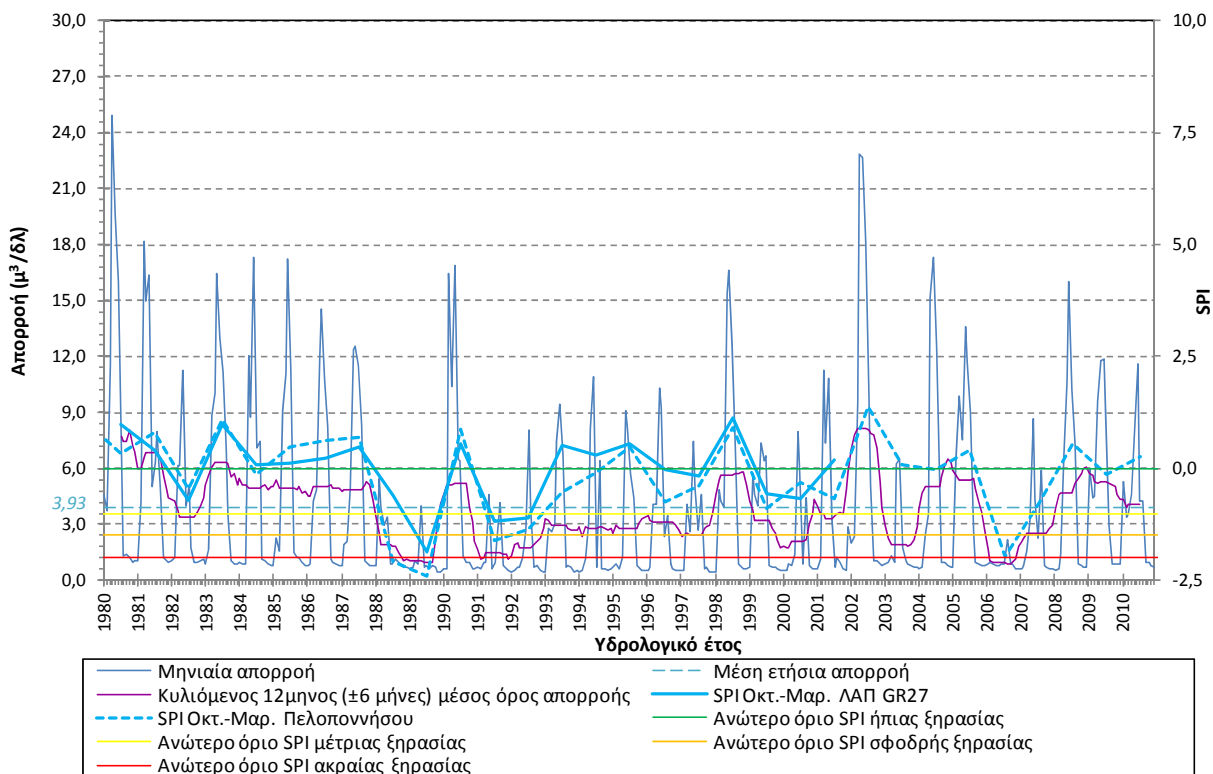
Σχήμα 5-27. Συσχέτιση SPI και όρια κατάταξης του με τη χρονοσειρά απορροής του μοντέλου Sacramento για την περιοχή της εκβολής του π. Βουραϊκού (Σημείο 2_631_0)
