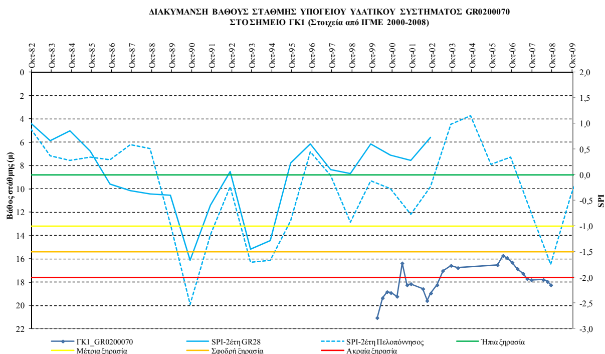
Σχήμα 5-30. Συσχέτιση SPI και όρια κατάταξής του με τη χρονοσειρά στάθμης νερού γεώτρησης στο σημείο ΓΚ1 του ΥΥΣ GR0200070
