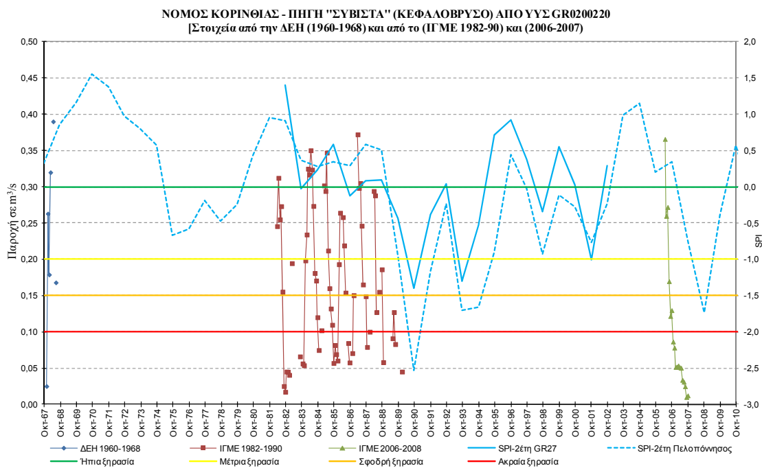
Σχήμα V-7. Συσχέτιση SPI και όρια κατάταξής του με τη χρονοσειρά παροχής της πηγής Συβίστα (Κεφαλόβρυσο)
