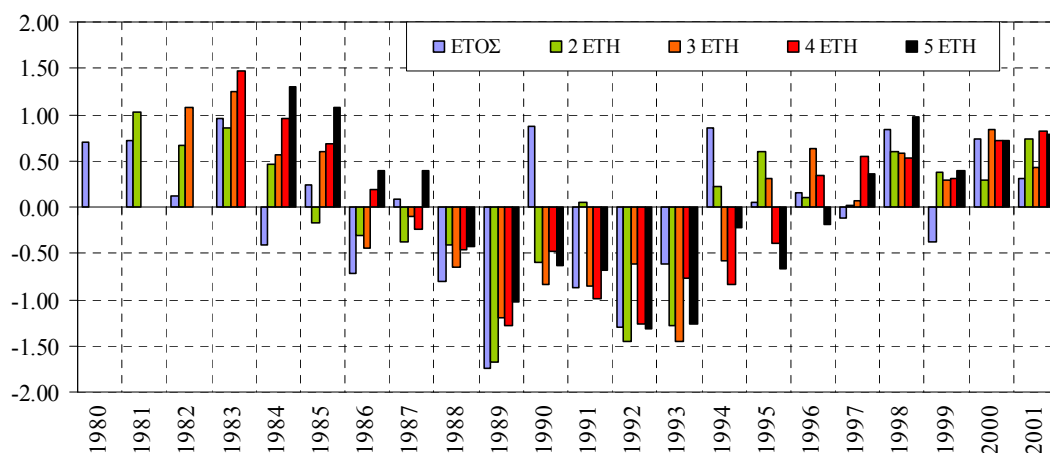
Σχήμα 5-11. Εκτίμηση δείκτη ξηρασίας διαχειριστικής ενότητας Πείρου-Βέργα-Πηνειού, για χρονικές κλίμακες από ετήσια έως πενταετή.
