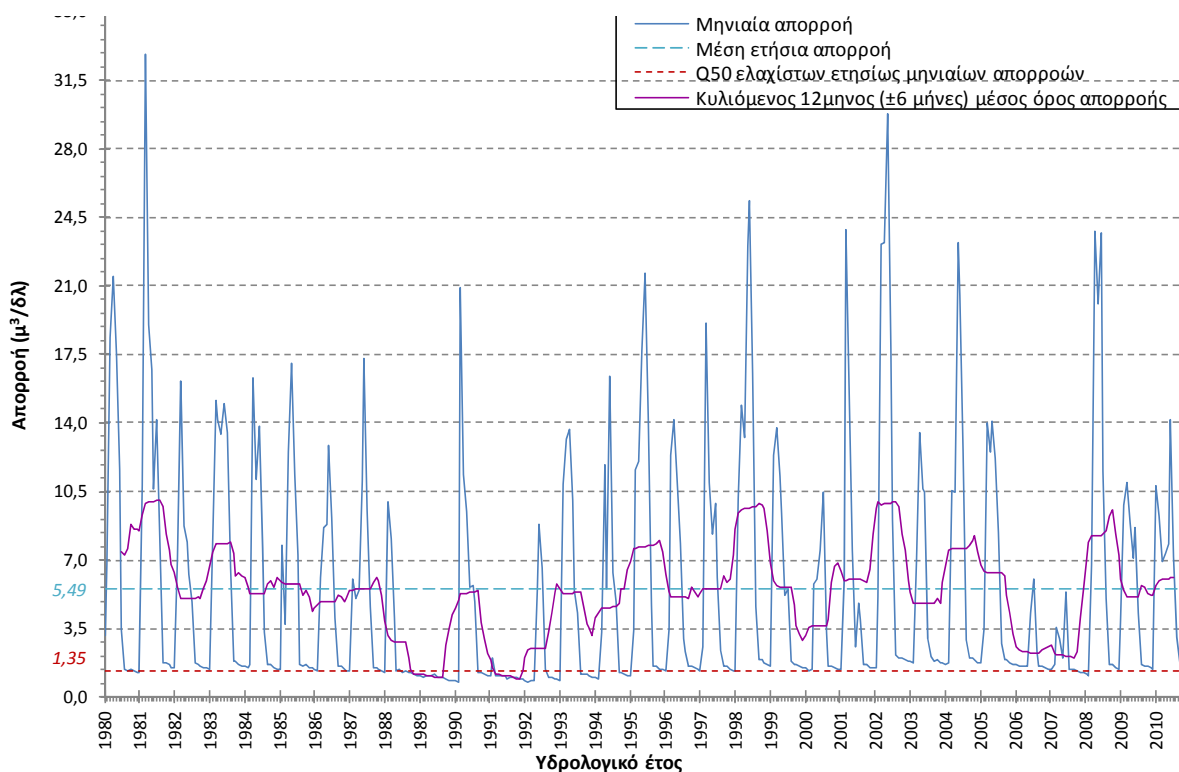
Σχήμα 4-10. Χρονοσειρά απορροής, μέση ετήσια απορροή, κυλιόμενος μέσος όρος και Q 50 ελαχίστων για την περιοχή της εκβολής του π. Σελινούντα (Σημείο 2_601_0)
