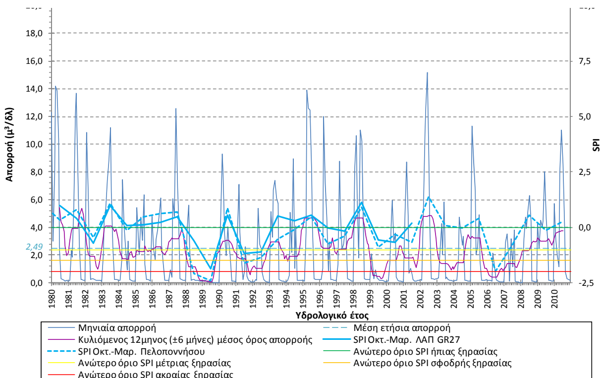
Σχήμα 5-26. Συσχέτιση SPI και όρια κατάταξης του με τη χρονοσειρά απορροής του μοντέλου Sacramento για την περιοχή της εκβολής του π. Ασωπού (Σημείο 2_611_0)
