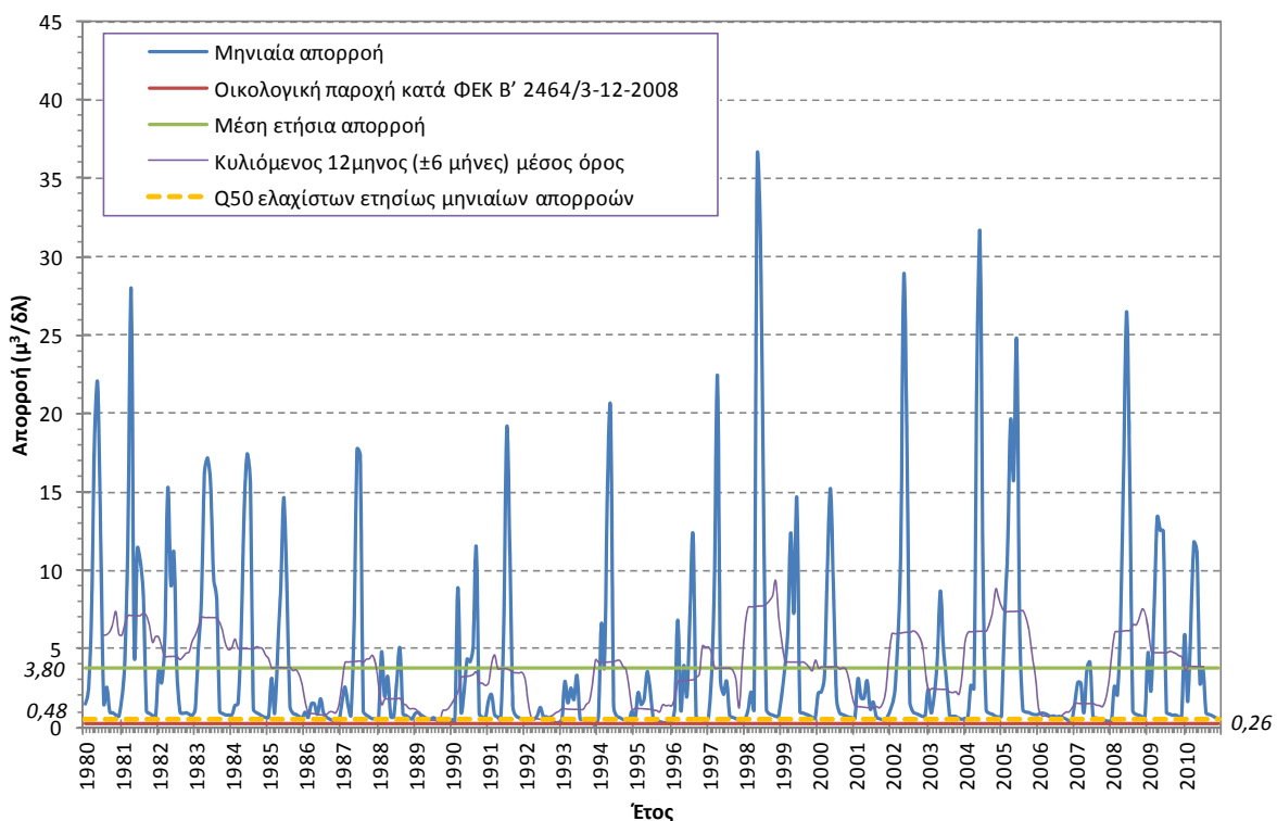
Σχήμα 8-5. Γράφημα απορροών στην εκβολή του π. Πείρου (GR28)
