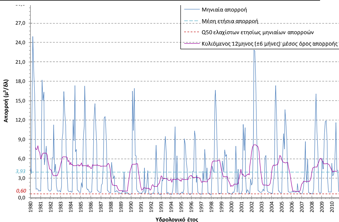
Σχήμα 4-12. Χρονοσειρά απορροής, μέση ετήσια απορροή, κυλιόμενος μέσος όρος και Q_{50} ελαχίστων για την περιοχή της εκβολής του π. Βουραϊκού (Σημείο 2_631_0)
