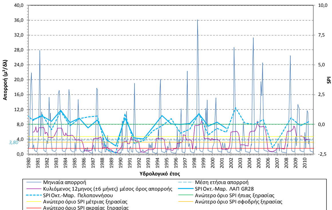
Σχήμα 5-24. Συσχέτιση SPI και όρια κατάταξης του με τη χρονοσειρά απορροής του μοντέλου Sacramento για την περιοχή της εκβολής του π. Πείρου (Σημείο 2_201_0)
