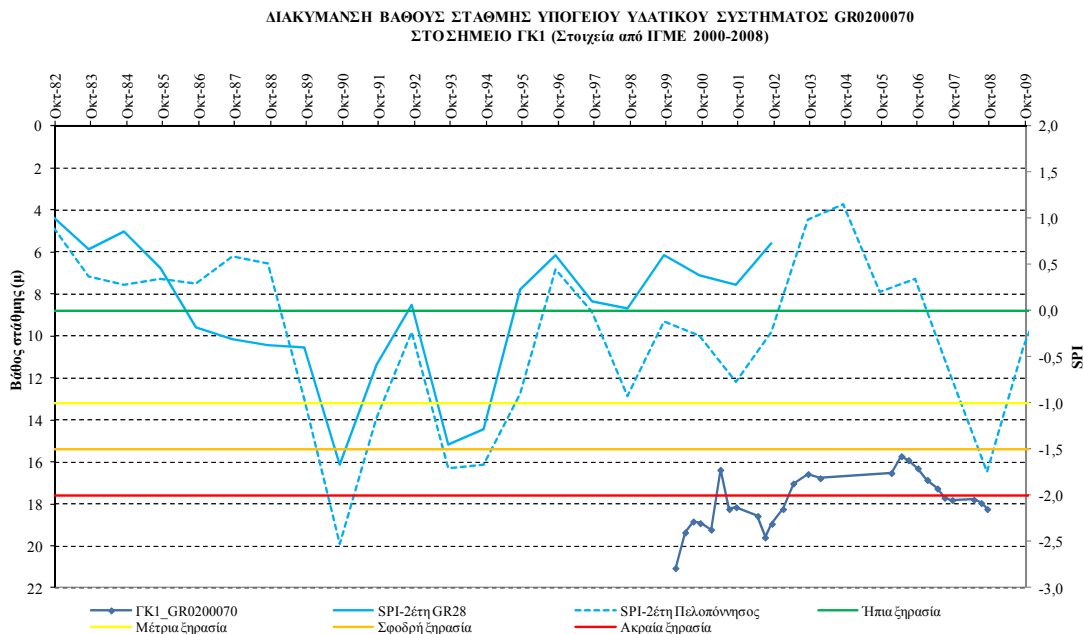
Σχήμα VI-13. Συσχέτιση SPI και όρια κατάταξής του με τη χρονοσειρά στάθμης νερού γεώτρησης στο σημείο ΓΚ1 του ΥΥΣ GR0200070
