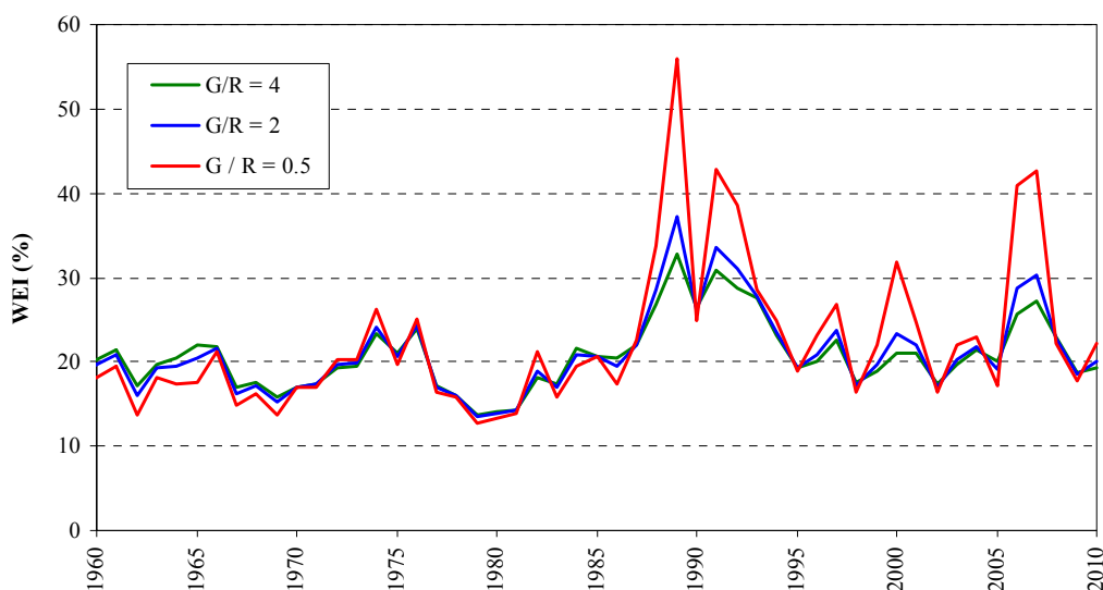
Σχήμα 7-18. Χρονική εξέλιξη του WEI για διάφορες σχέσεις αναλογίας μεταξύ των ετήσιων υπόγειων αποθεμάτων προς την ετήσια απορροή.
